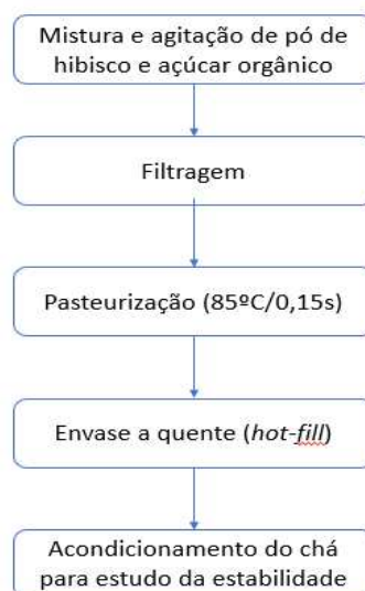
Figura 5. Fluxograma da elaboração do chá de hibisco com açúcar orgânico.
