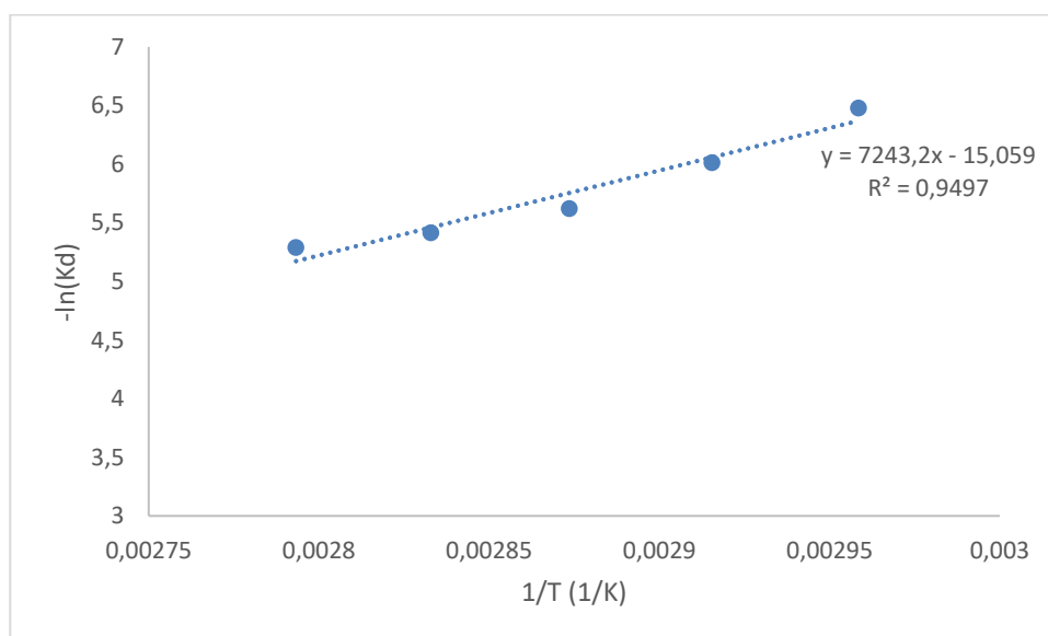
Figura 8. Determinação da energia de ativação ( E_a ) por meio do logaritmo neperiano da constante de degradação térmica pelo inverso da temperatura (K).
