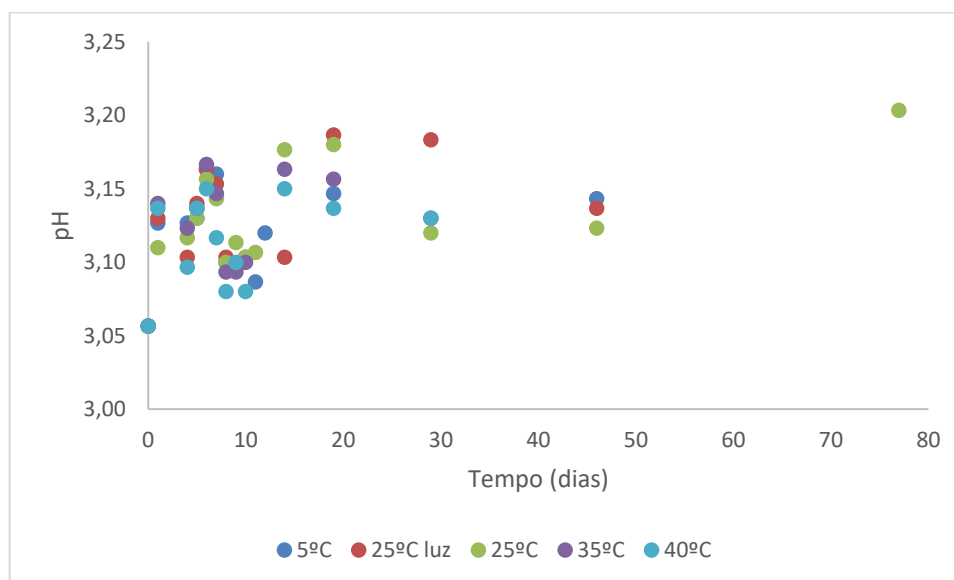
Figura 9. Valores de pH ao longo de 77 dias para as condições de 5°C, 25°C, 25°C (luz), 35°C e 40°C.
