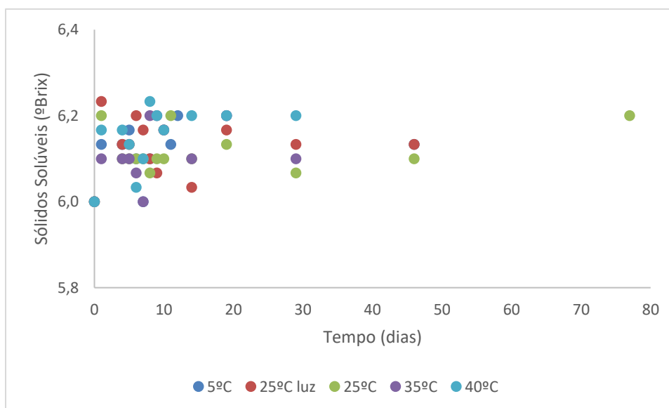
Figura 10. Valores determinados de sólidos solúveis (°Brix) ao longo de 77 dias para o chá de hibisco nas temperaturas de 5°C, 25°C, 25°C (luz), 35°C e 40°C.
