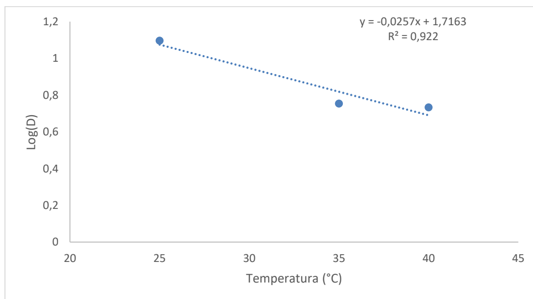
Figura 15. Determinação do valor Z por meio do logaritmo de D pela temperatura (°C).
