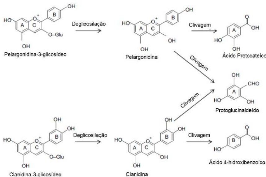
Figura 4. Mecanismo de degradação de antocianinas.
