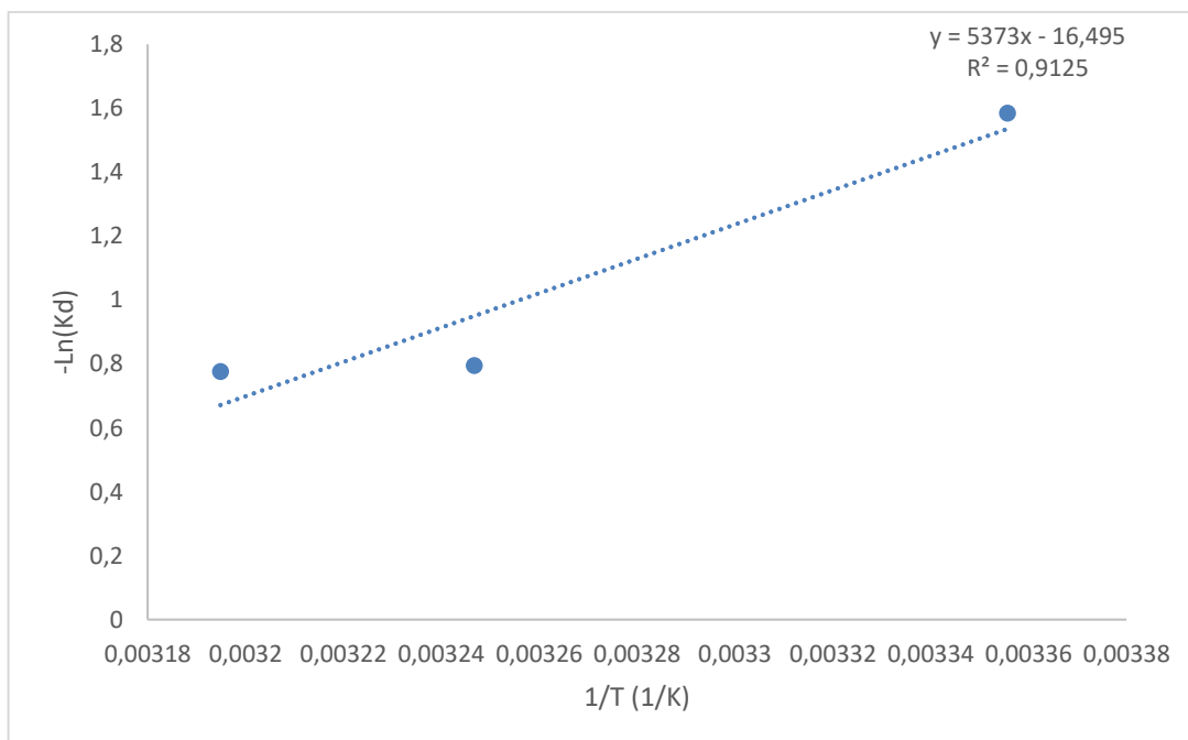
Figura 16. Determinação da energia de ativação ( E_a ) por meio do logaritmo neperiano da constante de degradação térmica pelo inverso da temperatura (K).
