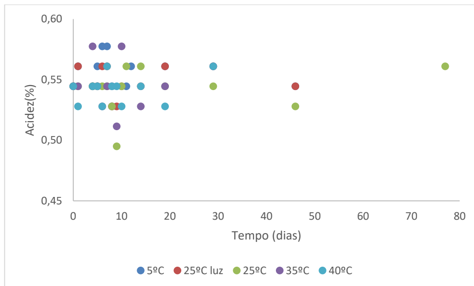
Figura 11. Valores de acidez titulável total ao longo de 77 dias para as condições de 5°C, 25°C, 25°C (luz), 35°C e 40°C.
