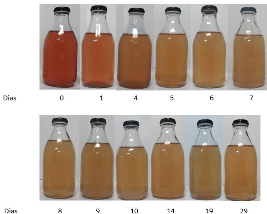
Figura 21. Amostras de chá de hibisco com açúcar orgânico ao longo do tempo de armazenamento a 40°C.
