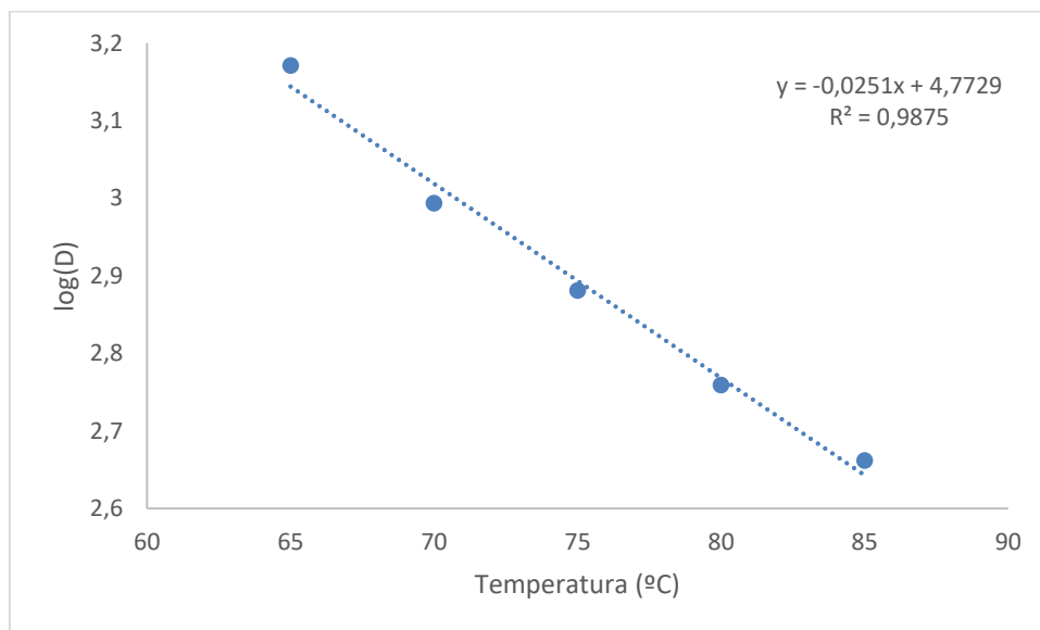
Figura 7. Determinação do valor Z por meio do logaritmo de D pela temperatura (°C).
