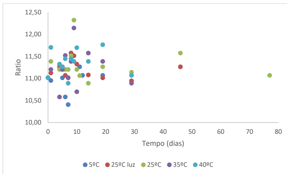
Figura 12. Valores de ratio ao longo de 77 dias para as condições de 5°C, 25°C, 25°C (luz), 35°C e 40°C.
