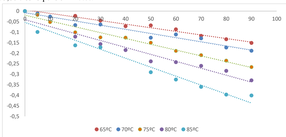
Figura 6. Degradação das antocianinas do extrato de hibisco durante aquecimento a 65,70,75,80 e 85°C por 90 minutos.
