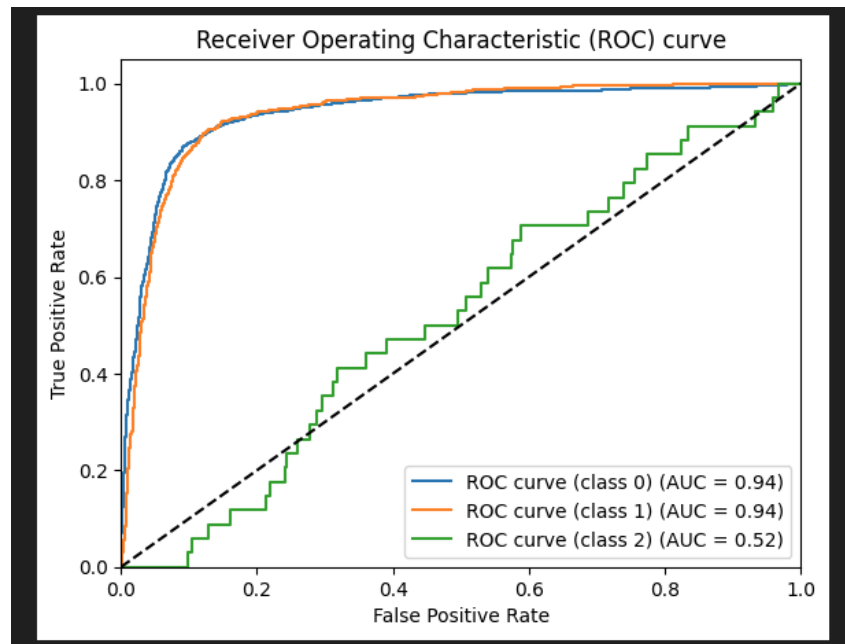
Figura 5.6 – Curva ROC do teste
