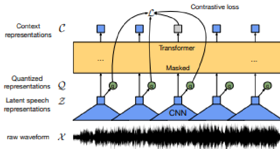
Figura 4.1 – Estrutura do modelo Wav2Vec2 (BAEVSKI et al. , 2020)
