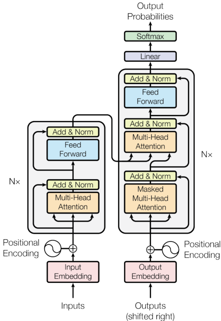
Figura 3.2 – Estrutura completa de um transformer (VASWANI et al. , 2023)
