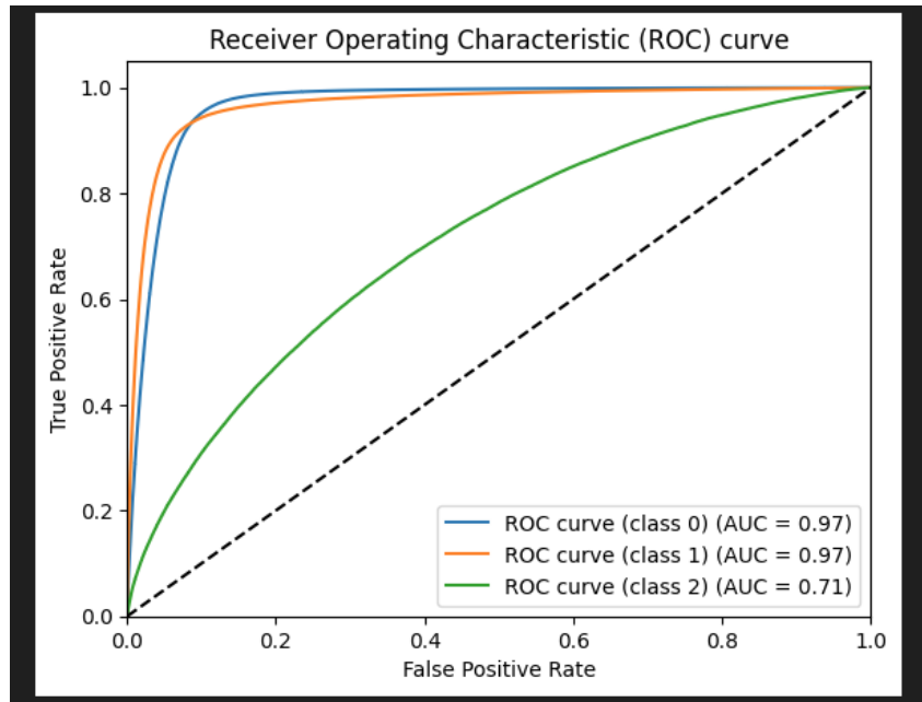
Figura 5.4 – Curva ROC do treinamento
