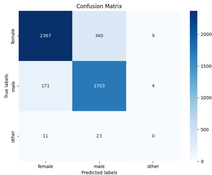
Figura 5.3 – Matriz de Confusão do conjunto de teste
