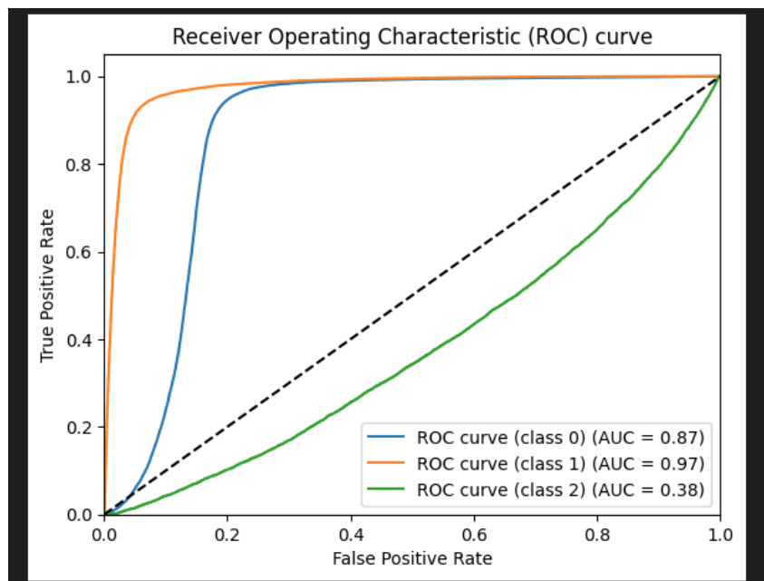
Figura 5.5 – Curva ROC da validação
