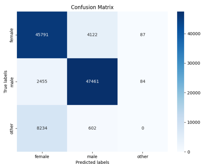
Figura 5.2 – Matriz de Confusão do conjunto de validação
