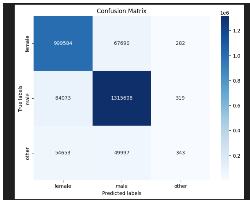
Figura 5.1 – Matriz de Confusão das 7 épocas de treinamento
