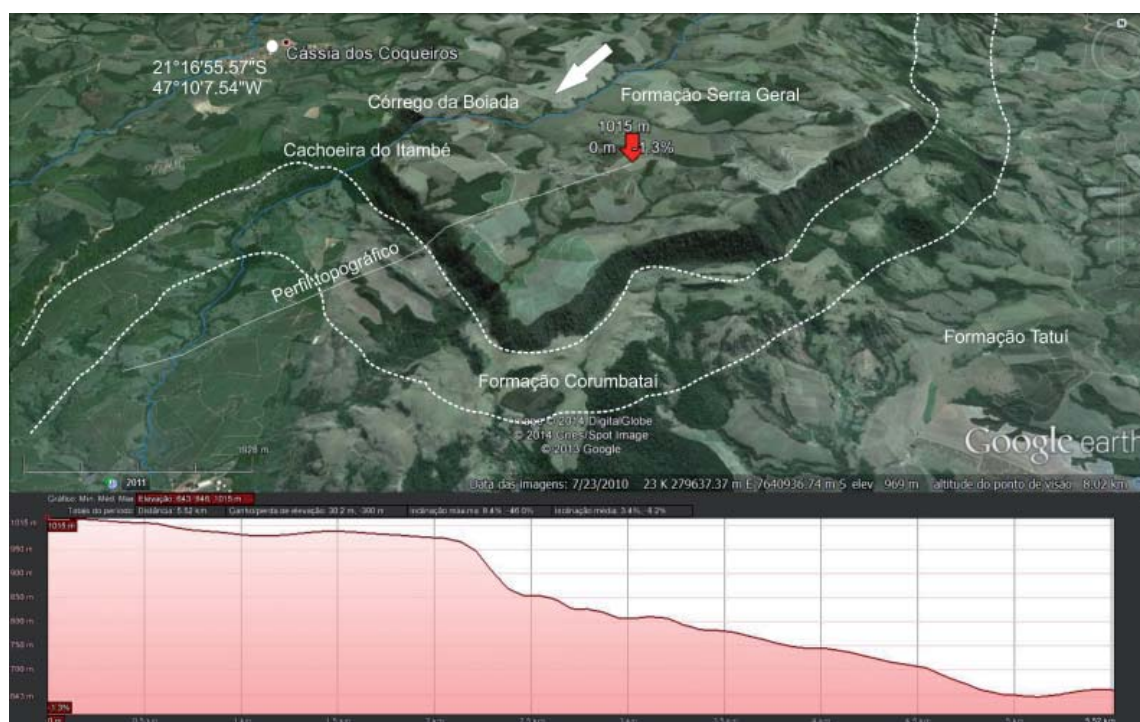
Figura 11 - Área da cachoeira do Itambé no Córrego da Boiada, em detalhe o ressaltamento entre as formações permianas e carboníferas (abaixo de 850 m) e a Formação Serra Geral (1000 m). A seta branca indica a direção do fluxo da drenagem.
