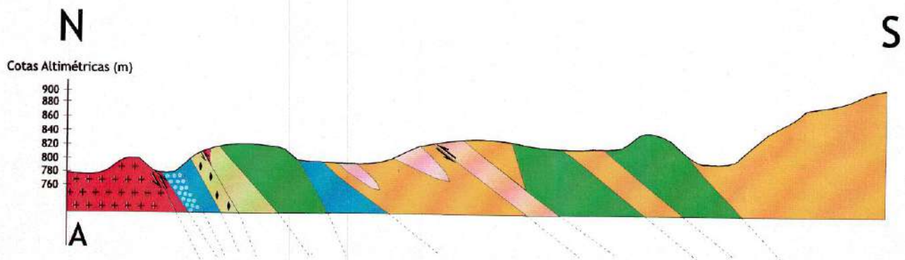
Perfil A - A'
