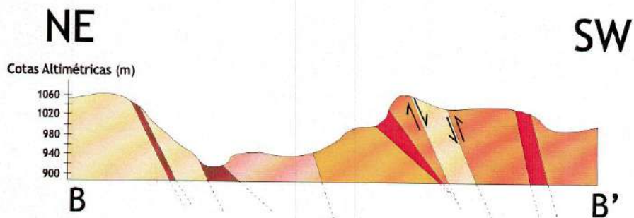
Perfil B - B'
