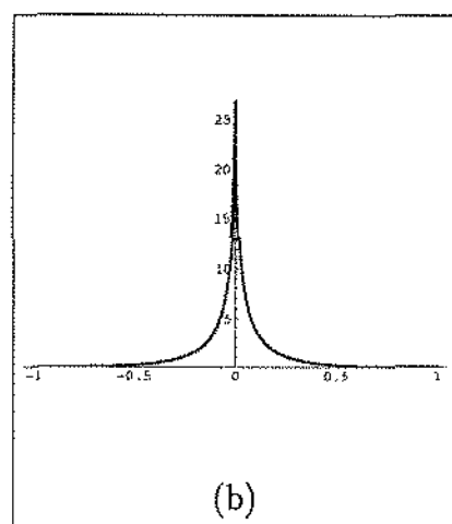
Figura 2.5: (a) Núcleo de redistribuição com suporte compacto dado pela expressão k(x) = a - b \ln(|x|) , a e b constantes positivas. (b) Núcleo de redistribuição com cauda exponencialmente limitado, descrito por k(x) = \exp[a - b\sqrt{|x|}] , a e b constantes positivas.
