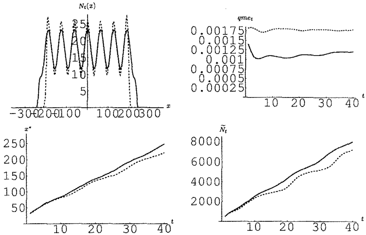
Figura 3.30: Comparação entre o modelo de taxa por recursos existentes (linha pontilhada) e o modelo de taxa por recursos disponíveis (linha cheia) para qualidade tipo seno para \mu = 0.25 e \alpha = 0.01 . (a) A solução N_t(x) dos dois modelos na iteração final; (b) evolução da qualidade média experimentada; (c) frente de onda e (d) evolução da população total.
