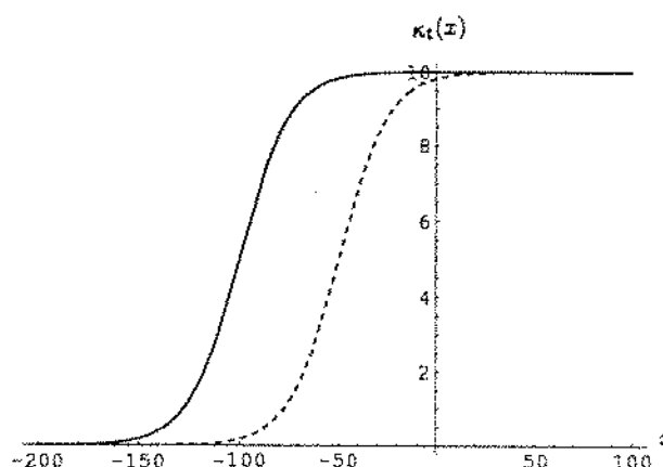
Figura 3.4: Capacidade suporte variável no espaço e no tempo. No sentido de x negativo a capacidade suporte nula indica a impossibilidade de sobrevivência das abelhas africanizadas nestas regiões. A linha cheia indica o avanço da fronteira natural em direção ao sul durante os meses quentes do verão enquanto a linha pontilhada representa a capacidade suporte correspondente aos meses mais frios do outono, inverno e primavera.
