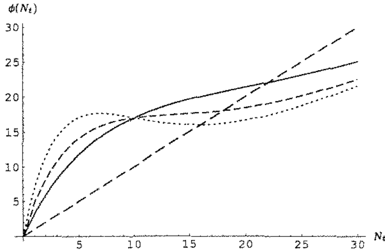
Figura 3.1: Ilustração da função \phi(N_t) que atualiza o número de colônias em cada iteração para diversos valores de r . Assume um efeito de saturação dependente da densidade. A intersecção de cada curva com a reta pontilhada y = x representa o respectivo ponto de equilíbrio não nulo \bar{N}_2 .
