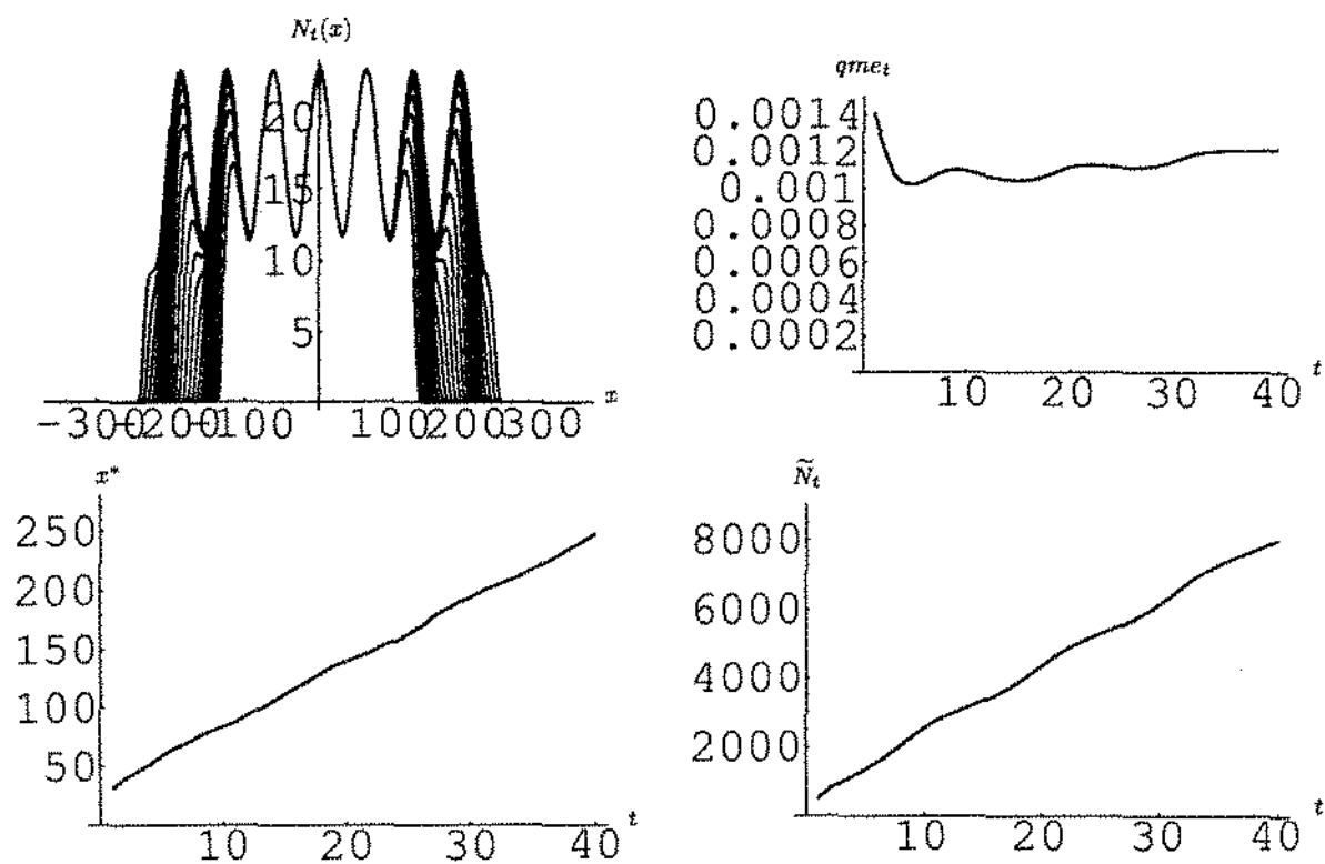
Figura 3.26: Solução obtida com o modelo de taxa por recursos disponíveis com qualidade tipo seno: (a) As vinte últimas iterações; (b) evolução da qualidade média experimentada; (c) frente de onda nos dois sentidos do domínio e (d) evolução da população total com o tempo.
