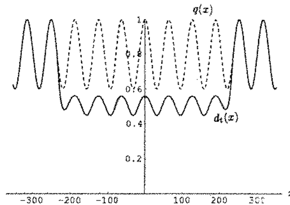
Figura 3.27: Função disponibilidade na última iteração. A linha pontilhada representa a função qualidade, que foi modificada.
