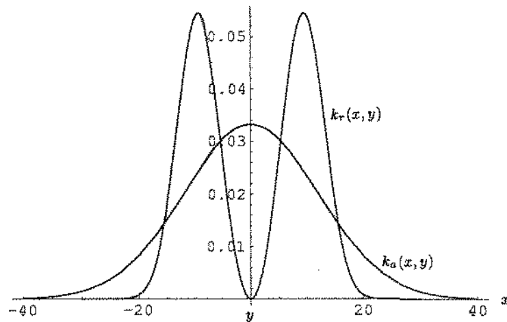
Figura 3.3: Gráfico do núcleo de redistribuição para abandonos e do núcleo de redistribuição para enzimas reprodutivos. Representam a probabilidade de uma colônia na posição y = 0 migrar para cada posição x do domínio, por abandonos ou enzimas reprodutivos.
