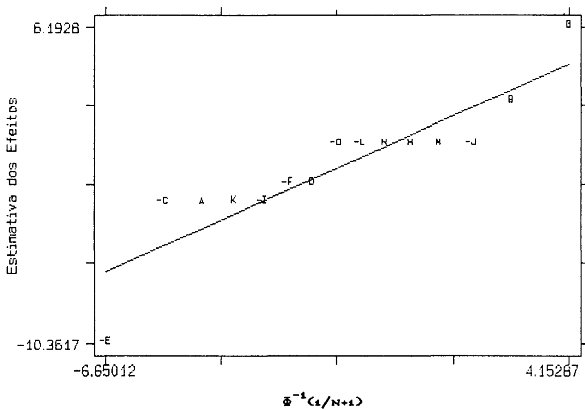
Figura 3.1 - Gráfico probabilístico normal dos efeitos principais dos fatores, estimados segundo os princípios da AA para os dados do Exemplo B.
