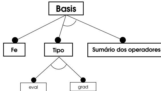
Figura 5.5: DSL para o conceito “base de elementos finitos”.
