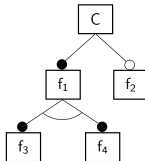
Figura 5.1: Exemplo de diagrama de características.
