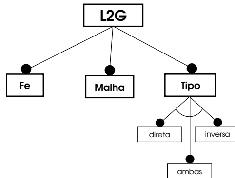
Figura 5.6: DSL para transformação elemento padrão \leftrightarrow elemento real.
