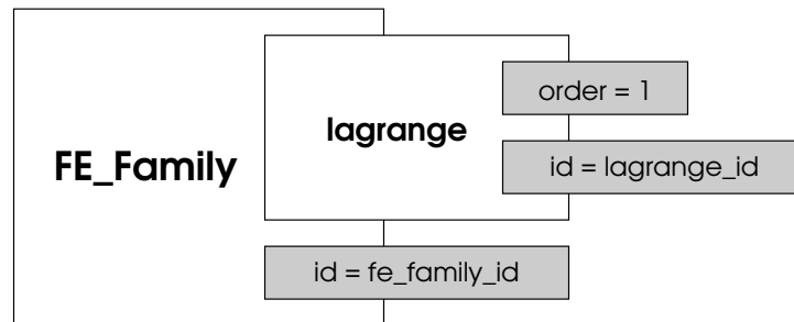
Figura 5.3: Instância de FE_Family< lagrange< 1 > > .
