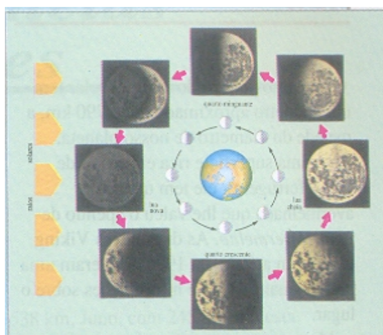
FIGURA 4.18 – Fases da Lua, conforme BRETONES (1993).
