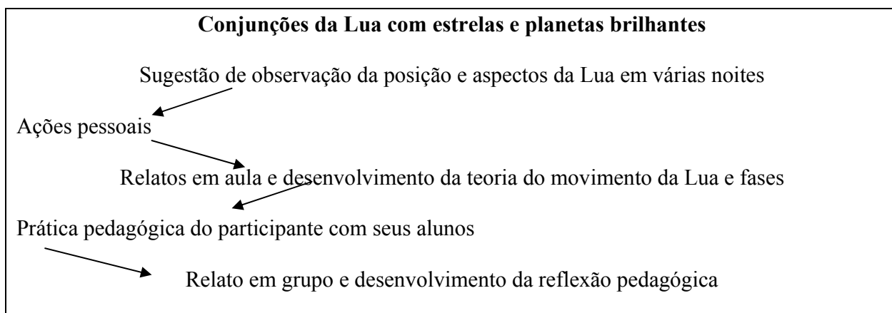
FIGURA 5.5 – Movimentos sugeridos na prática da observação de conjunções da Lua com planetas e estrelas brilhantes.
