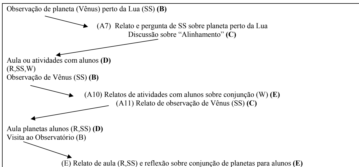
FIGURA 4.13 – Movimentos referentes às observações de Vênus e a Lua, relatos dos participantes e desenvolvimento do tema referente às conjunções dos planetas.
