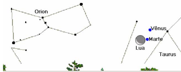
FIGURA 4.11 – Aspecto do céu, na região do horizonte oeste, evidenciando a presença da Lua e os planetas Vênus e Marte no começo da noite de 14 de maio de 2002.
