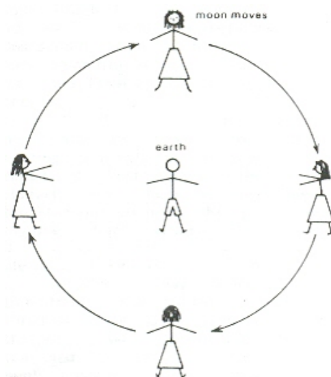
FIGURA 4.20 – Demonstrações de alunos do movimento da Lua ao redor da Terra, conforme OSBORNE (1991).
