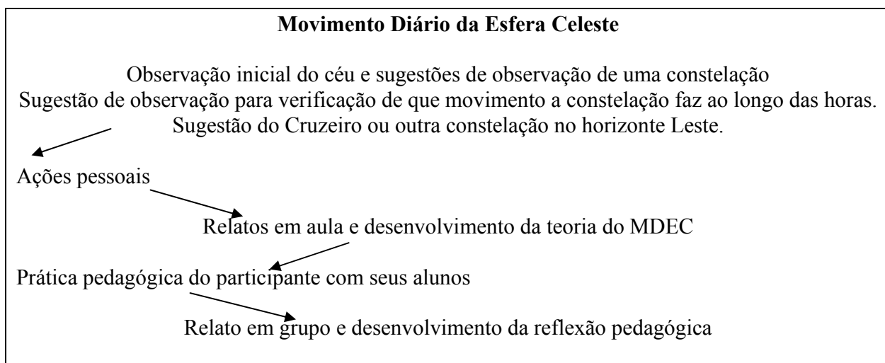
FIGURA 5.4 – Movimentos sugeridos na prática de observação e desenvolvimento do conteúdo sobre o movimento diário da esfera celeste.
