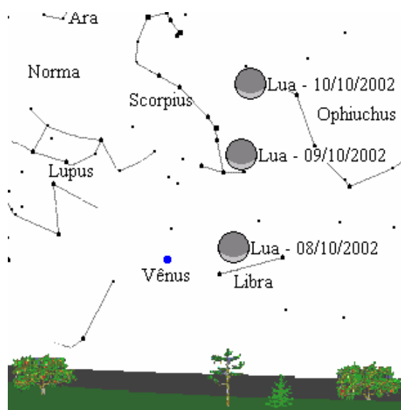
FIGURA 4.19 – Aspecto do céu, na região do horizonte oeste, evidenciando a presença da Lua e o planeta Vênus, no começo das noites de 08, 09 e 10 de outubro de 2002.
