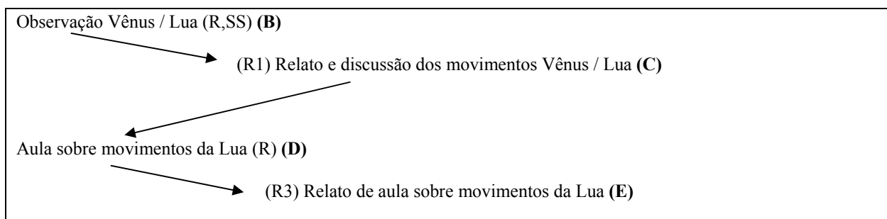
FIGURA 4.22 – Movimentos referentes às observações de Vênus e a Lua, relatos dos participantes e desenvolvimento do tema referente aos movimentos da Lua.
