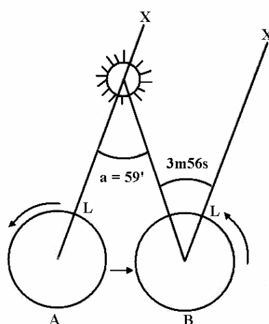
FIGURA 4.25 - Movimento da Terra de um dia para outro entre as posições A e B, conforme BARROS (1978), adaptado.
