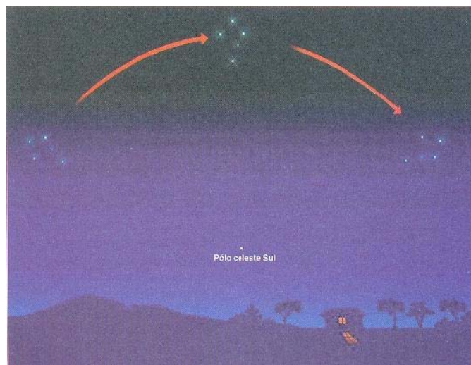
FIGURA 4.5 – Movimento da constelação do Cruzeiro do Sul ao redor do pólo celeste Sul (sentido horário), conforme BRETONES (1995).
