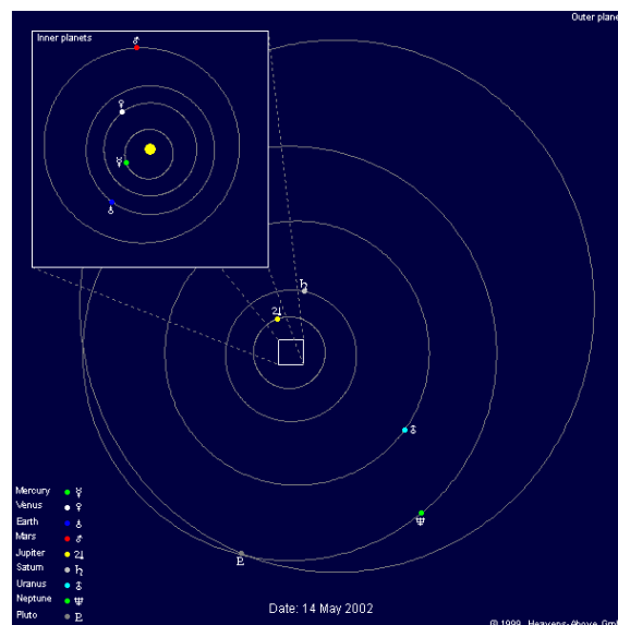
FIGURA 4.12 – Posições dos planetas nas respectivas órbitas em maio de 2002, conforme (www.heavens-above.com)
