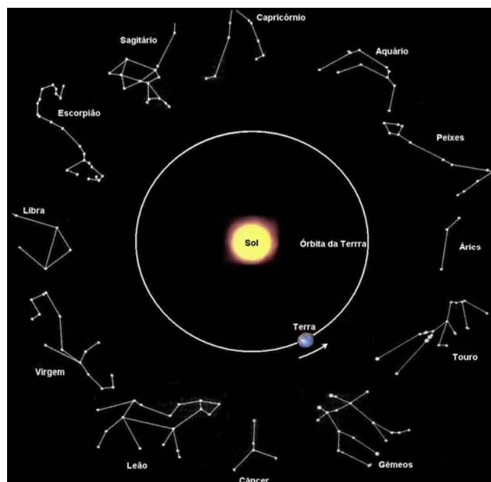
FIGURA 4.15 – Movimento da Terra ao redor do Sol, fora da escala, evidenciando as constelações do zodíaco visíveis ao longo do ano.
