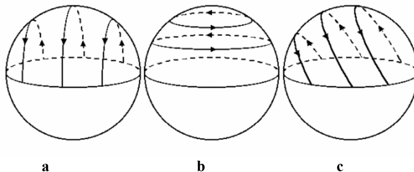
a b c FIGURA 4.4 – Movimento diário da esfera celeste para várias latitudes.
