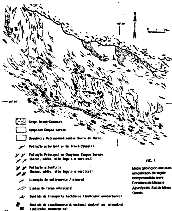
FIG. 1 Mapa geológico estrutural simplificado da região compreendida entre Alpinópolis, Sul de Minas Gerais Figura 32 Mapa estrutural do domínio autóctone entre Alpinópolis e Fortaleza de Minas (Morales et al. 1991).
