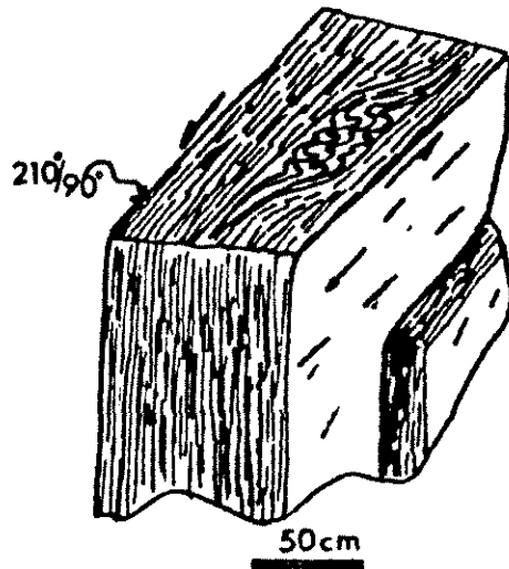
Figura 20 Afloramento do ultramilonito marcado por uma foliação verticalizada e uma fraca lineação sub horizontal. Note a presença de dobras sin-miloníticas assimétricas
