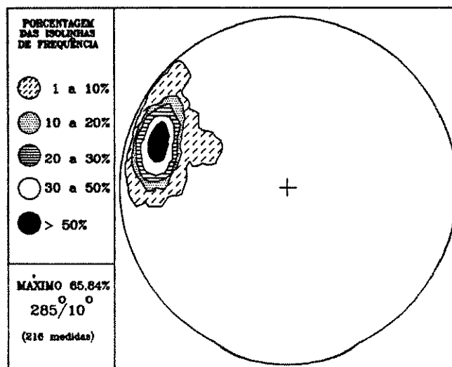
Figura 12 Diagrama de contorno da lineação mineral e de estiramento desenvolvida nas rochas do Bloco Sul.
