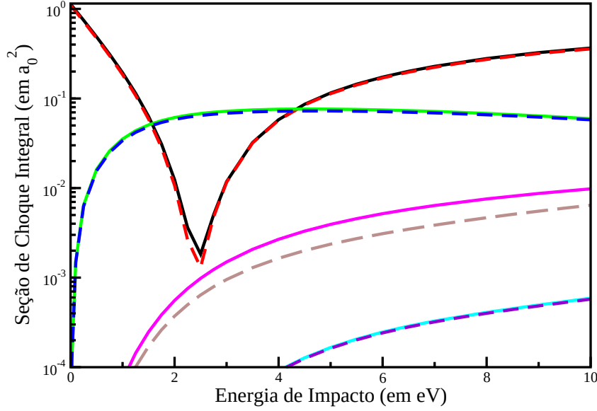
Figura 6.2: Seção de Choque Integral para espalhamento de pósitron por Hélio na aproximação estática mais polarização do alvo. As linhas cheias são os dados atuais e as linhas tracejadas representam os obtidos na conta anterior [51]. Linha preta e linha tracejada vermelha: simetria A_g ; linha verde e linha tracejada azul: simetrias B_{(1,2,3)u} ; linha magenta e linha tracejada marrom: simetrias B_{(1,2,3)g} ; linha ciano e linha tracejada violeta: simetria A_u .
