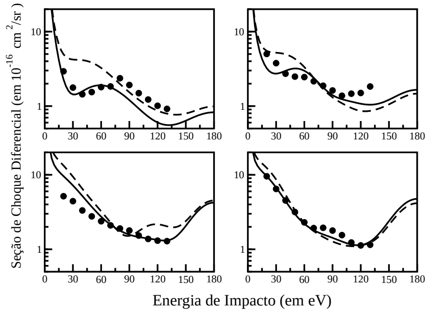
Figura C.4: Seção de Choque Diferencial para espalhamento de elétrons por propeno. Paineis superior esquerdo: 1.5 eV; painel superior direito: 3.0 eV; painel inferior esquerdo: 5.0 eV; painel inferior direito: 7.0 eV. Em todos os gráficos: linha tracejada: conta na aproximação estático-troca; linha cheia: conta na aproximação estático-troca mais polarização; círculos cheios: experimento de [110].
