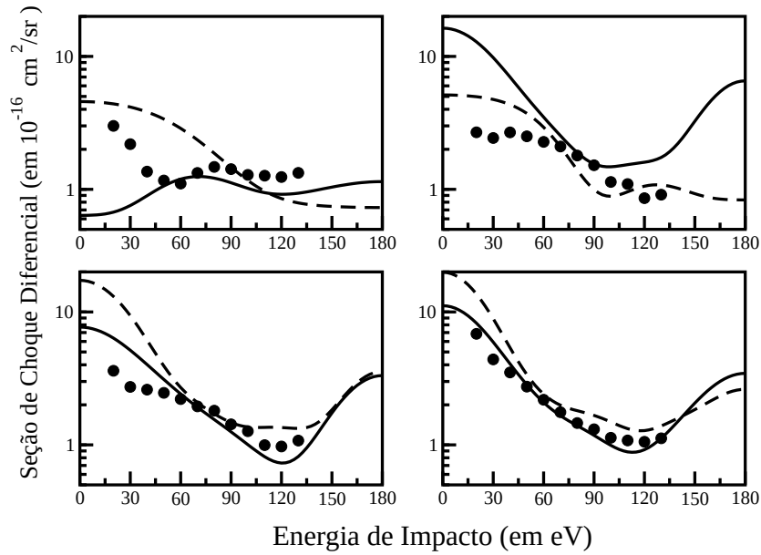
Figura C.3: Seção de Choque Diferencial para espalhamento de elétrons por aléno. Painel superior esquerdo: 1.5 eV; painel superior direito: 3.0 eV; painel inferior esquerdo: 5.0 eV; painel inferior direito: 7.0 eV. Em todos os gráficos: linha tracejada: conta na aproximação estático-troca; linha cheia: conta na aproximação estático-troca mais polarização; círculos cheios: experimento de [110].
