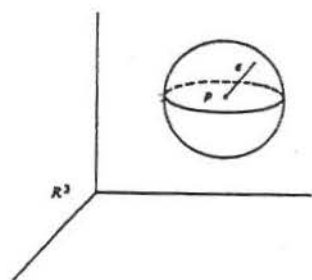
Bola de centro p e raio \varepsilon .
