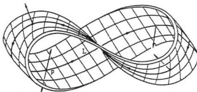
Não-orientabilidade da Faixa de Möbius através de setas.
