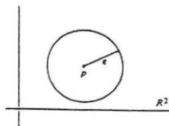
Disco de centro p e raio \varepsilon .
