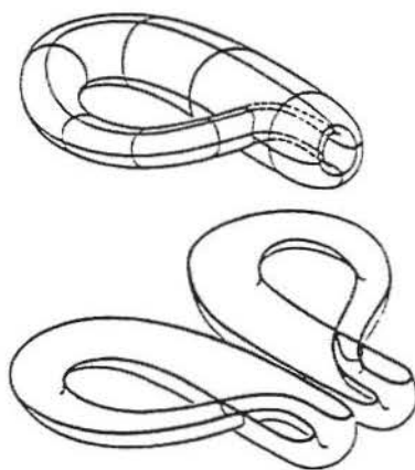
Garrafa de Klein
