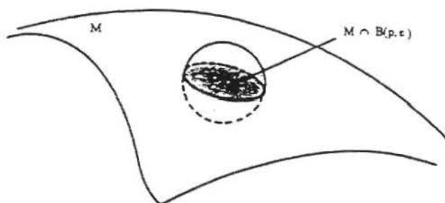
Intersecção de M com a bola B(p, \varepsilon) .
