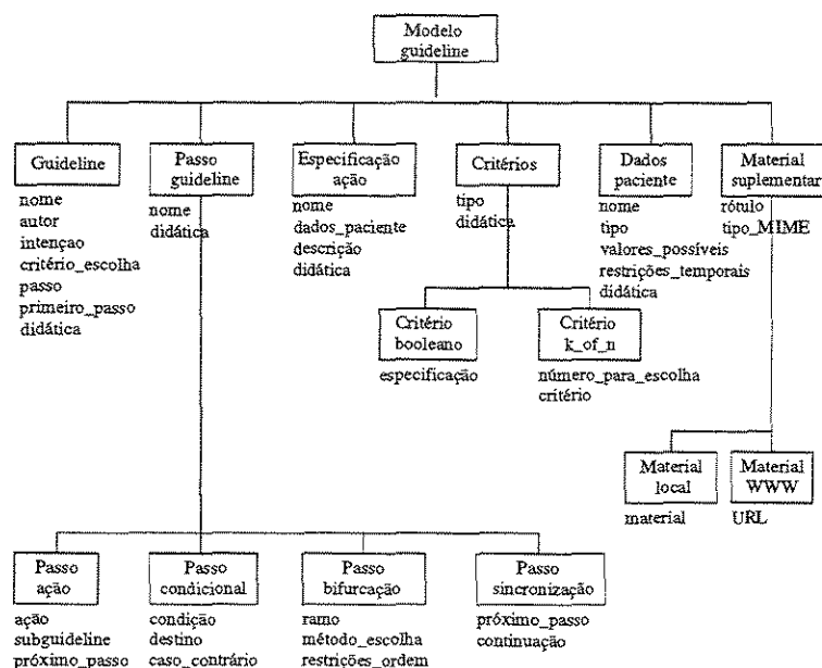
Figura 2.16: Modelo GLIF
