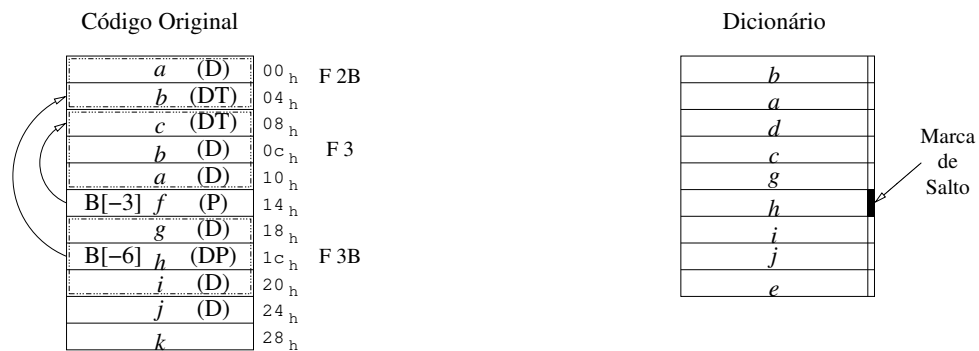
Figura 5.9: Exemplo do algoritmo de compressão: Passo 6
