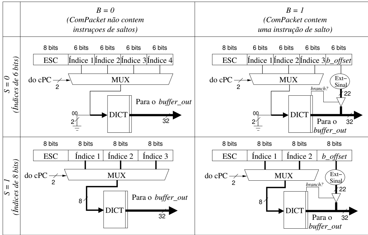
Figura 5.14: Lógica de descompressão para o PDC-ComPacket
