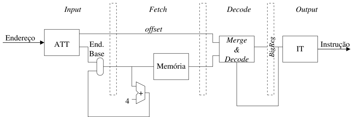
Figura 4.4: Pipeline do descompressor IBC para o Leon
