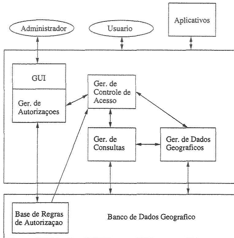
Figura 5.13: Arquitetura do modelo.
