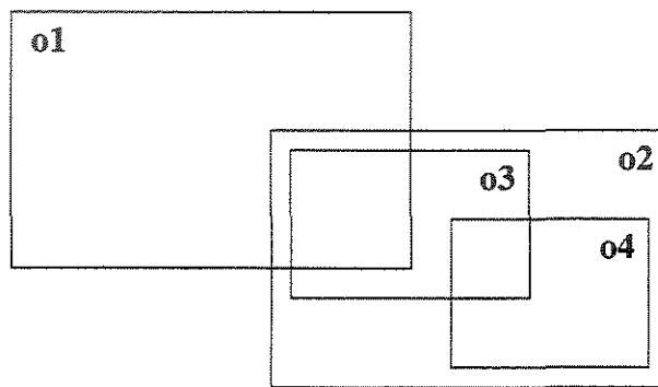
Figura 5.3: Intersecção e continência de polígono.
