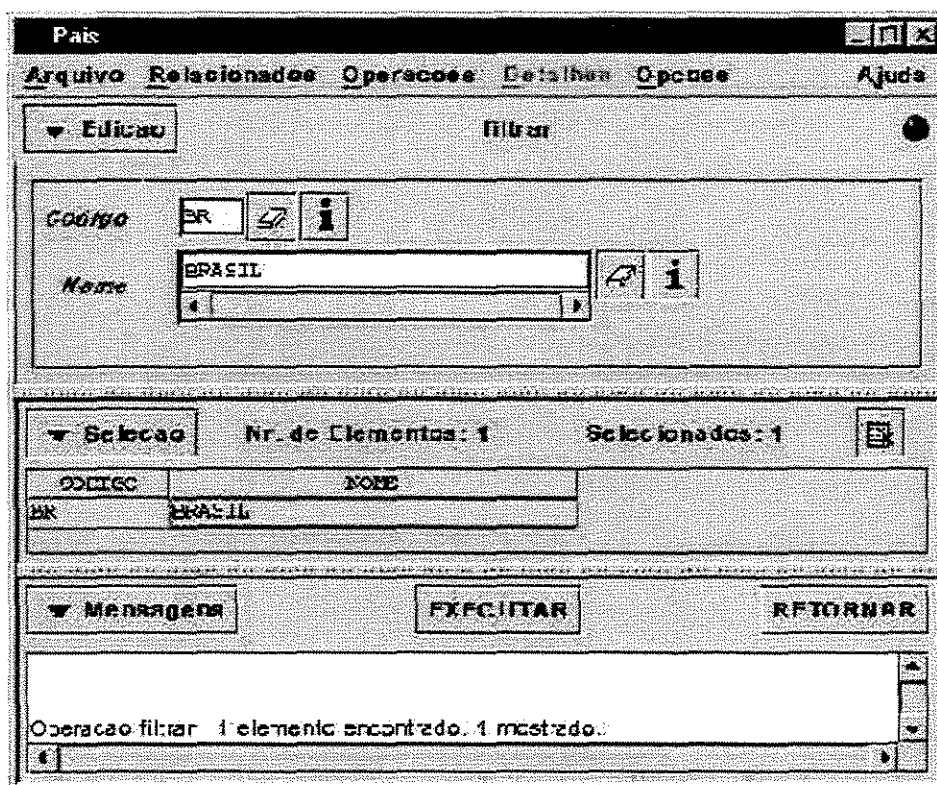
Figura 6.6: Interface de atributos do SAGRE.
