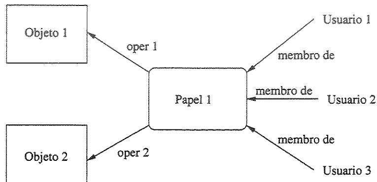
Figura 2.1: Relacionamento entre usuários, papéis, operações e objetos.
