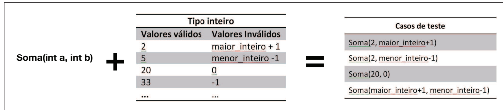
Figura 3.1: Abordagem da Ballista.
