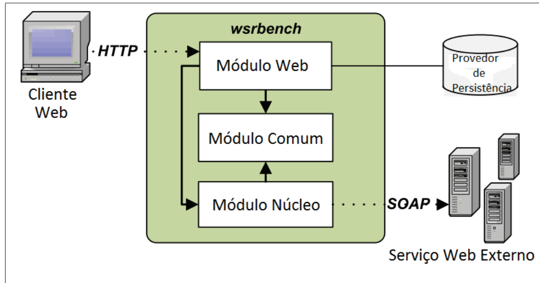
Figura 3.5: Arquitetura da wsrbench [13].
