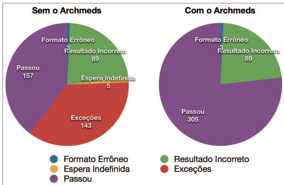
Figura 5.11: Resultados da Campanha 3 reclassificados.
