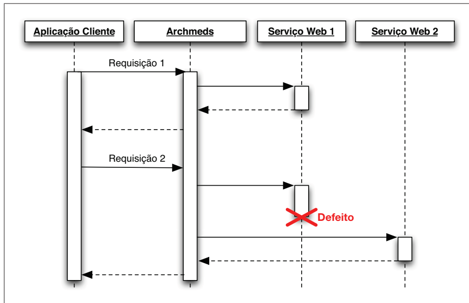
Figura 5.3: Diagrama de sequência de uma mediação confiável.
