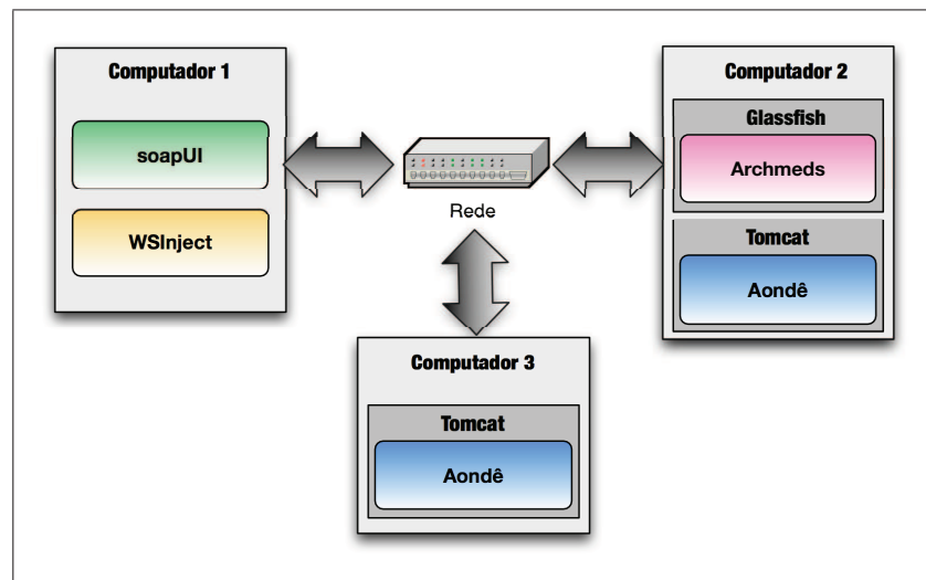
Figura 5.7: Configuração da arquitetura de testes.
