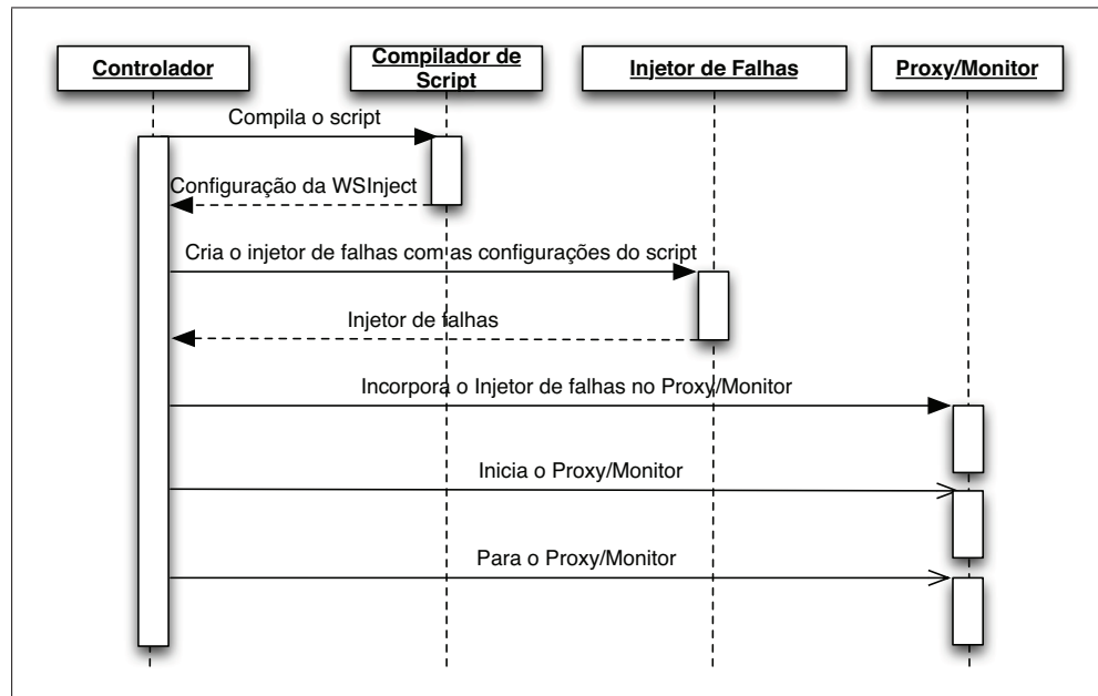
Figura 4.3: Diagrama de sequência da inicialização da WSIInject.
