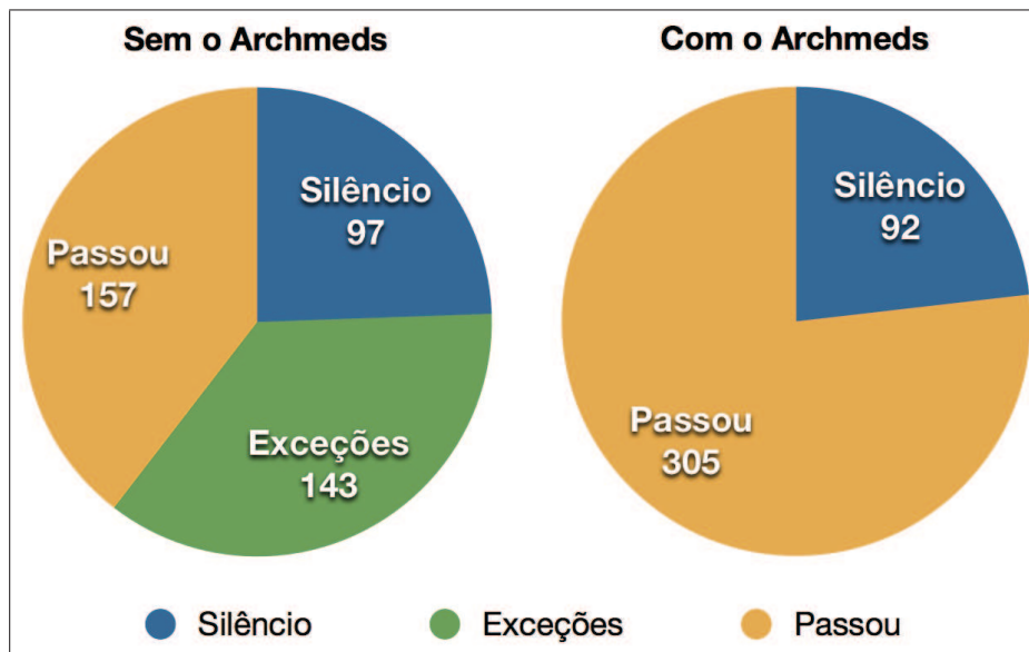
Figura 5.10: Resultados da Campanha 3.
