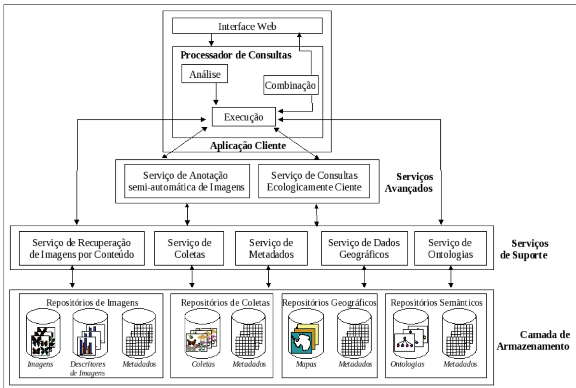
Figura 5.1: Arquitetura do BioCORE [8] apud [11].
