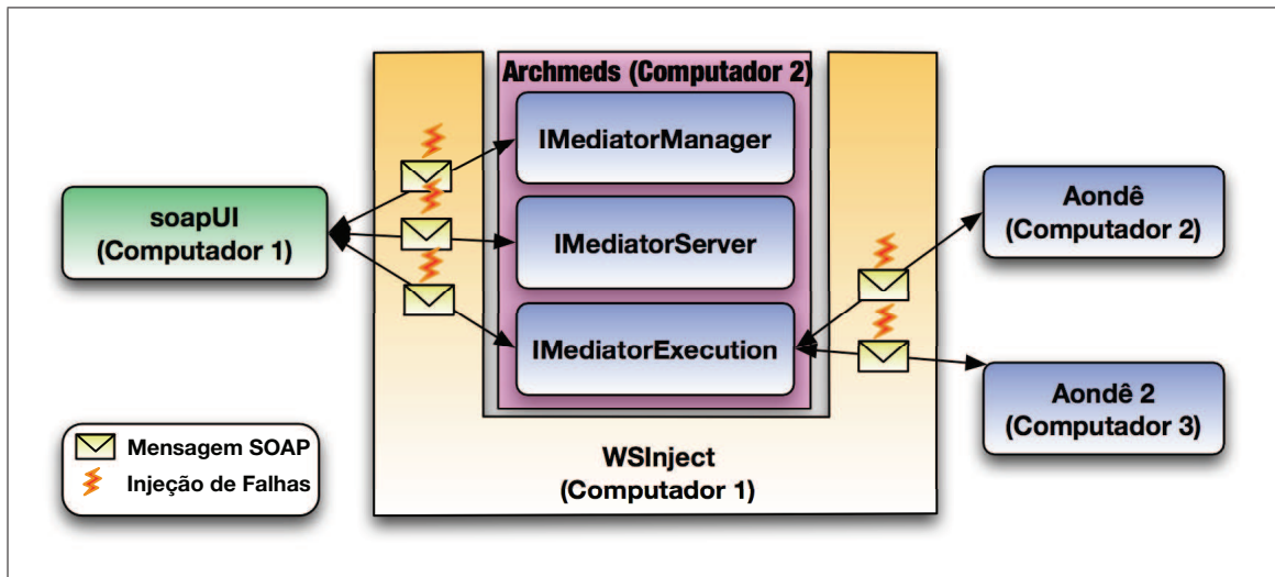
Figura 5.8: Visão lógica da arquitetura de testes.
