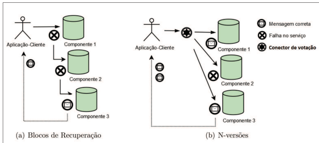
Figura 5.4: Estratégias de tolerância a falhas [8].
