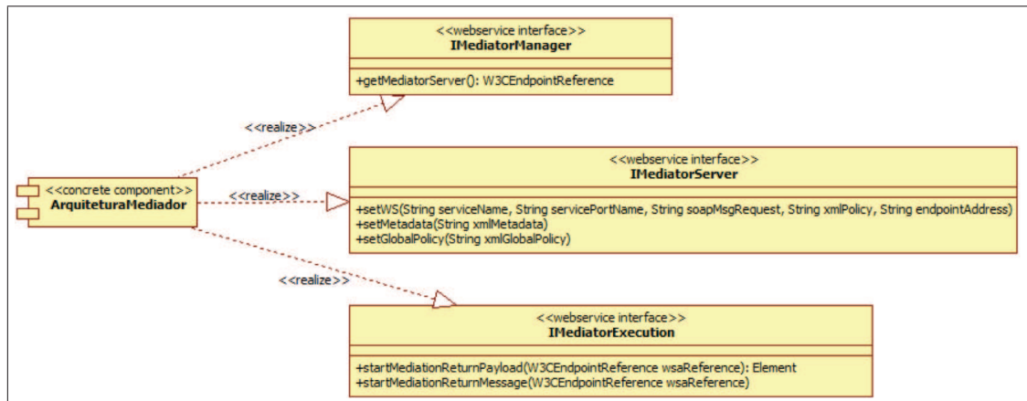
Figura 5.5: Interfaces públicas que compõe o Archmeds.
