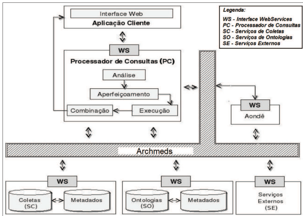
Figura 5.2: Arquitetura do BioCORE com Archmeds [8].
