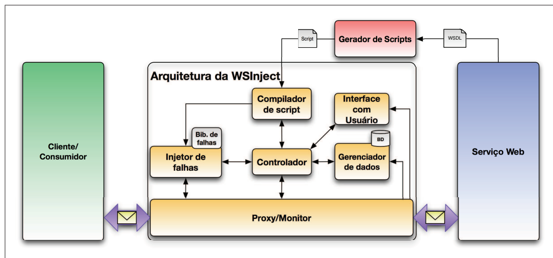
Figura 4.2: Arquitetura da WSInject.
