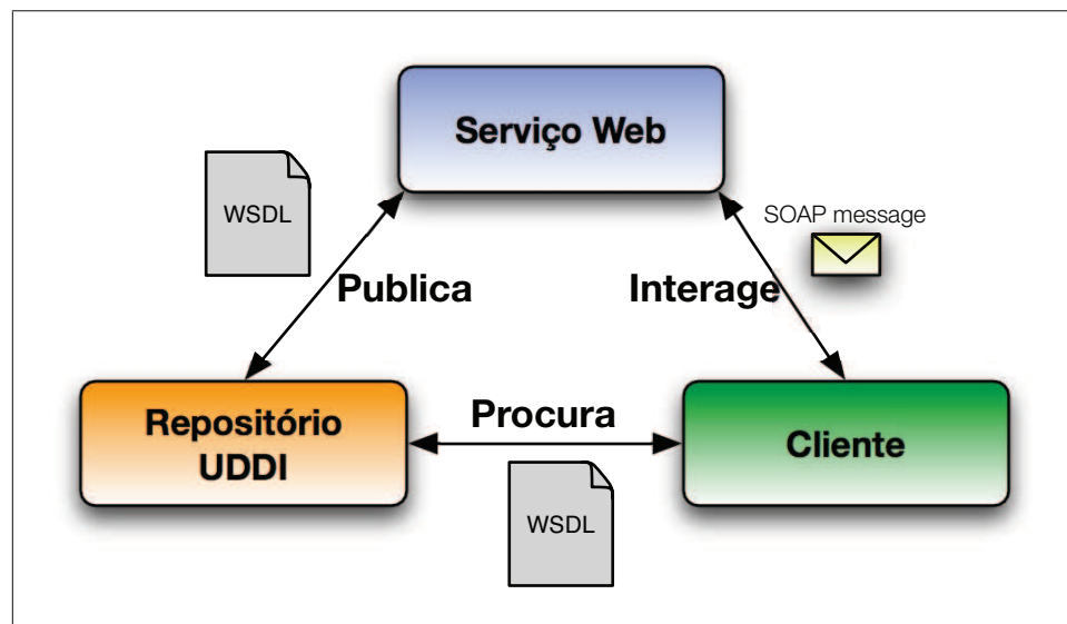
Figura 2.3: SOA com padrão de WSs.
