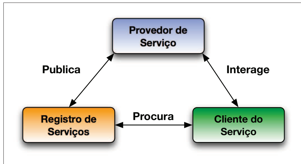
Figura 2.1: Arquitetura orientada a serviços.
