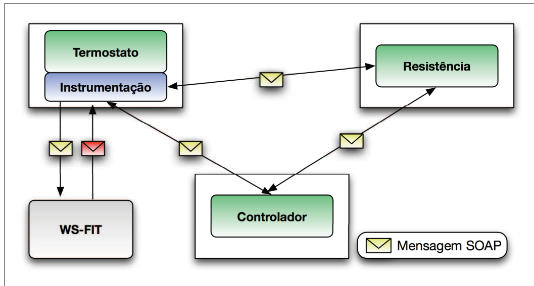
Figura 3.6: Exemplo de como a WS-FIT funciona.
