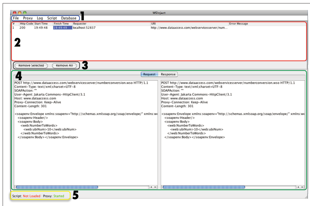
Figura 4.4: Interface gráfica da WSInject.
