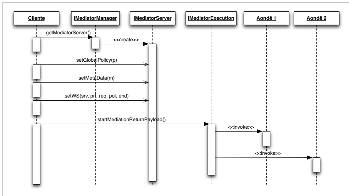
Figura 5.6: Diagrama de sequência do funcionamento do Archmeds.
