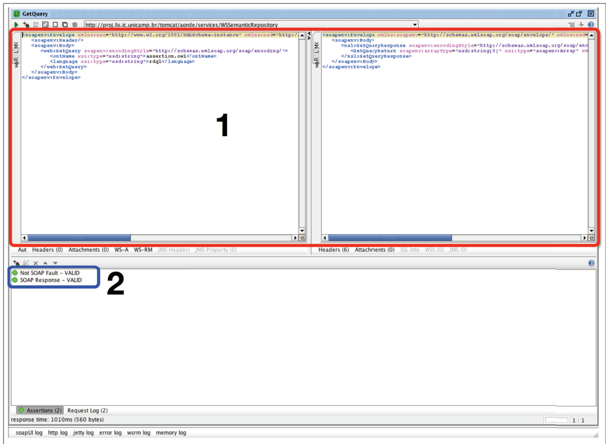
Figura 5.9: Tela do soapUI. (1) Mensagem de requisição e resposta. (2) Assertivas.
