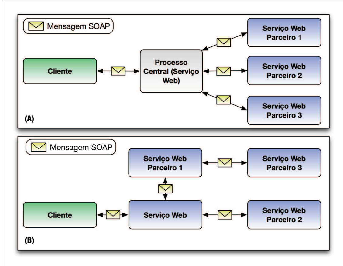
Figura 3.2: (A) Orquestração e (B) Coreografia.
