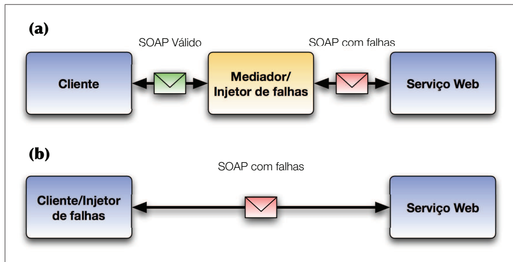
Figura 4.1: (a) Baseada em proxy (b) Baseada em cliente.
