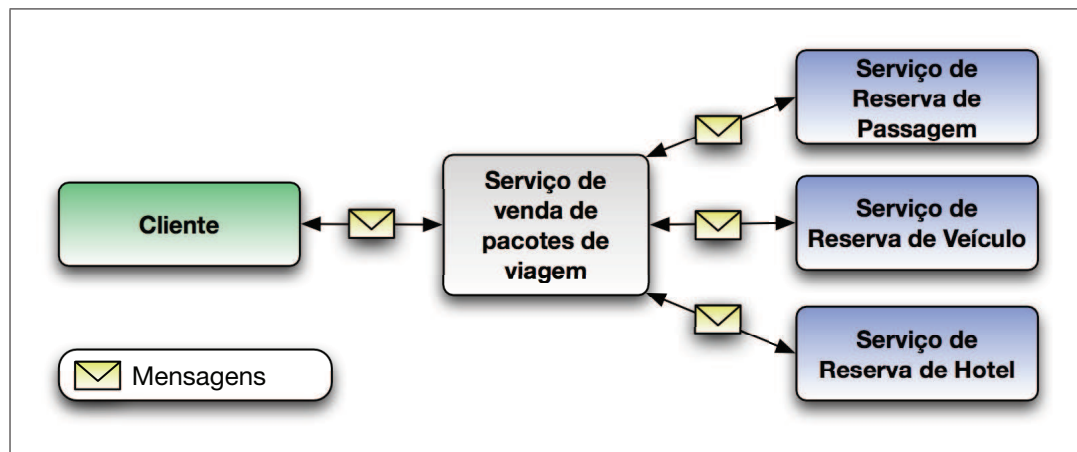
Figura 2.2: Composição de serviços.
