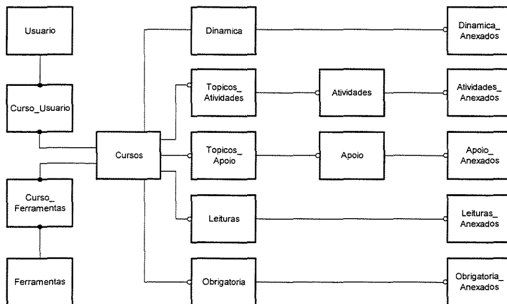
Figura 5.18: Esquema do banco de Dados
