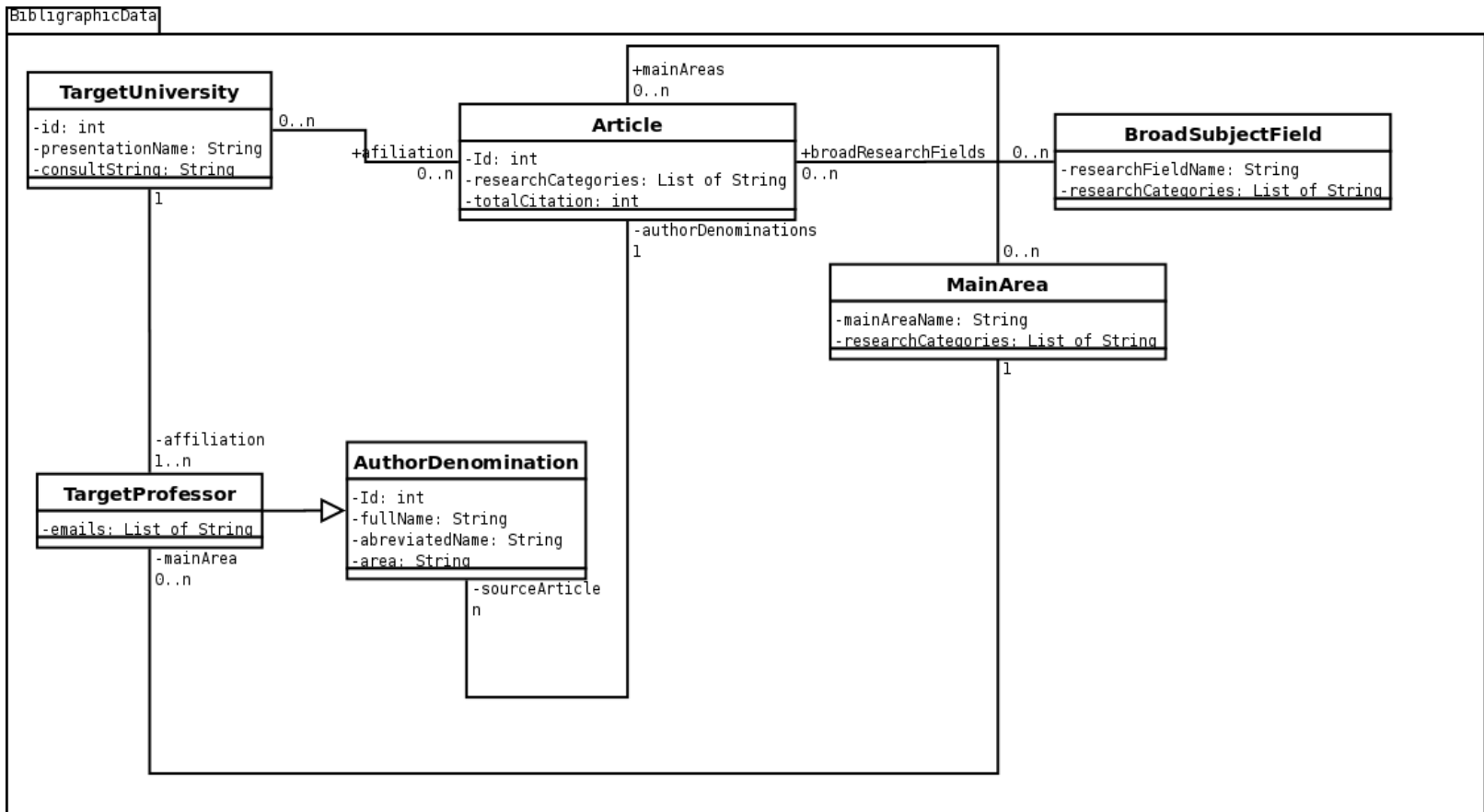
Figura 3.1: Diagrama do modelo da base de dados.
