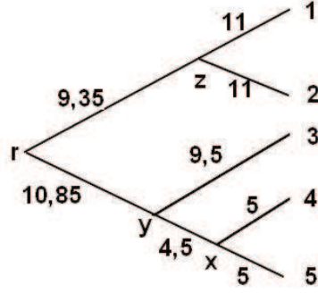
Figura 4.1: Árvore construída com o método UPGMA, com base na matriz de distâncias da Tabela 4.1
