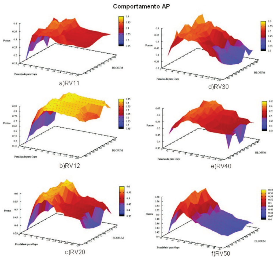
Figura 5.3: Pontuação do alinhador de perfil com alinhamento global (051), com pontuação para gap variando entre -1 e -20, e BLOSUM de 45 a 80. Em a) temos o gráfico para o conjunto RV11, em b) para RV12, em c) para RV20, em d) para RV30, em e) para RV40 e em f) para RV50
