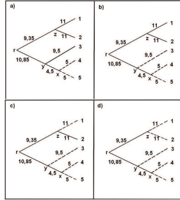
Figura 4.5: Seleção de pares por bloco único para a árvore da Figura 4.1. Linhas tracejadas indicam as seqüências já incluídas no bloco.
