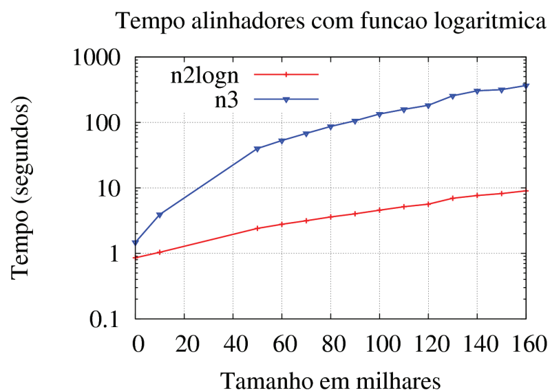
Figura 5.6: Comparação de tempo dos algoritmos de pontuação logarítmica para alinhamento de pares de sequências. No eixo X temos o produto do tamanho das sequências do par (em milhares) e no eixo Y o tempo em segundos que o alinhador utilizou para alinhar os pares de sequências
