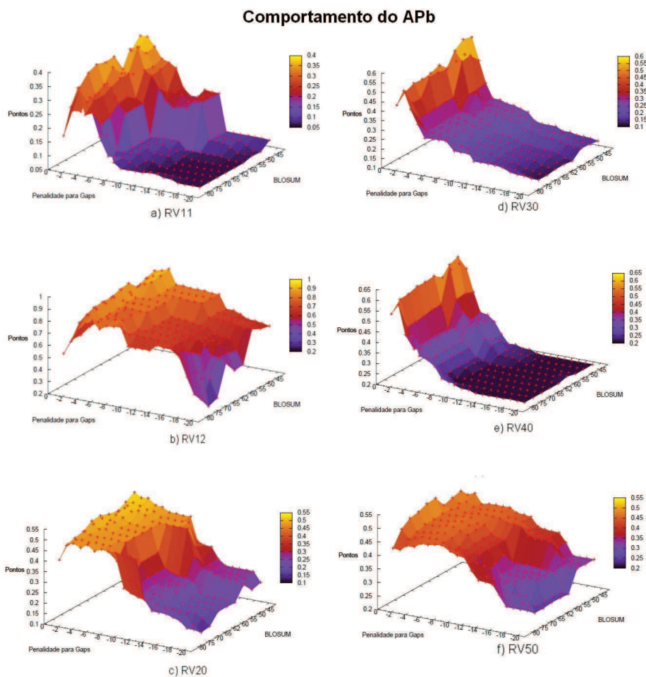
Figura 5.5: Pontuação do alinhador de perfil com alinhamento semi-global (051b), com pontuação para gap variando entre -1 e -20, e BLOSUM de 45 a 80. Em a) temos o gráfico para o conjunto RV11, em b) para RV12, em c) para RV20, em d) para RV30, em e) para RV40 e em f) para RV50
