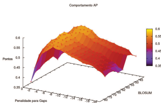
Figura 5.2: Pontuação do alinhador de perfil com alinhamento global (051), com pontuação para gap variando entre -1 e -20 , e BLOSUM de 45 a 80.
