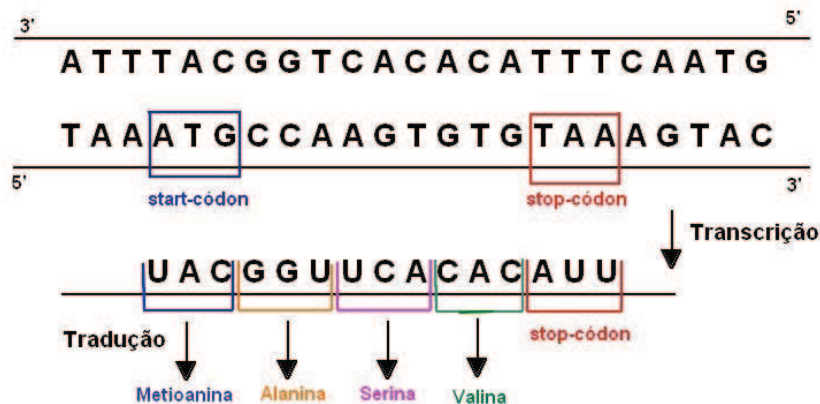
Figura 2.2: Processos de transcrição e tradução dos aminoácidos Metionina, Alanina, Serina e Valina, a partir de uma molécula de DNA.
