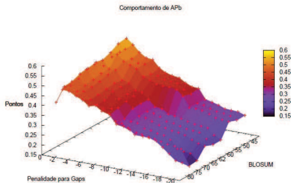
Figura 5.4: Pontuação do alinhador de perfil com alinhamento semi-global (051b), com pontuação para gap variando entre -1 e -20, e BLOSUM de 45 a 80.
