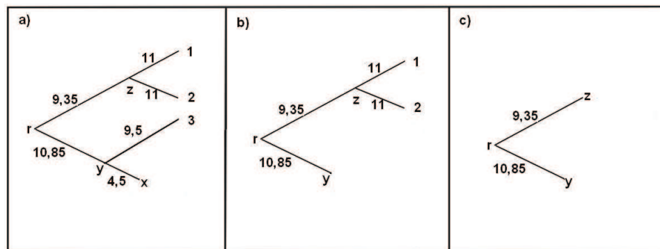
Figura 4.4: Seleção de pares mais próximos para a árvore da Figura 4.1
