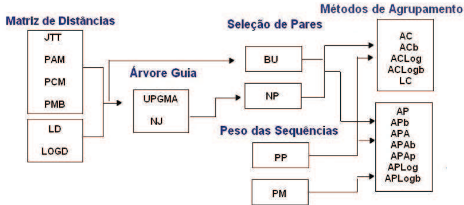
Figura 5.1: Métodos utilizados em cada etapa dos 342 alinhadores múltiplos progressivos construídos
