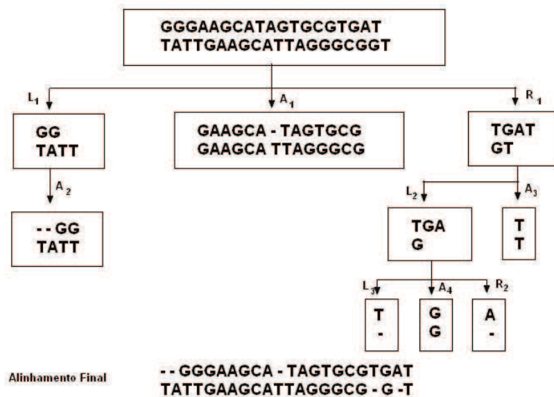
Figura 3.1: Etapas do alinhamento recursivo, Algoritmo 3
