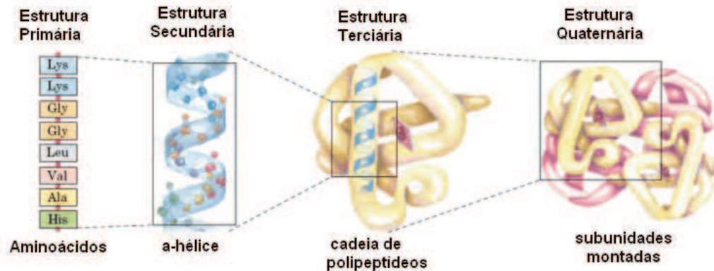
Figura 2.3: Estruturas de uma proteína [39].
