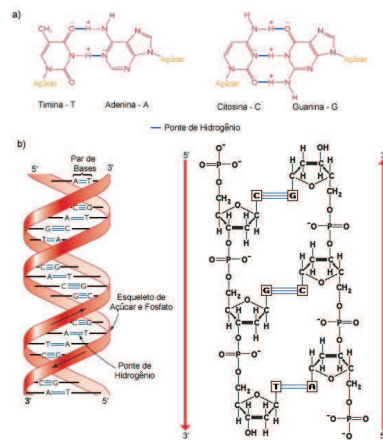
Figura 2.1: a) Bases que compõem o DNA e ligações de bases complementares por pontes de hidrogênio. b) Estrutura de dupla hélice do DNA com terminações 5' (fosfato livre) e 3' (hidroxil livre) [4].
