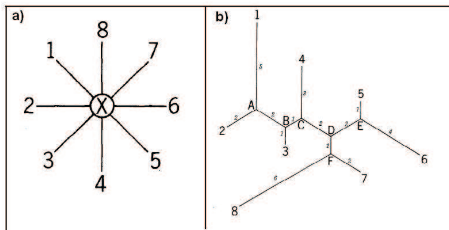
Figura 4.2: a)Árvore estrela, inicial para construção da árvore guia. b)Árvore guia construída pelo método Neighbor Joining [61]
