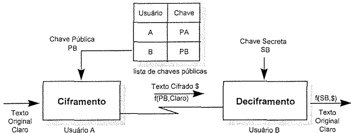
Figura 4.3 - Sistema de Chave Pública para Ciframento.
