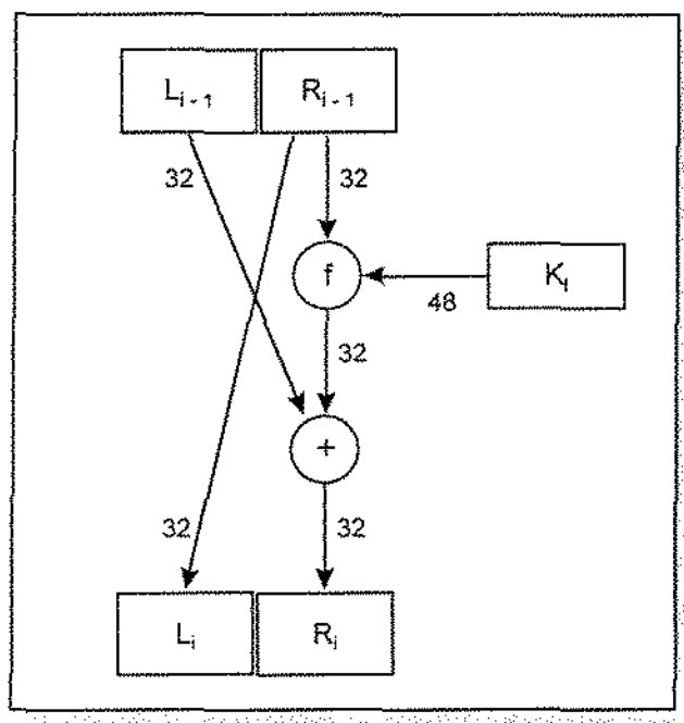
Figura 4.6 - Uma iteração do ciframento DES [Stinson 95].
