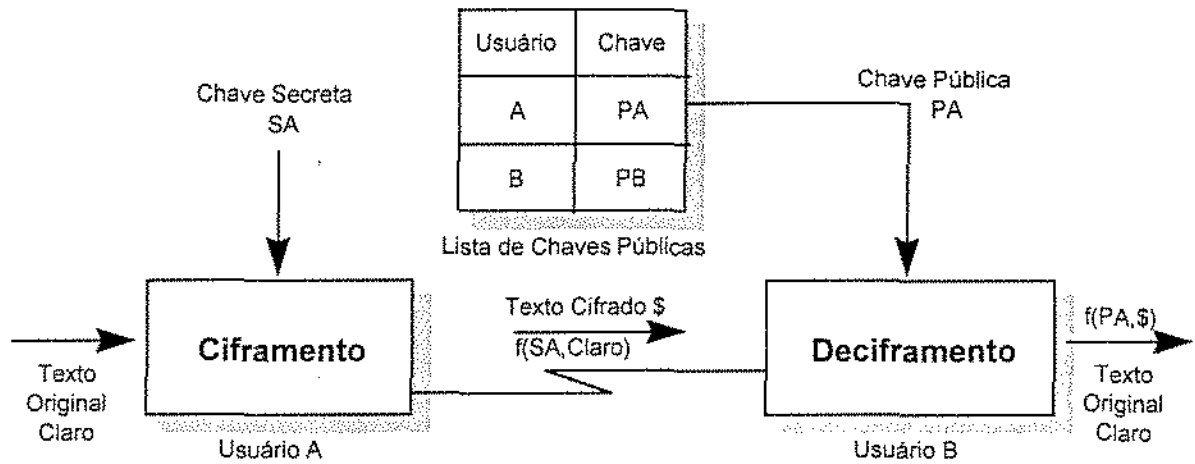
Figura 4.2 - Sistema de Chave Pública Para Autenticação.
