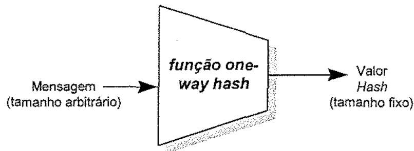
Figura 4.4 - Função One-Way Hash [Schneier 95].
