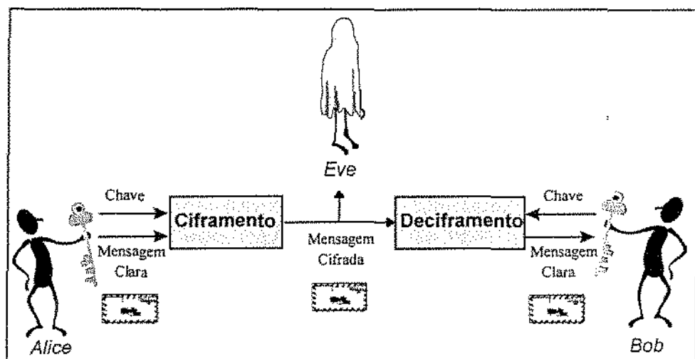
Figura 2.5 - Ciframento e Deciframento com Chave.
