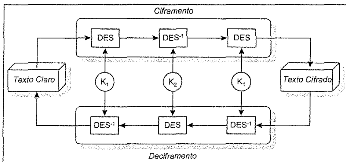
Figura 4.7 - Triplo DES.
