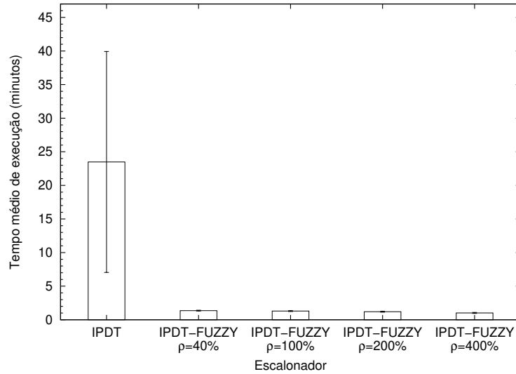
Figura 3.13: Tempo médio de execução para o DAG WIEN2k
