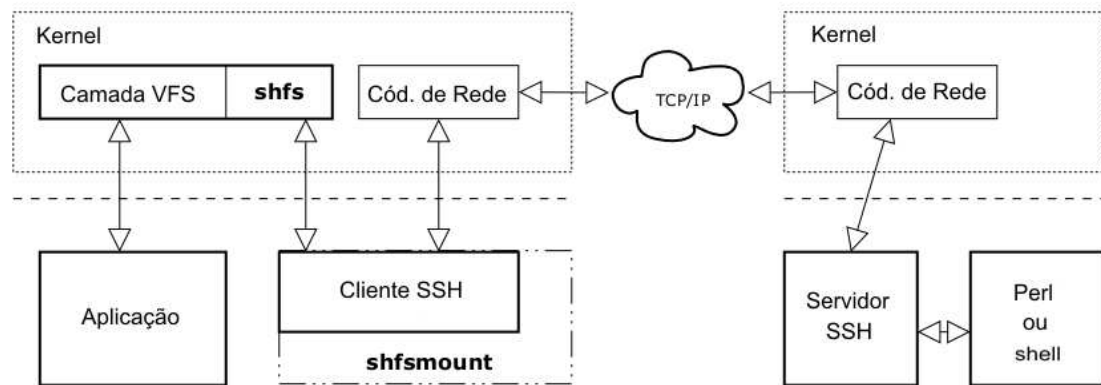
Figura 3.1: Diagrama do SHFS
