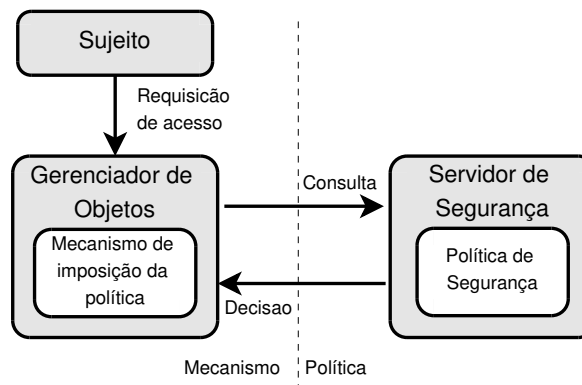
Figura 4.1: Arquitetura Flask
