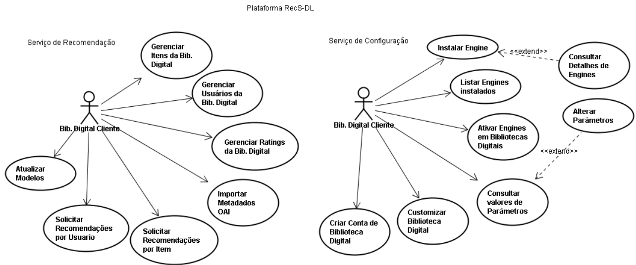
Figura 3.3: Serviços da Plataforma RecS-DL.
