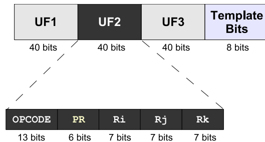
Figura 2.4: Formato de uma instrução IA64
