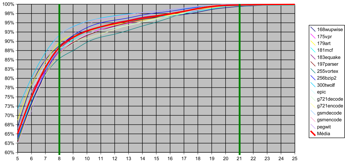
Figura 3.25: Utilização dos campos da palavra PBIW de 128 bits por programa codificado
