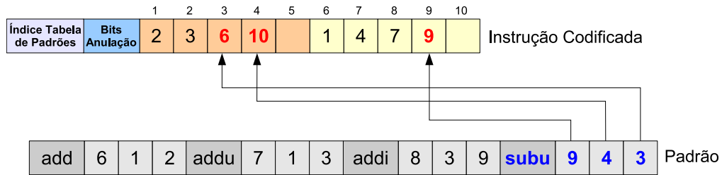
Figura 3.13: Codificação da operação subu r9, r10, r6
