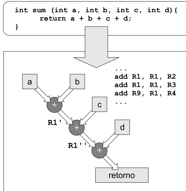
Figura 2.9: Strand composto por três instruções
