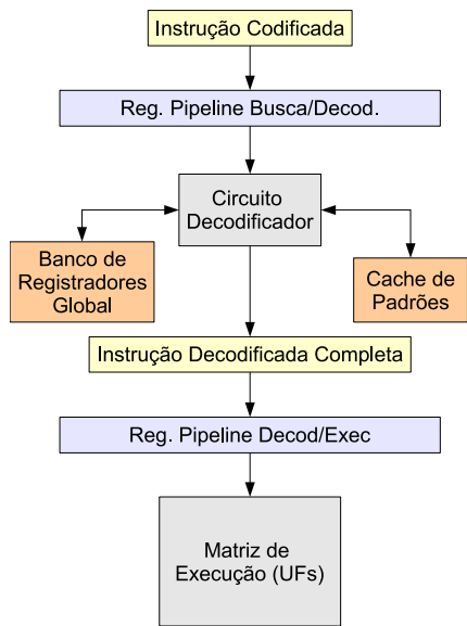
Figura 3.21: Fluxo de decodificação de uma instrução PBIW
