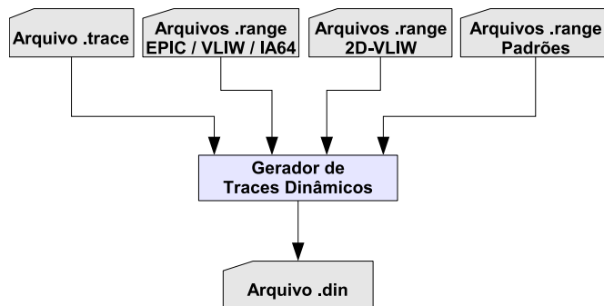
Figura 4.17: Fluxo de execução do Gerador de Traces Dinâmicos
