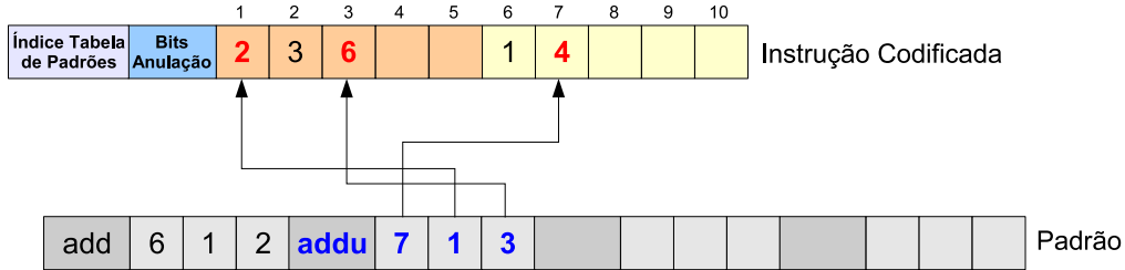
Figura 3.11: Codificação da operação addu r4, r2, r6
