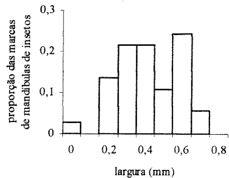
Figura 20. Proporção observada da altura e largura das marcas de mandíbulas de insetos em intervalos de classes de 0,05mm e 0,1mm, respectivamente, para os três tamanho de modelos. Altura: pequeno n=73 ; médio n=58 ; grande n=56 . Largura: pequeno n=63 ; médio n=45 ; grande n=37 .
