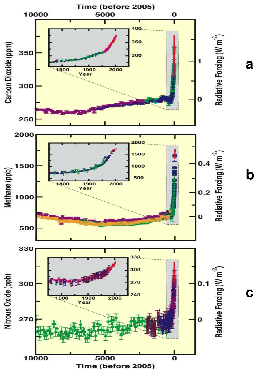
Figura 1. Registro da concentração de \text{CO}_2 (a), Metano (b) e Oxido Nitroso (c) na atmosfera terrestre nos últimos 10.000 anos. Destaque é dado para a aceleração do aumento das concentrações a partir da revolução industrial (IPCC 2007).
