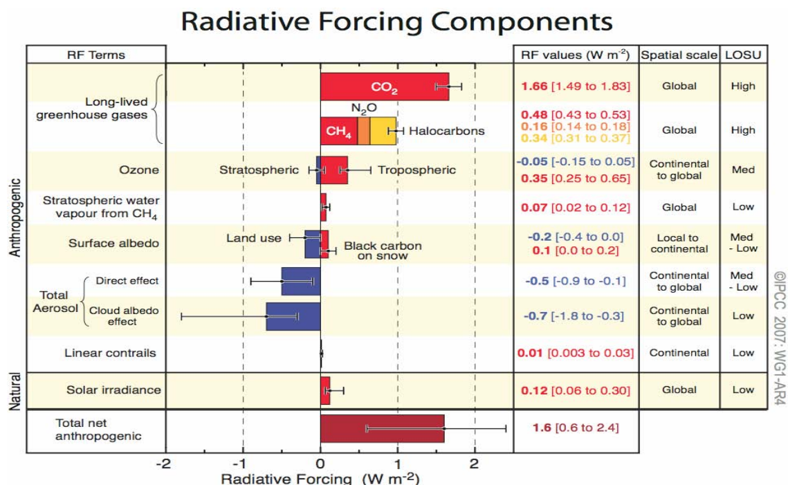
Figura 2. Componentes das forças radiativas que resultam no aquecimento da superfície terrestre (IPCC 2007).
