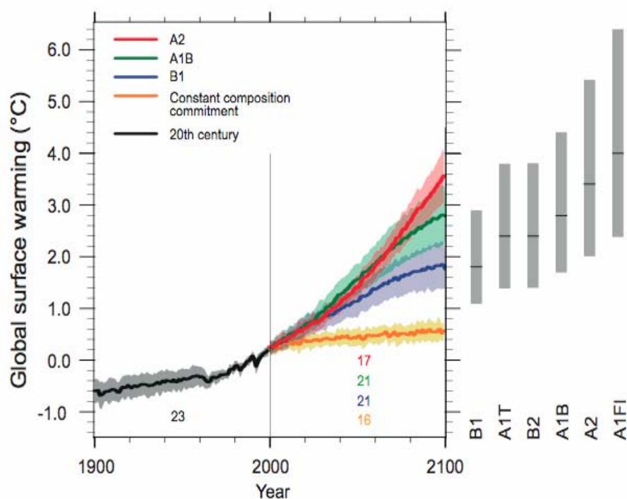
Figura 3. Cenários de aumento da temperatura média da superfície terrestre. O cenário otimista B1 prevê um aumento da ordem de 2^{\circ}\text{C} enquanto que o cenário pessimista A1FI prevê um aumento da ordem de 4^{\circ}\text{C} (IPCC 2007).
