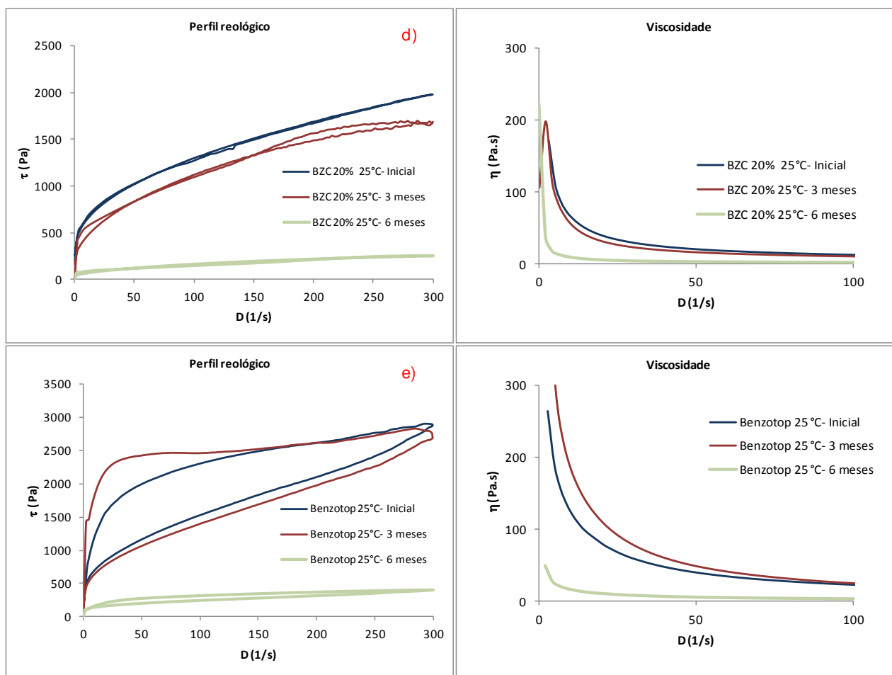
Figura 36. Variação na tensão de cisalhamento (esquerda) e viscosidade (direita) dos géis de Benzocaína em diferentes tempos após preparo (tempo inicial, 3 e 6 meses, medidos a 25°C.
