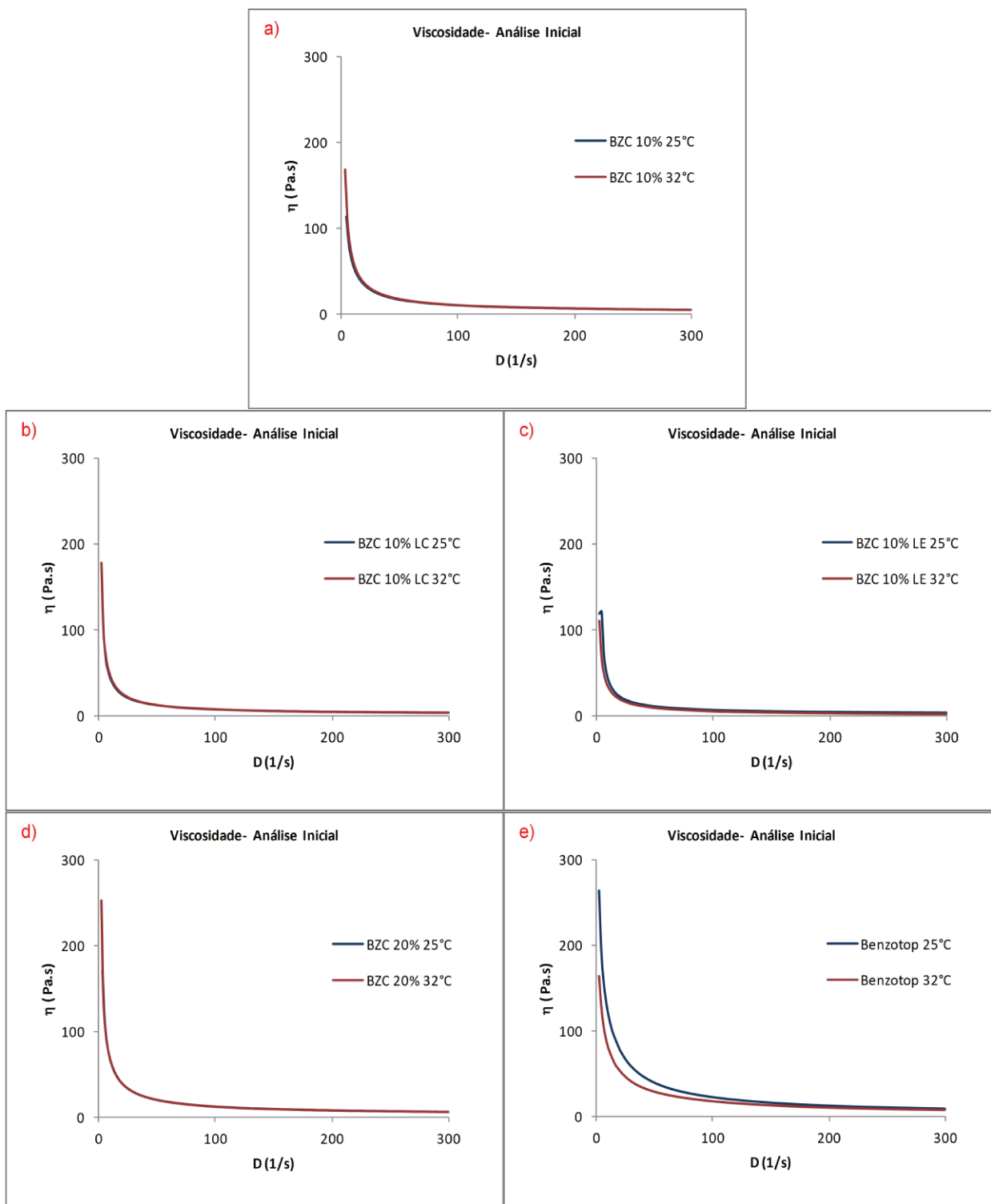
Figura 35. Viscosidade do geis de Benzocaína em diferentes temperaturas (25°C e 32°C).
