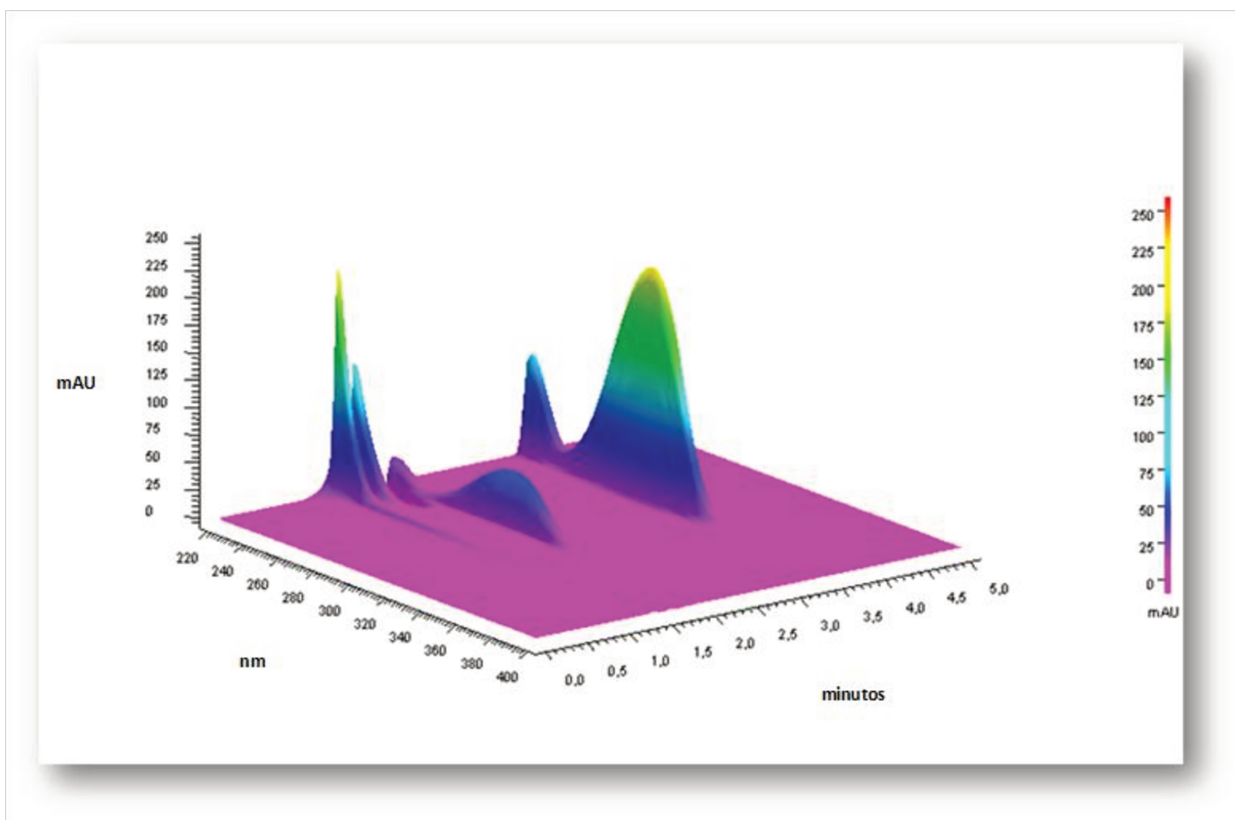
Figura 23. Cromotograma da amostra de gel de benzocaína em 3D, após 10 minutos de exposição ao NaOH 0,1N.
