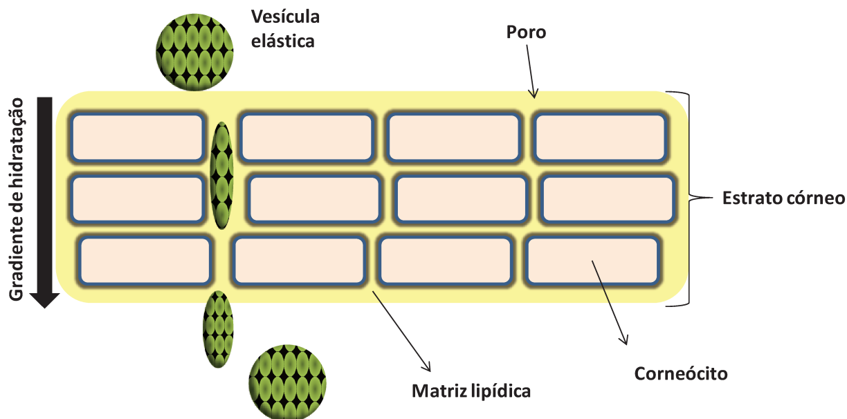
Figura 6. Deformação de lipossomas elásticos durante a penetração entre os poros intercelulares da pele.
