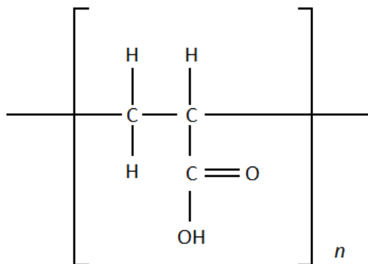
Figura 3. Estrutura química do ácido acrílico, monômero formador do polímero Carbopol
