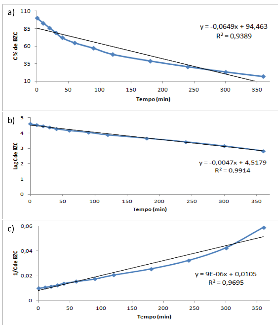
Figura 27. Ajuste dos dados de degradação da BZC em NaOH 0,1N para cinética de a) ordem zero; b) primeira ordem; c) segunda ordem
