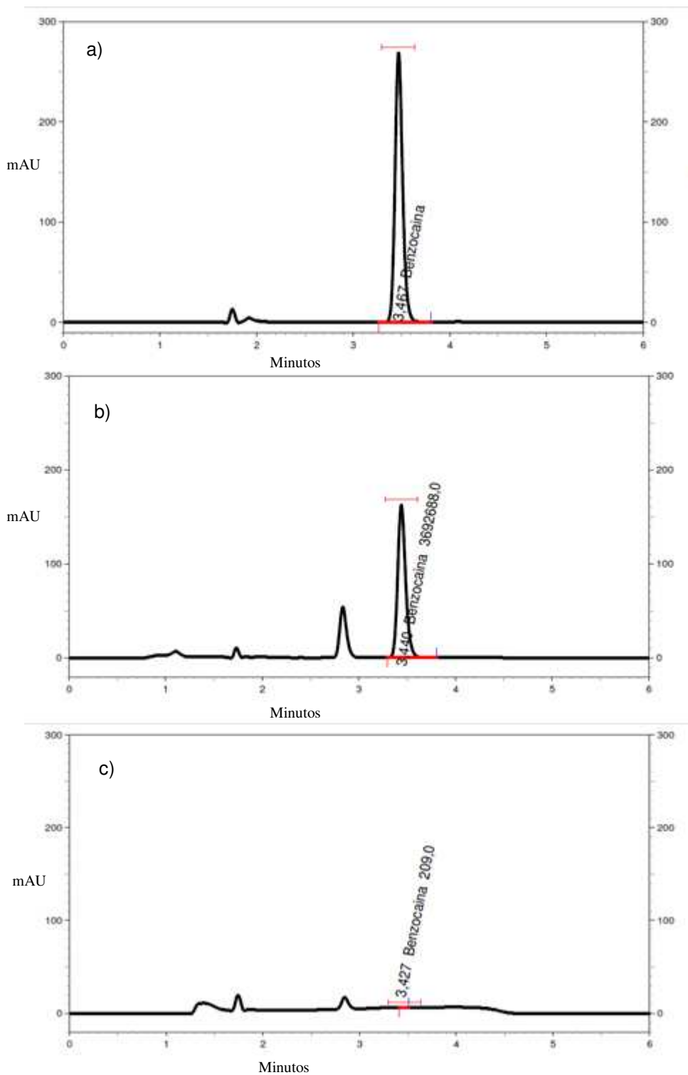
Figura 22. Cromatograma de amostra de gel de benzocaína – (a) amostra inicial sem exposição ao NaOH 0,1N, (b) benzocaína após 10 minutos de exposição ao hidróxido de sódio, (c) após 24 horas de exposição ao hidróxido de sódio.
