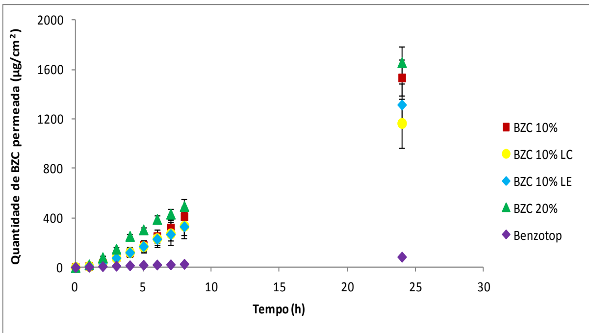
Figura 40. Perfis de liberação de benzocaína ( \mu\text{g}/\text{cm}^2 ) através de pele de orelha de porco a partir das formulações em gel aqui preparadas e da formulação comercial de benzocaína. Dados apresentados como média e desvio padrão ( n= 6-8 )
