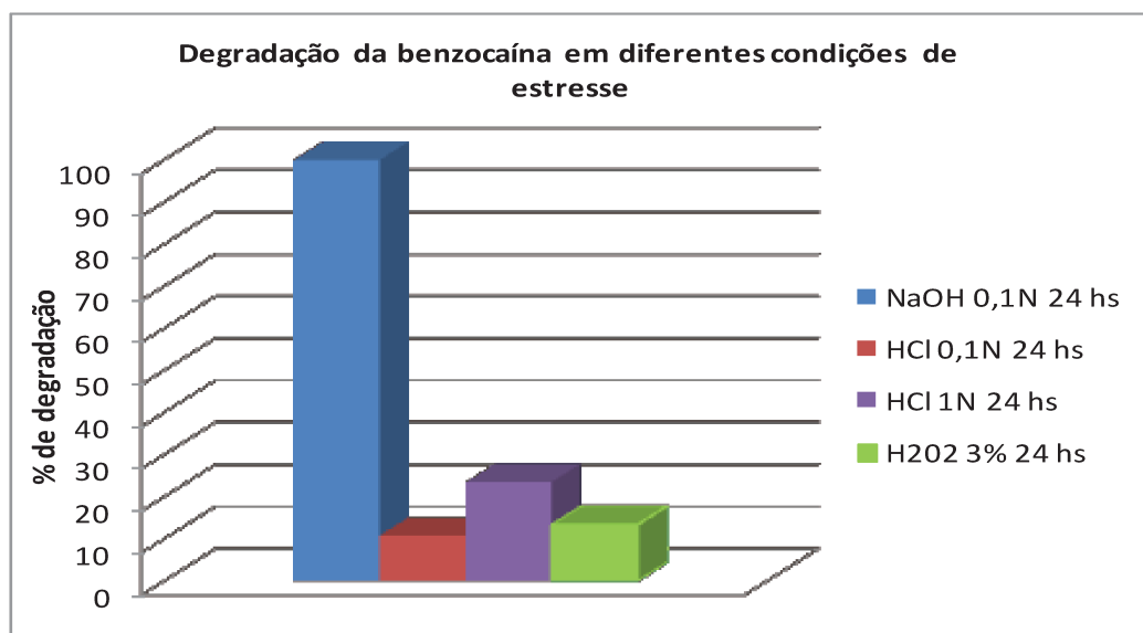
Figura 21. Degradação da benzocaína sob diferentes condições de estresse.
