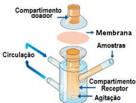
Figura 15. Representação esquemática da célula de difusão vertical (célula de Franz). Adaptado http://www.permegear.com/franz.htm . Acessado em 21 de janeiro de 2010
