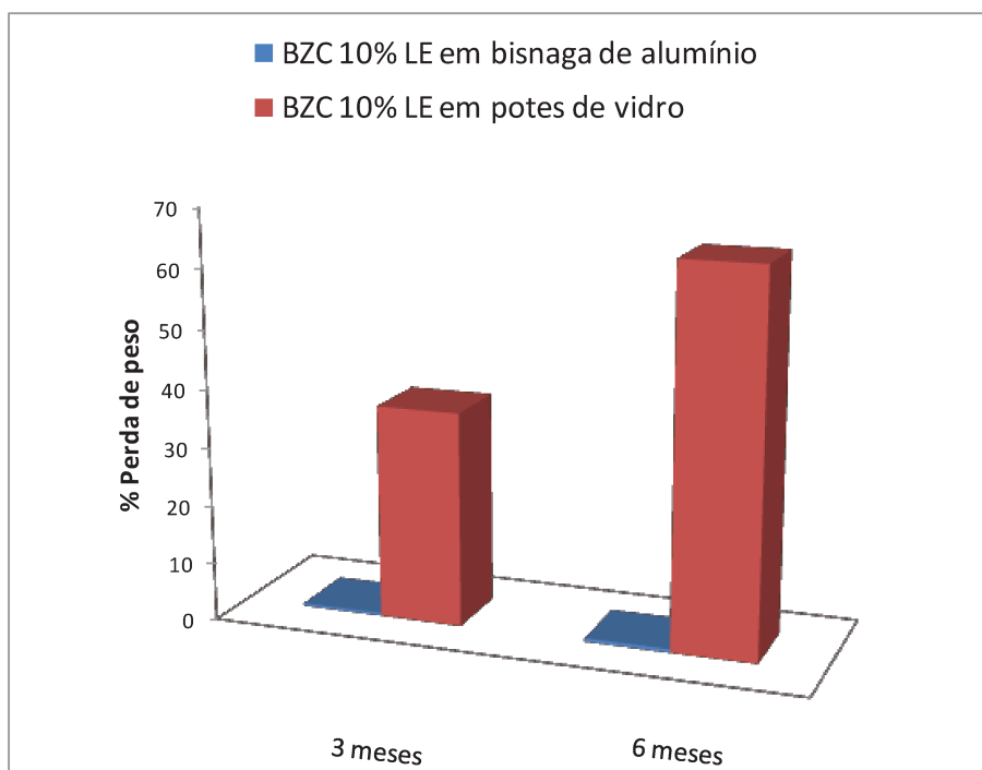
Figura 33. Avaliação de perda de peso das formulações de benzocaína 10% em lipossomas elásticos, após 3 e 6 meses de estabilidade.
