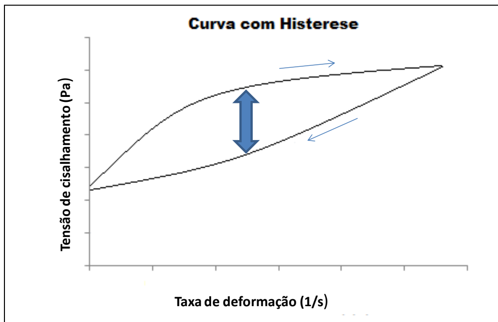
Figura 13. Representação de uma curva de perfil reológico, mostrando o distanciamento (seta azul) entre a curva ascendente e descendente denominado de histerese.
