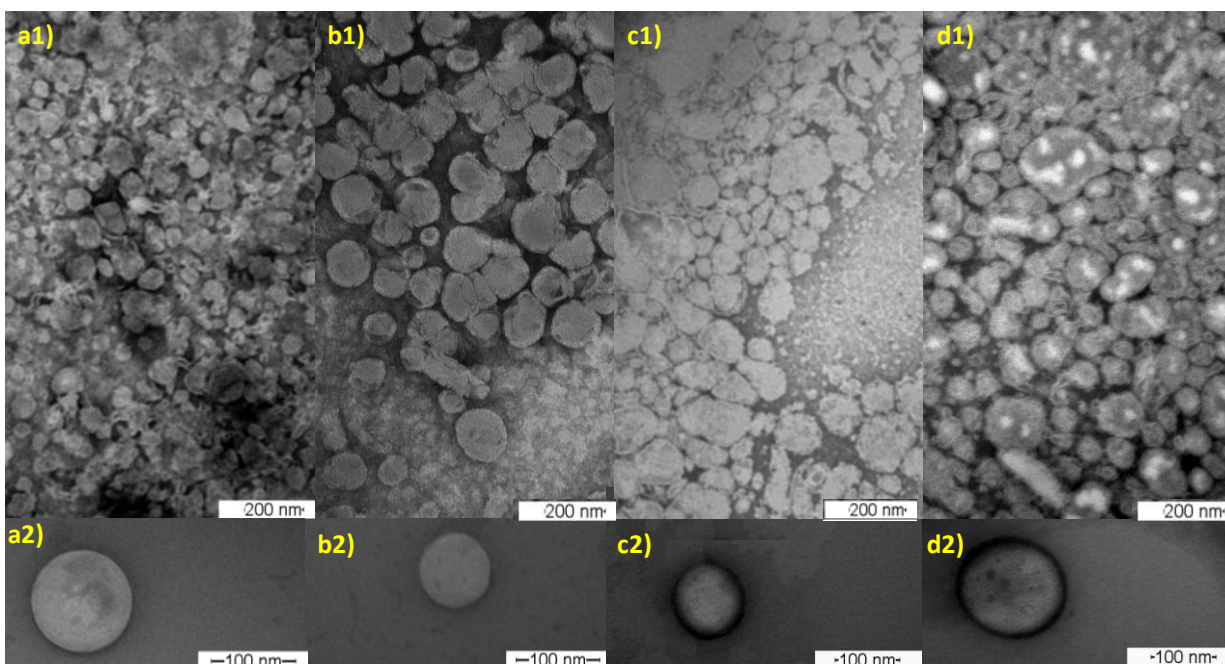
Figura 17. Imagens obtidas em microscopia eletrônica de transmissão dos lipossomas: (a1) lipossomas convencionais (60.000 x), (a2) lipossoma convencional (100.000 x), (b1) lipossomas convencionais contendo BZC (60.000 x), (b2) lipossoma convencional contendo BZC (100.000 x), (c1) lipossomas elásticos vazios (60.000 x), (c2) lipossoma elástico vazio (100.000 x), (c1) lipossomas elástico contendo BZC (60.000 x), (b2) lipossoma elástico contendo BZC(100.000 x),
