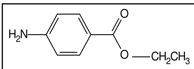
Figura 9. Estrutura química da benzocaína.
