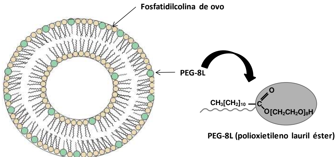
Figura 5. Esquema de um lipossoma elástico formado por moléculas de fosfatidilcolina de ovo e polioxietileno lauril éster (PEG 8-L).
