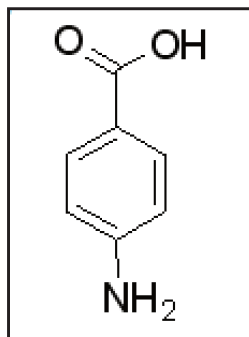
Figura 24. Fórmula estrutural do ácido p-aminobenzóico
