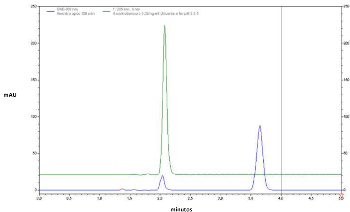
Figura 25. Sobreposição dos cromatogramas de um padrão de ácido p -aminobenzoico (linha verde) e de uma amostra de benzocaína (linha azul), após 120 minutos de exposição ao meio alcalino (NaOH 0,1N).
