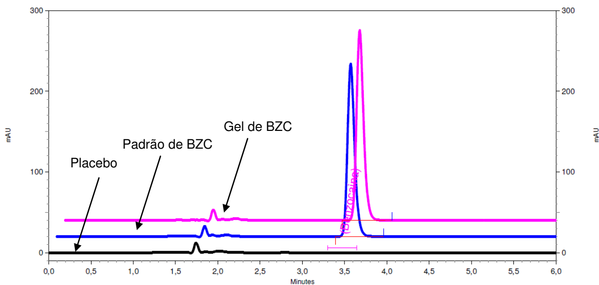
Figura 18. Cromatograma das amostras de placebo, padrão e gel de benzocaína, analisadas segundo as condições cromatográficas descritas.
