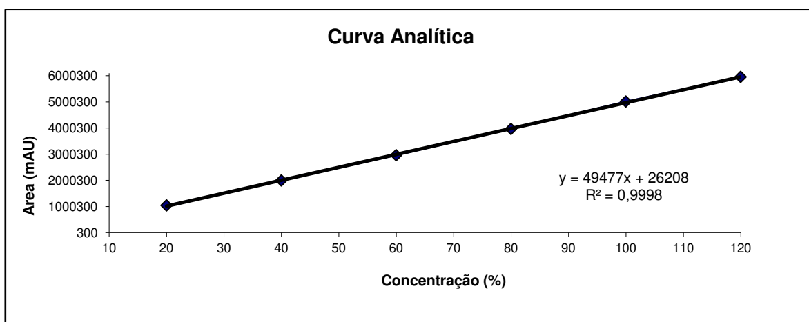
Figura 20. Curva de calibração de Benzocaína (Linearidade)
