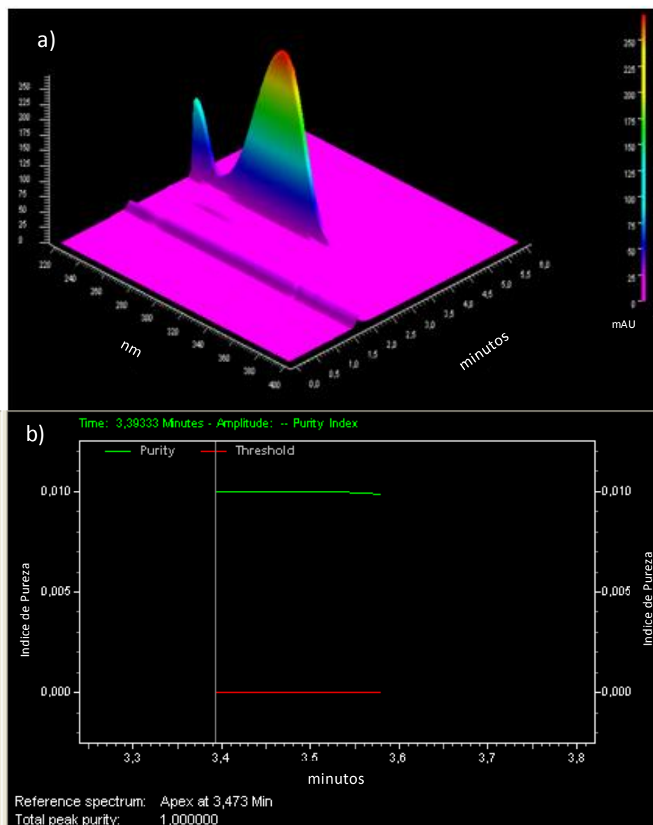
Figura 19. a) Cromatograma tridimensional (absorbância vs. tempo de retenção vs. Comprimento de onda) de uma solução de benzocaína pura. b) Gráfico de determinação de pureza de pico de benzocaína
