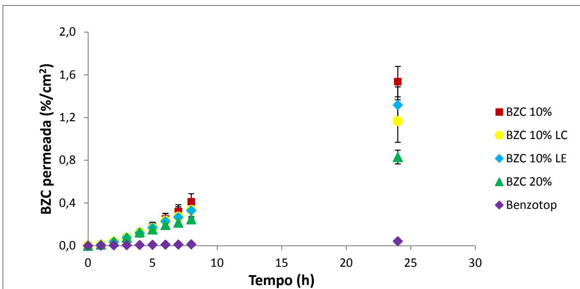
Figura 41. Perfis de liberação de benzocaína ( \text{\%}/\text{cm}^2 ) através de pele de orelha de porco a partir das formulações em gel aqui preparadas e da formulação comercial de benzocaína. Dados apresentados como média e desvio padrão ( n= 6-8 )
