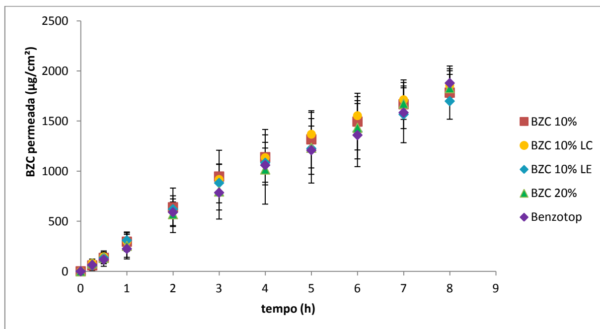
Figura 38. Perfis de liberação de benzocaína ( \mu\text{g}/\text{cm}^2 ) através de membrana artificial com poro de 30 nm a partir das formulações em gel aqui preparadas e da formulação comercial de benzocaína
