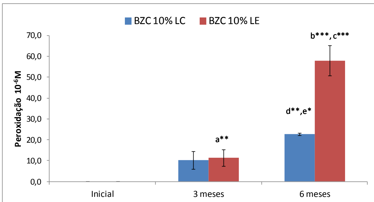
Figura 28. Teste de peroxidação lipídica pela medida de MDA ( 10^{-6}M ) em formulações em gel de benzocaína lipossomal (lipossomas convencionais e elásticos): análise inicial, após 3 e 6 meses de armazenamento a 40°C e 75% de UR). Análise estatística: ANOVA/Tukey-Kramer, p < 0,05 (*); p < 0,01 (**); p < 0,001 (***).
