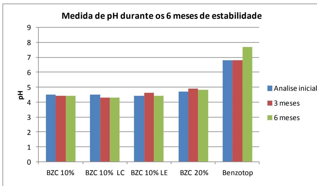
Figura 29. Média das medidas de pH das formulações em gel de benzocaína, durante 6 meses de estabilidade acelerada (40°C a 75% U.R.).
