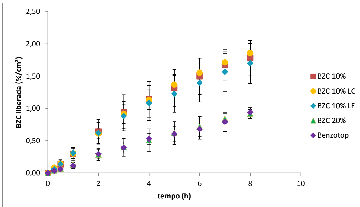
Figura 39. Perfis de liberação de benzocaína (%/cm 2 ) através de membrana artificial com poro de 30 nm a partir das formulações em gel aqui preparadas e da formulação comercial de benzocaína.
