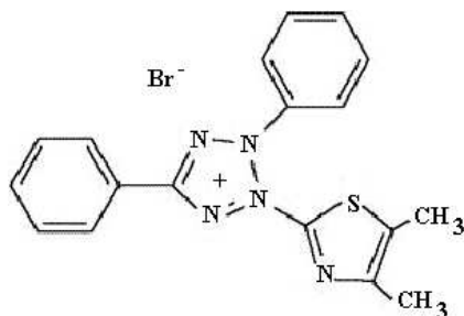
Figura 14. Estrutura química do MTT.
