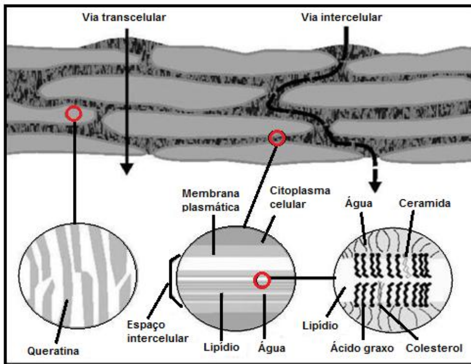
Figura 2. Representação esquemática das vias de penetração de solutos através da pele (adaptado de Gratieri et al., 2008).
