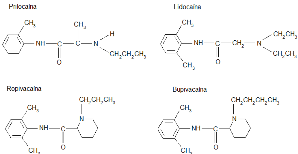
Figura 8. Estrutura química dos anestésicos locais do tipo amino-amida - prilocaína, lidocaína, ropivacaína e bupivacaína
