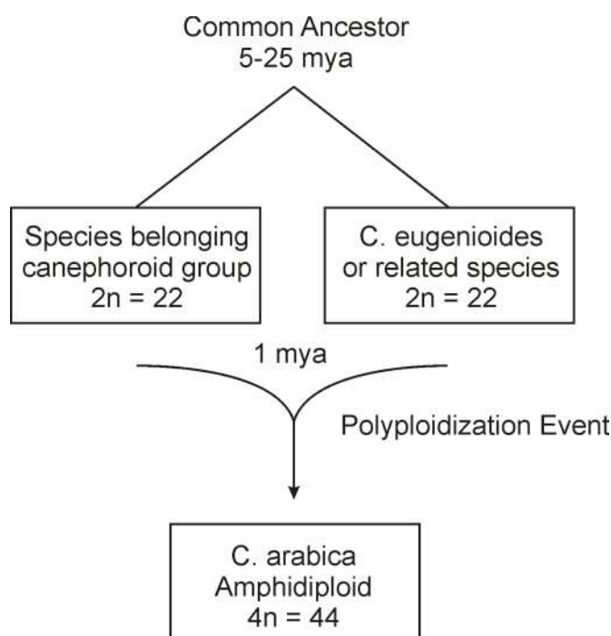
Figura 3. História evolutiva do Coffea arabica alotetraplóide. Os genomas progenitores de C. arabica estão representados pelos diplóides C. eugenioides e C. canephora . C. arabica formou-se a ~1-2 milhões de anos atrás pela fusão dessas duas espécies ou ecótipos relacionados. A divergência entre esses dois genomas é de 2,5 % em média.
