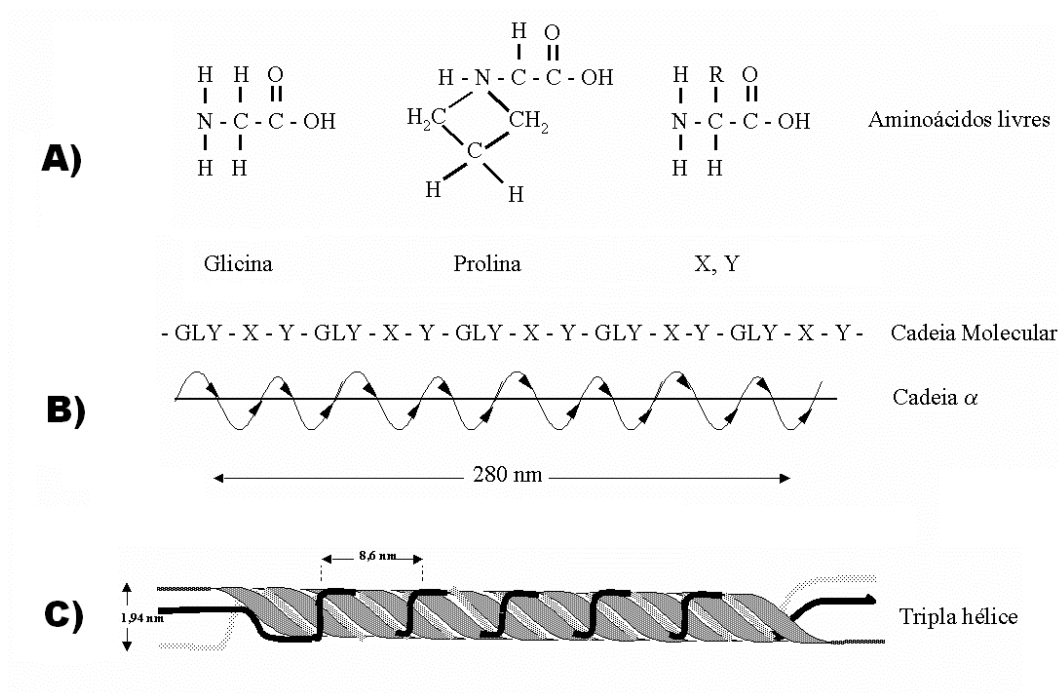
Figura 1. Diagrama da formação e estrutura do colágeno; A) fórmula estrutural dos aminoácidos mais comuns a molécula do colágeno; B) Estrutura primária da molécula do colágeno; C) Representação da estrutura secundária da molécula do colágeno, com a configuração espacial de uma tripla-hélice (Extraído e modificado de MOREIRA and AN, 2002).
