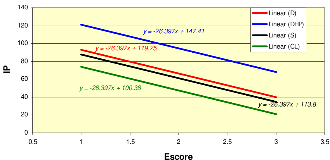
Figura 2. Modelo de regressão para o estudo de índice de permeabilidade em função do Escore com variáveis Dummy representando o efeito dos 4 tratamentos.
