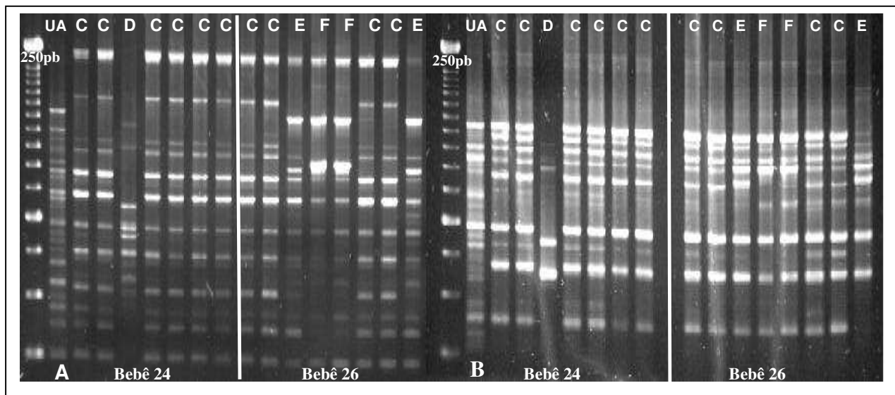
Figura 14. Gel representativo da análise de AP-PCR realizada em 15 isolados clínicos de duas crianças de 26 e 24 meses de idade com S. mutans detectáveis ambas em T18, e pertencentes à mesma EMEI. As linhas contínuas separam os isolados das crianças distintas. (A) Similaridade dos amplictipos nos isolados de dois bebês da mesma creche com o primer OPA-02 (amplictipo C , nos bebês 24 e 26). Outros perfis genotípicos diferentes foram também observados em ambas ( D , E e F ). O grau de similaridade em relação ao amplictipo C foi de 100%, podendo ser confirmada por análise com o primer arbitrário, OPA-03 (B) . UA: cepa padrão de S. mutans UA130.
