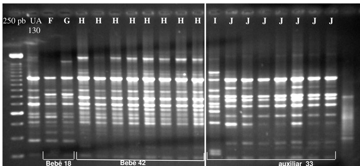
Figura 16. Gel representativo da análise de AP-PCR realizadas em 18 isolados clínicos de uma auxiliar e duas crianças de 22 meses de idade com altos níveis de S. mutans ( \geq 100 ufc) em T18, da mesma EMEI. Os diferentes amplitipos são identificados por letras acima de cada canaleta. A linha contínua separa os amplitipos da auxiliar de saúde dos amplitipos dos bebês. As letras F e G correspondem aos dois amplitipos representativos dos isolados uma criança, sendo comparado ao amplitipo H , também representativo dos isolados de outra criança da mesma creche. As letras I e J correspondem aos dois amplitipos de 8 isolados de uma cuidadora da mesma creche, entretanto, diferentes dos amplitipos da criança.
