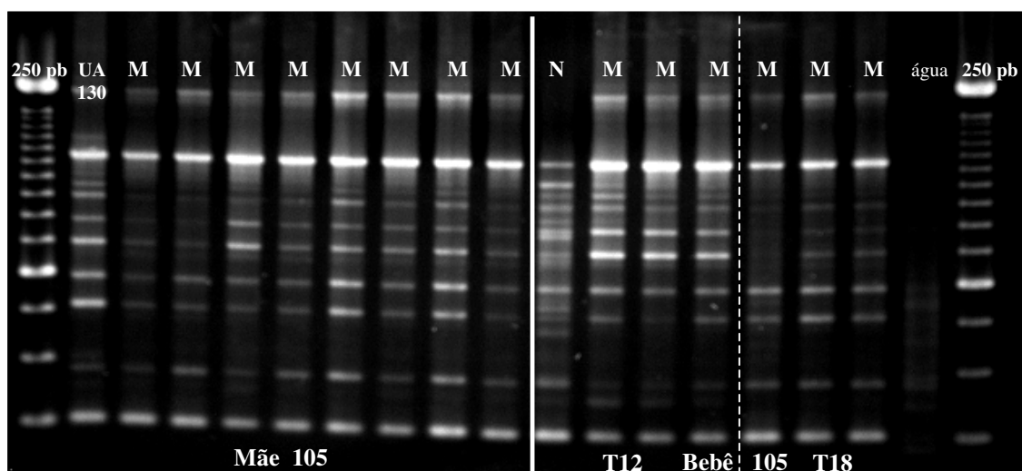
Figura 18. Gel representativo das análises de AP-PCR (OPA-02) realizadas em 8 isolados clínicos de uma mãe do sub grupo e 7 isolados representativos do filho de 30 meses de idade, em T12 e T18. Os diferentes amplictipos são identificados por letras acima de cada canaleta. A linha continua separa os isolados dos bebês dos isolados maternos, e as pontilhadas separam os dois momentos do estudo, onde o bebê foi positivo para S. mutans , com dois amplictipos detectados. A letra M representa um único amplictipo originado dos isolados da mãe, similar ao identificado na criança em dois momentos (T12 e T18). Um outro amplictipo N foi identificado em T12.
