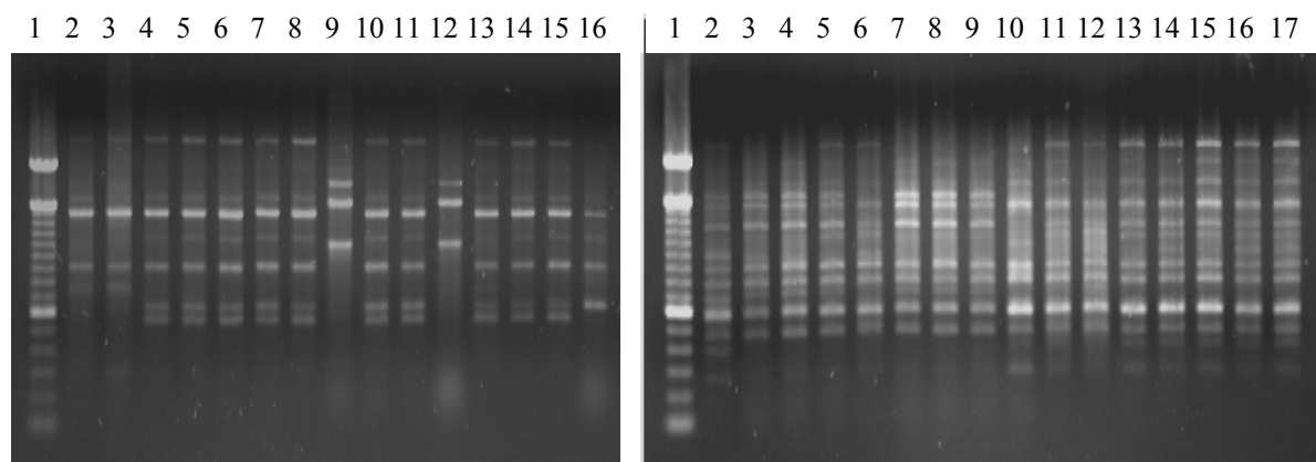
Figura 8 – Gel de AP-PCR realizado com primer OPA-13 e OPA-02 respectivamente.
