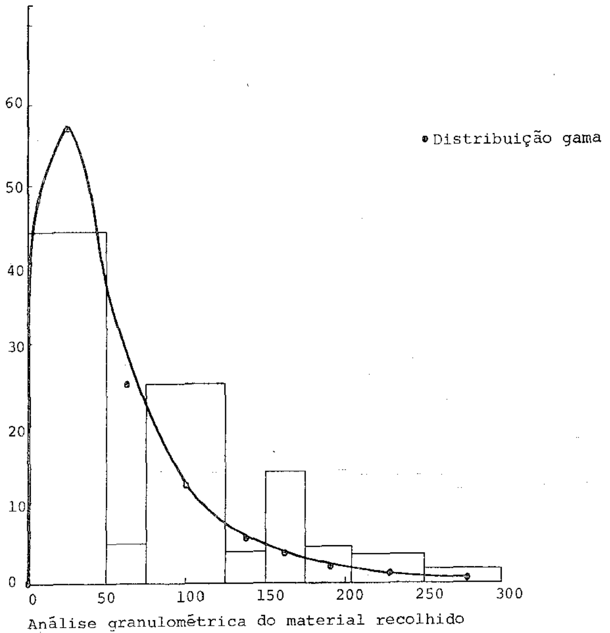
FIGURA - 33 - Hsep = 36.5 cm - Uo=3Umf
