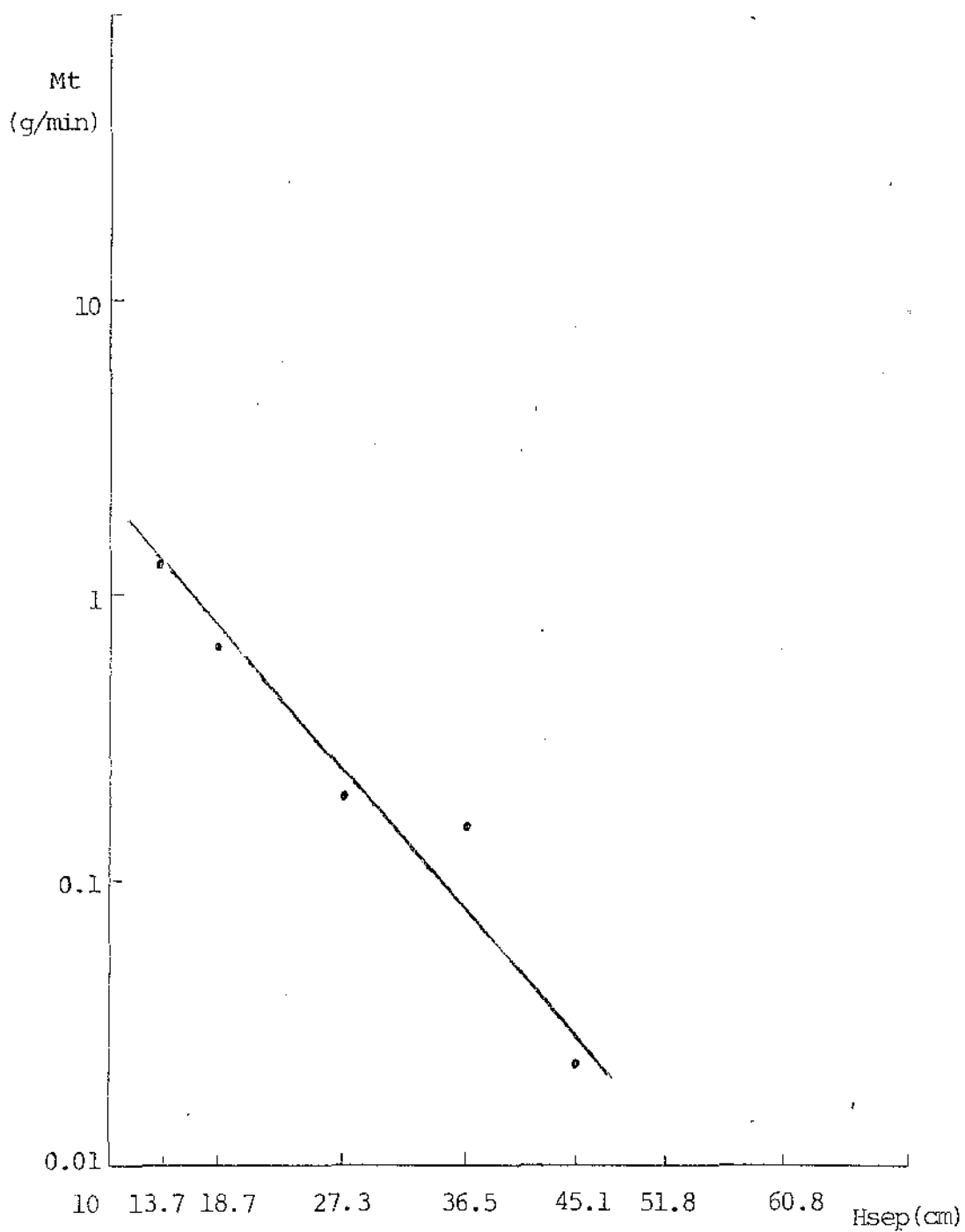
FIGURA - 11 - MASSA TRANSPORTADA VERSUS ALTURA DE SEPARAÇÃO
