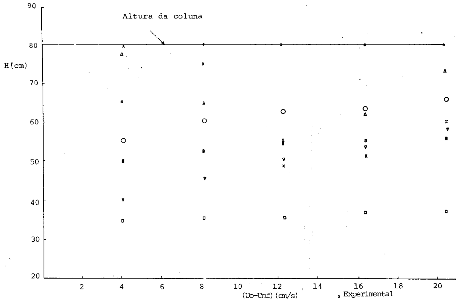
FIGURA - 46 - Gráfico de H versus ( U_o - U_{mf} )
