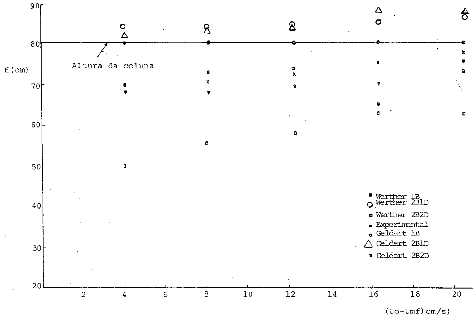
FIGURA - 44 - Gráfico de H versus (U o -U mf ) H sep =27.3cm
