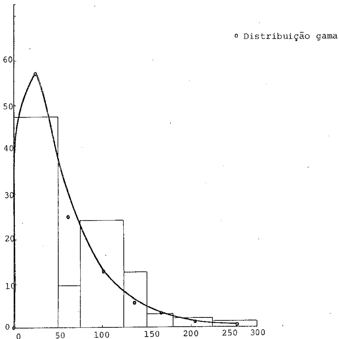
Análise granulométrica do material recolhido
