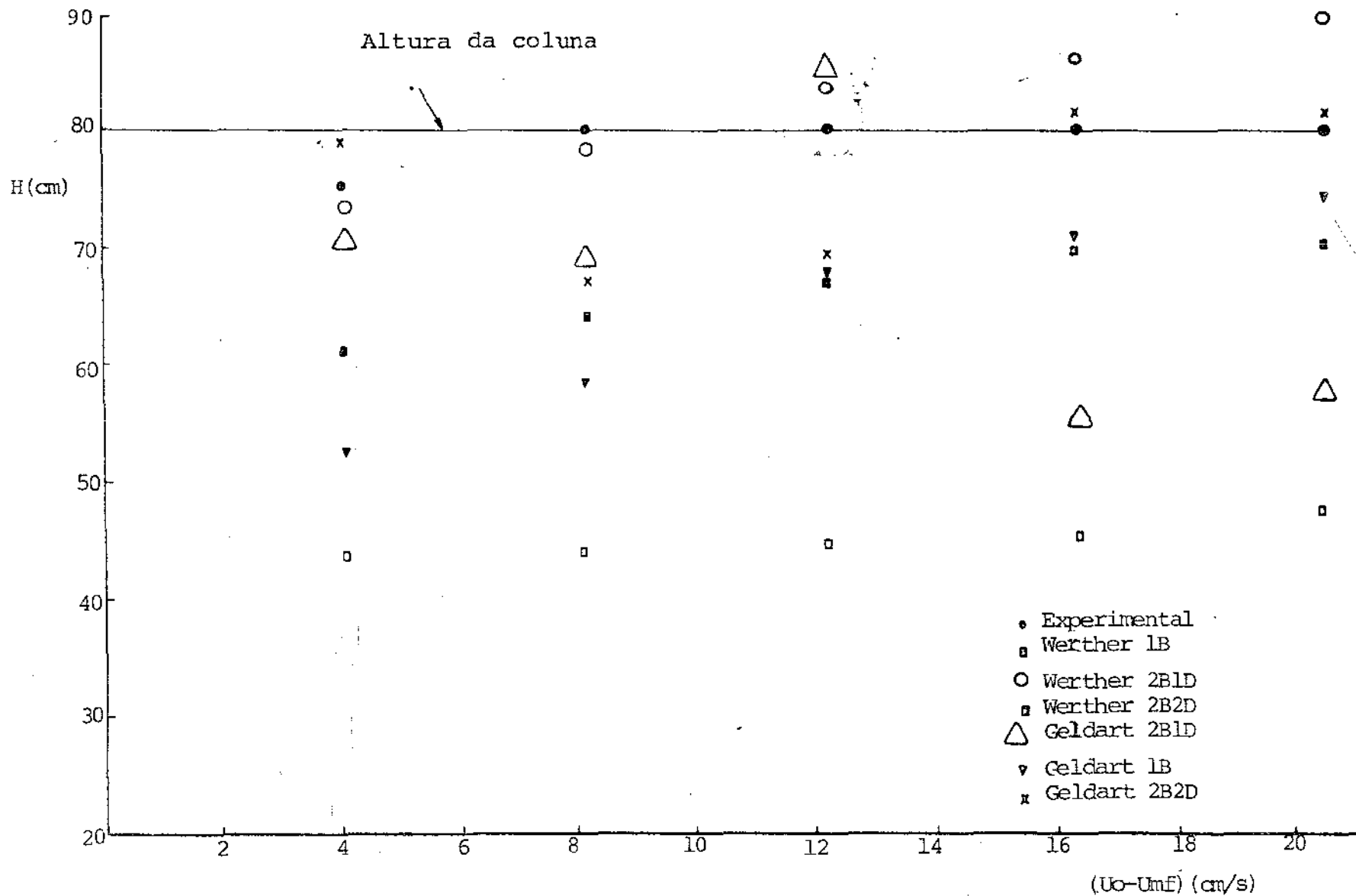
FIGURA - 45 - Gráfico de H versus (U o -U mf ) H sep =36.5cm
