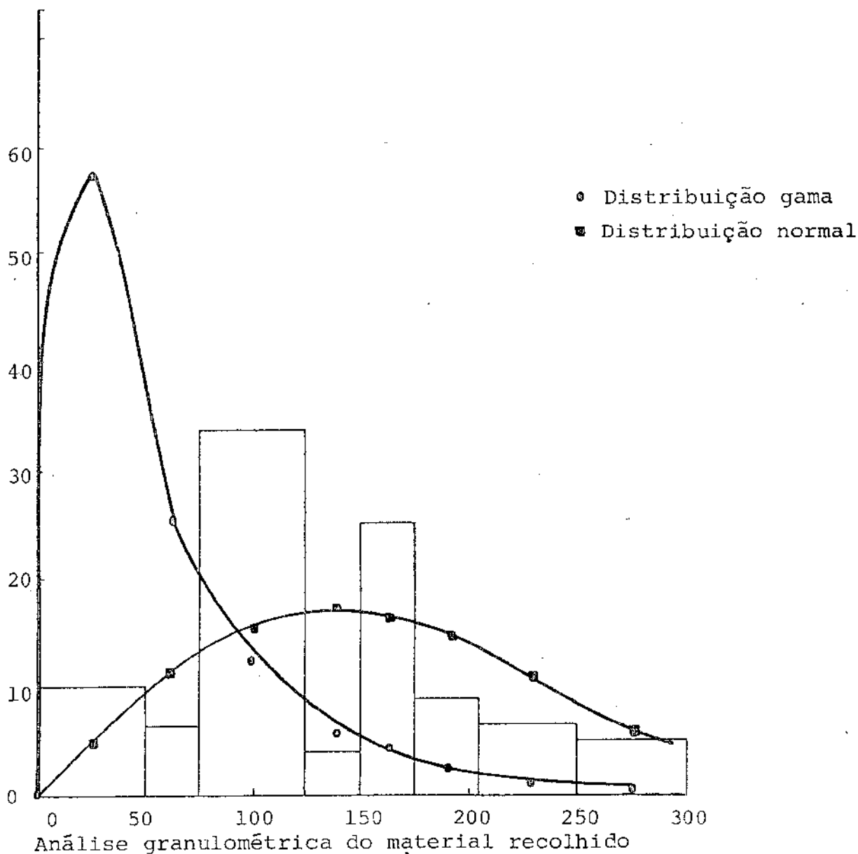
FIGURA - 36 - H_{sep} = 45.1 \text{ cm} - U_o = 6 \text{ Umf}
