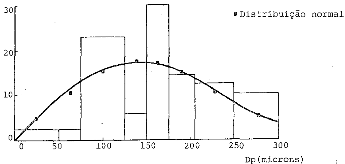
Análise granulométrica do leito
