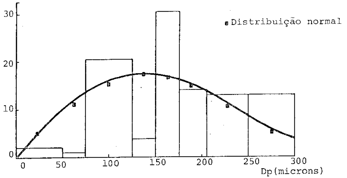
Análise granulométrica do leito
