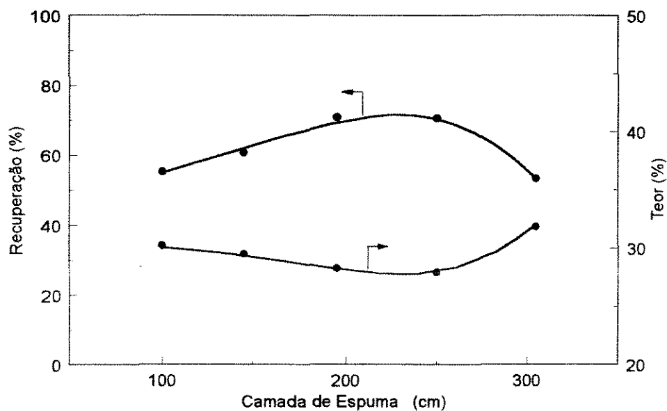
Figura V.17 - Efeito da altura da camada de espuma sobre o teor e recuperação de P_2O_5 no concentrado
