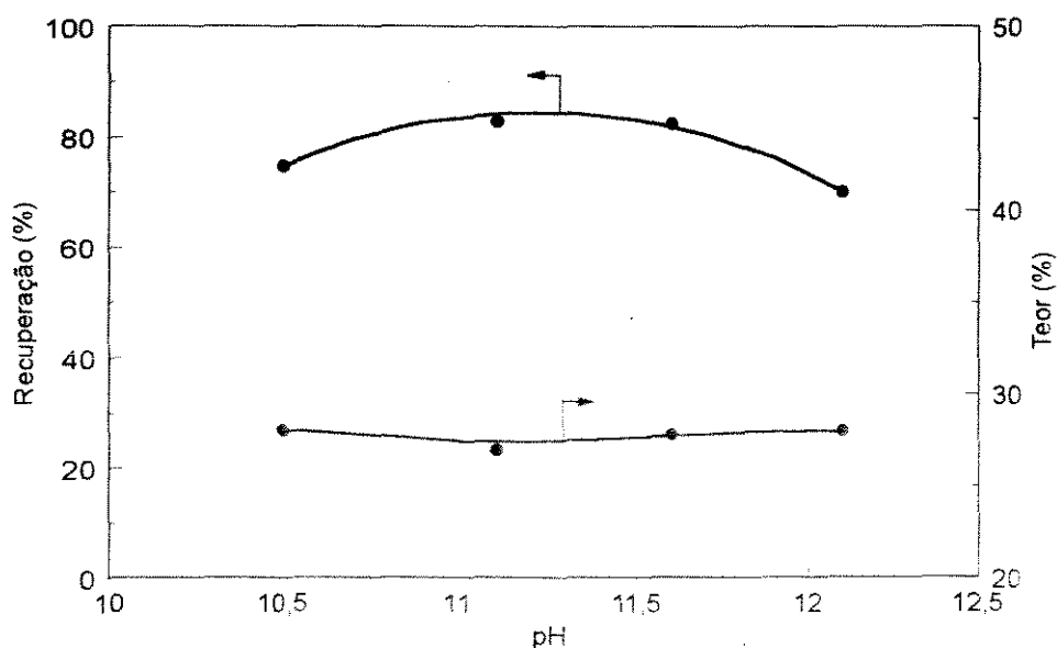
Figura V.3 - Efeito do valor do pH sobre o teor e recuperação de P_2O_5 no concentrado
