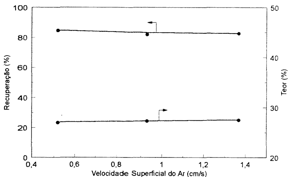
Figura V.4 - Efeito da velocidade superficial do ar sobre o teor e recuperação de P_2O_5 no concentrado
