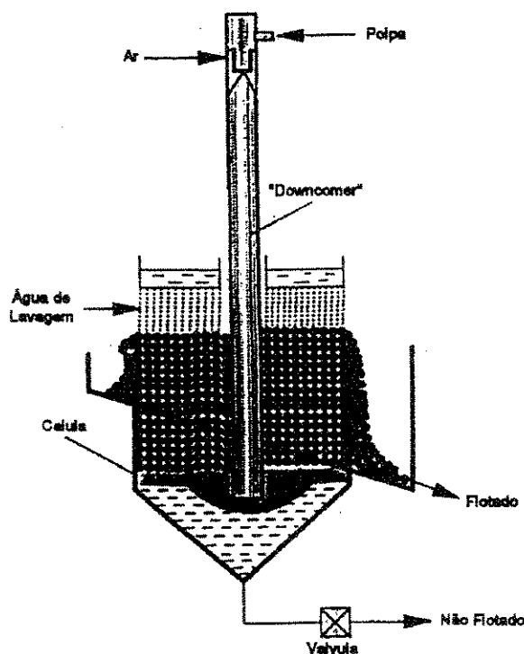
Figura II.15 – Desenho esquemático da célula Jameson
