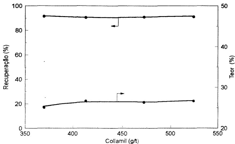
Figura VI.3 - Efeito da dosagem do collamil sobre o teor e recuperação de P_2O_5 no concentrado
