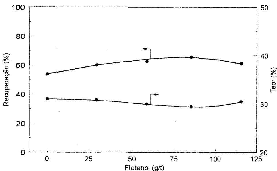
Figura V.15 - Efeito da dosagem de Flotanol sobre o teor e recuperação de P_2O_5 no concentrado
