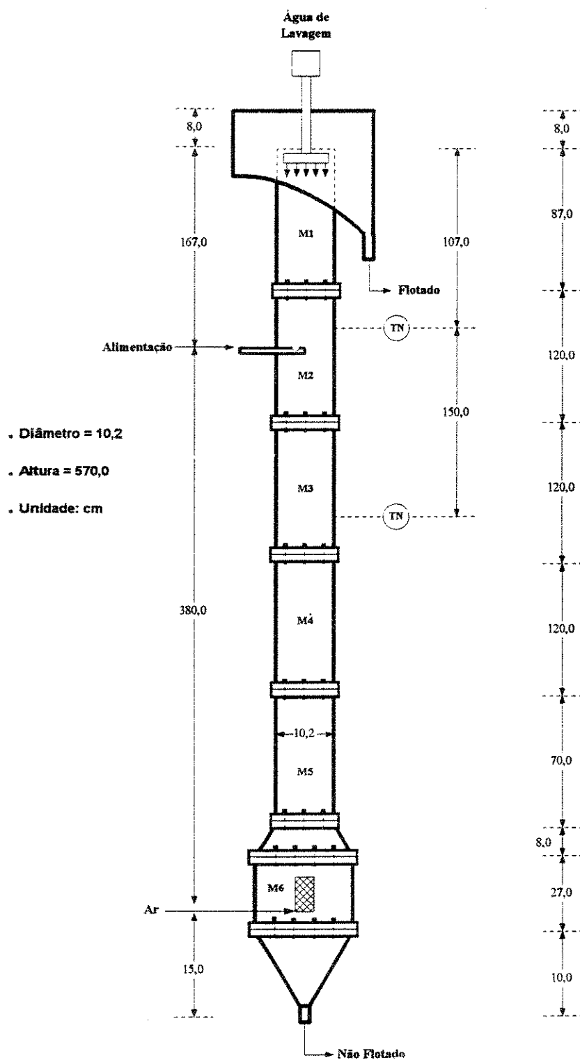
Figura III.4 - Desenho esquemático da coluna convencional
