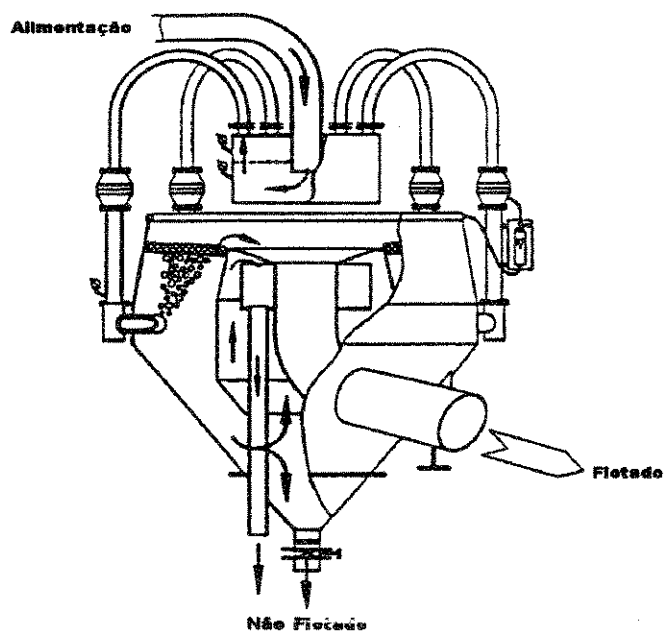
Figura II.9 - Alimentação da polpa na célula Bahr no sentido horizontal
