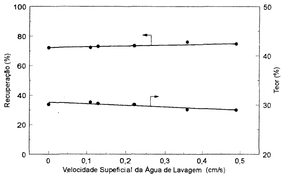
Figura V.18 - Efeito da velocidade superficial da água de lavagem sobre o teor e recuperação de P_2O_5 no concentrado
