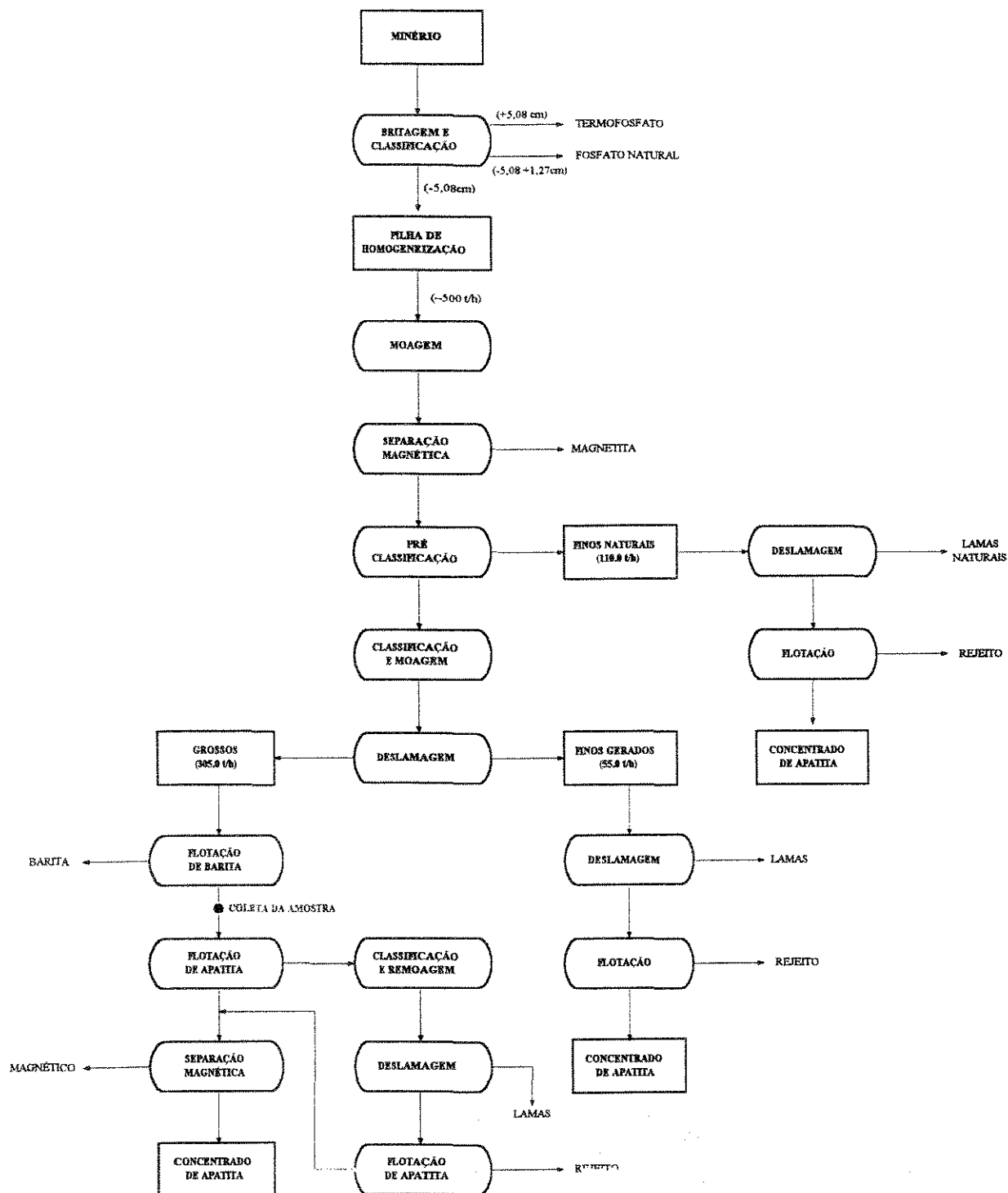
Figura III.1 – Fluxograma de blocos do circuito industrial da Arafertil
