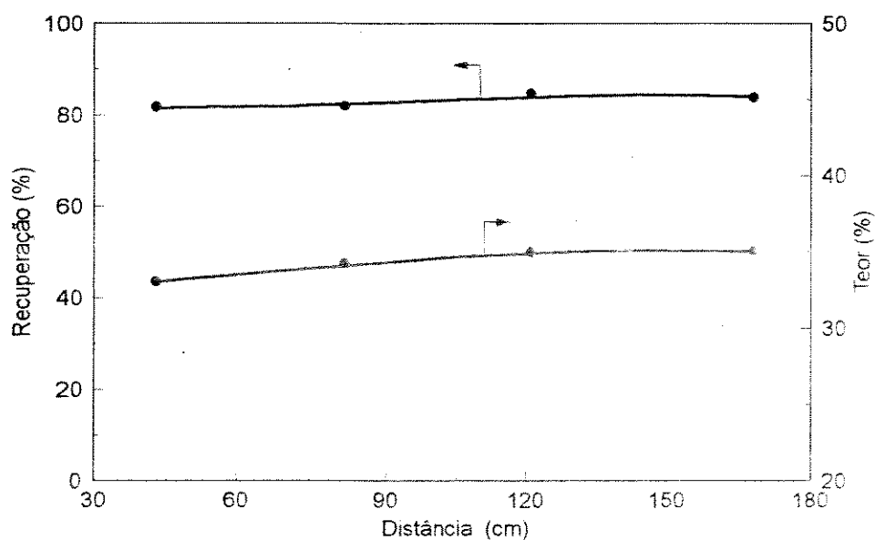
Figura VI.15 – Efeito da altura do ponto de alimentação da polpa sobre o teor e recuperação de P_2O_5 no concentrado
