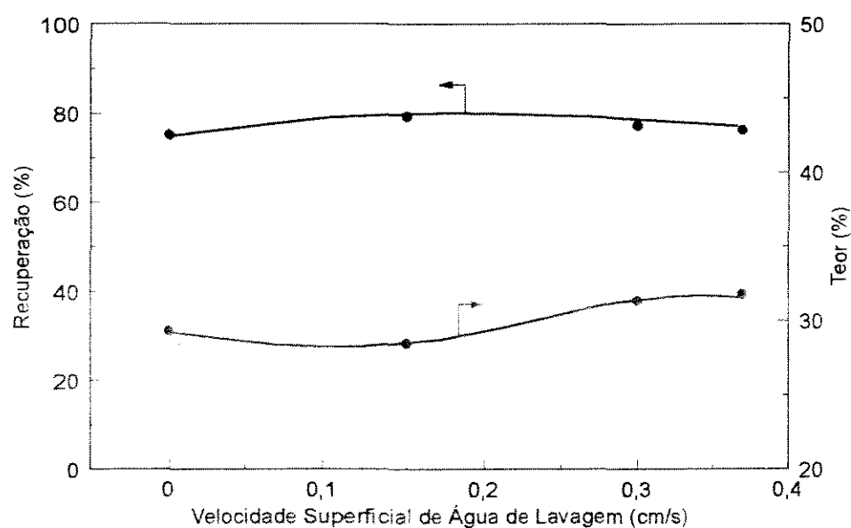
Figura V.8 - Efeito da velocidade superficial da água de lavagem sobre o teor e recuperação de \text{P}_2\text{O}_5 no concentrado
