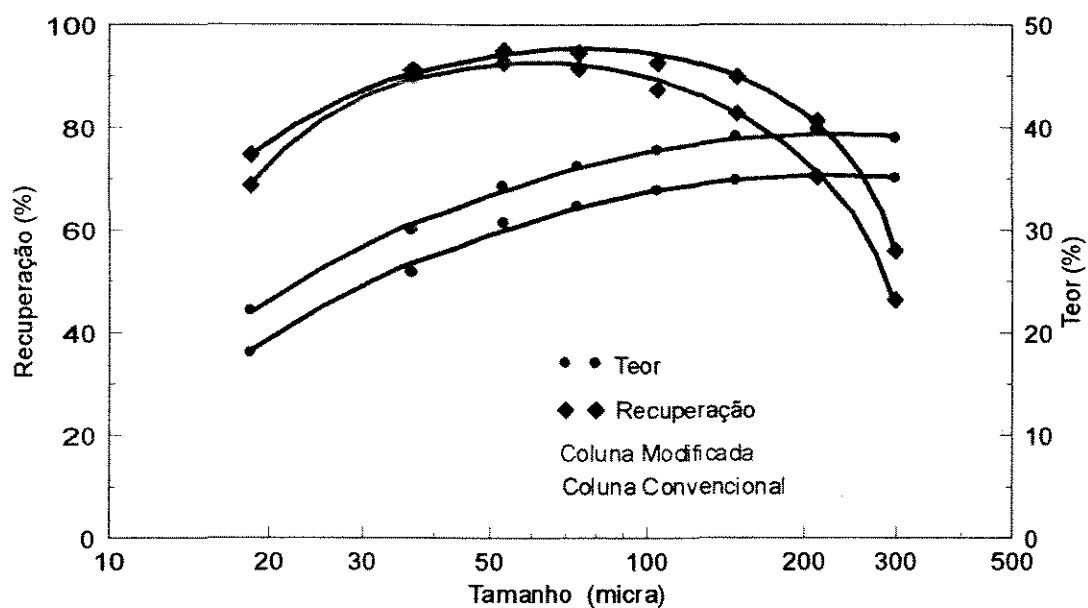
Figura VI.19 – Recuperação e teor de P_2O_5 no concentrado em função do tamanho de partícula
