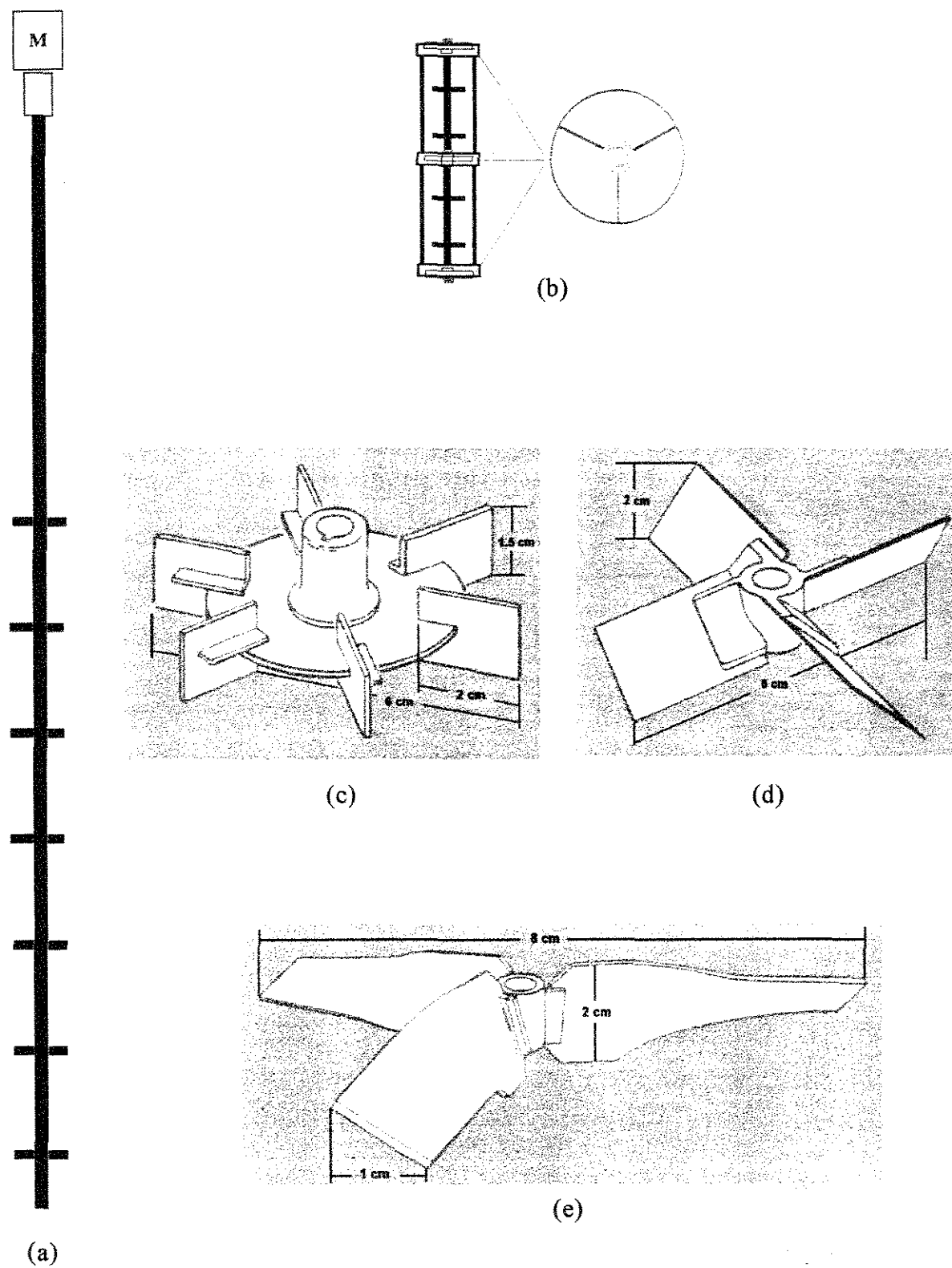
Figura III.6 – Detalhes do sistema de agitação.
