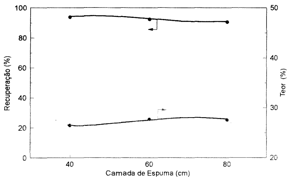
Figura VI.5 - Efeito da altura da camada de espuma sobre o teor e recuperação de P_2O_5 no concentrado
