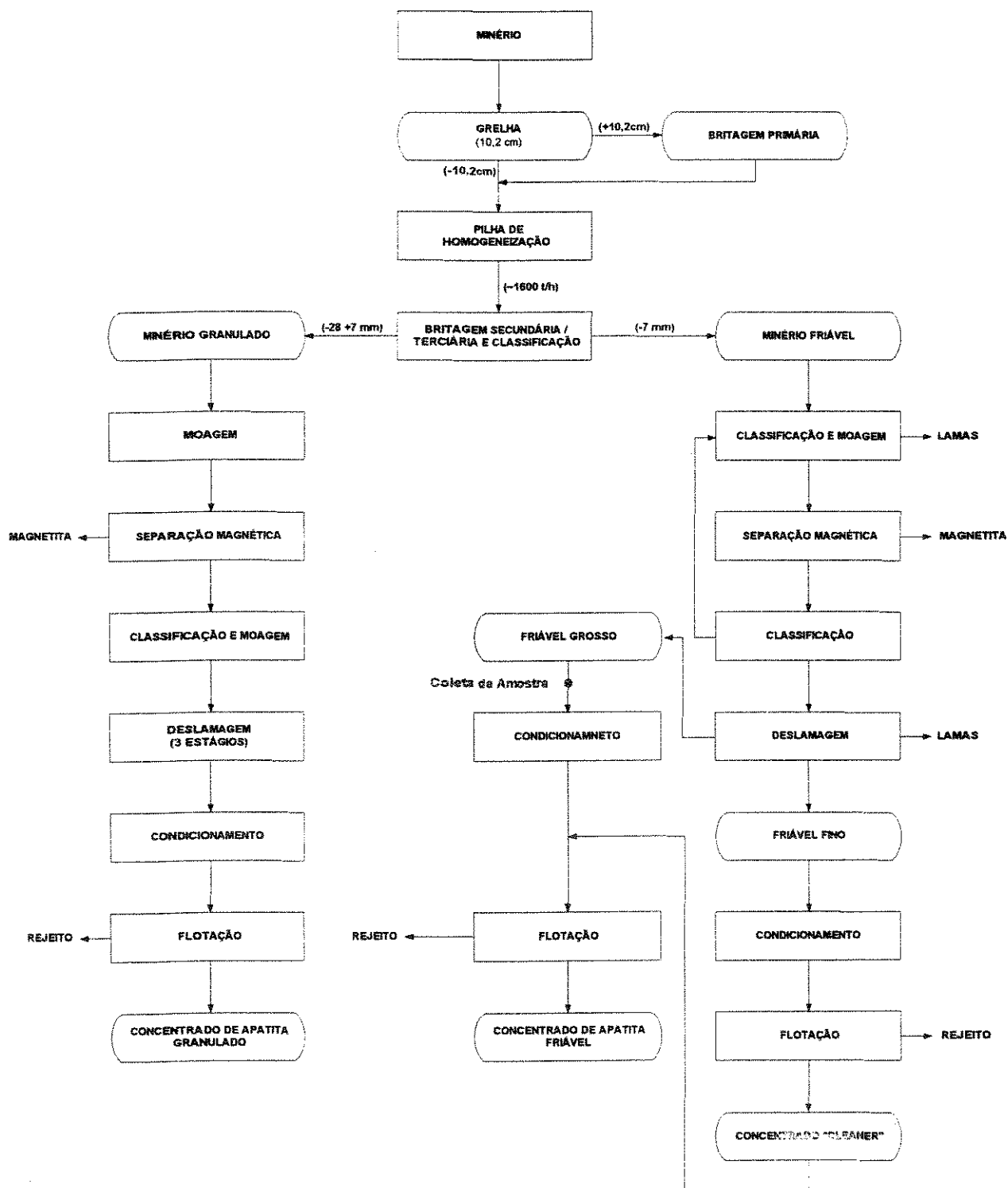
Figura III.2 - Fluxograma de blocos do circuito industrial da Fosfertil
