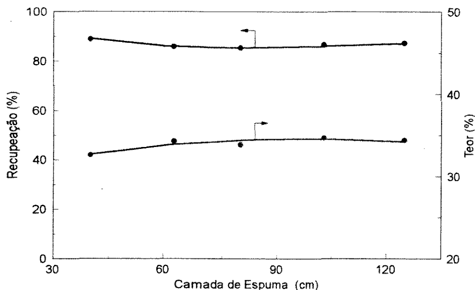
Figura VI.14 – Efeito da altura da camada de espuma sobre o teor e recuperação de P_2O_5 no concentrado
