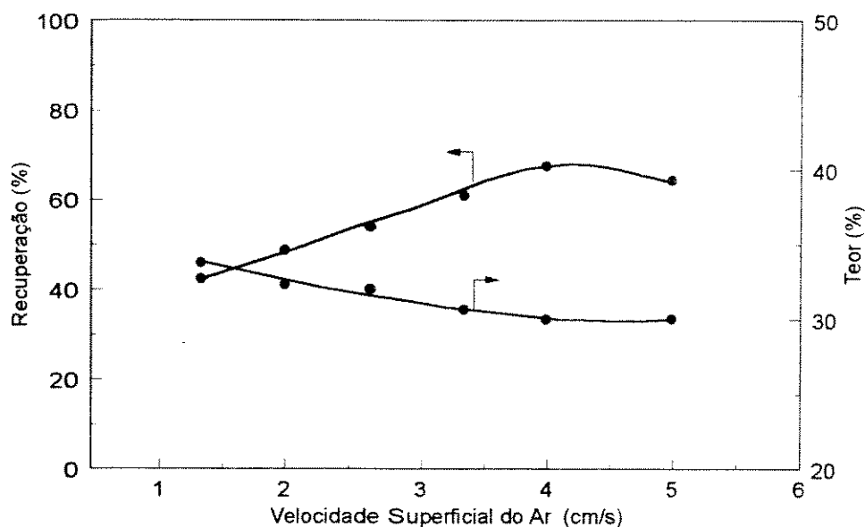
Figura V.16 - Efeito da velocidade superficial do ar sobre o teor e recuperação de P_2O_5 no concentrado
