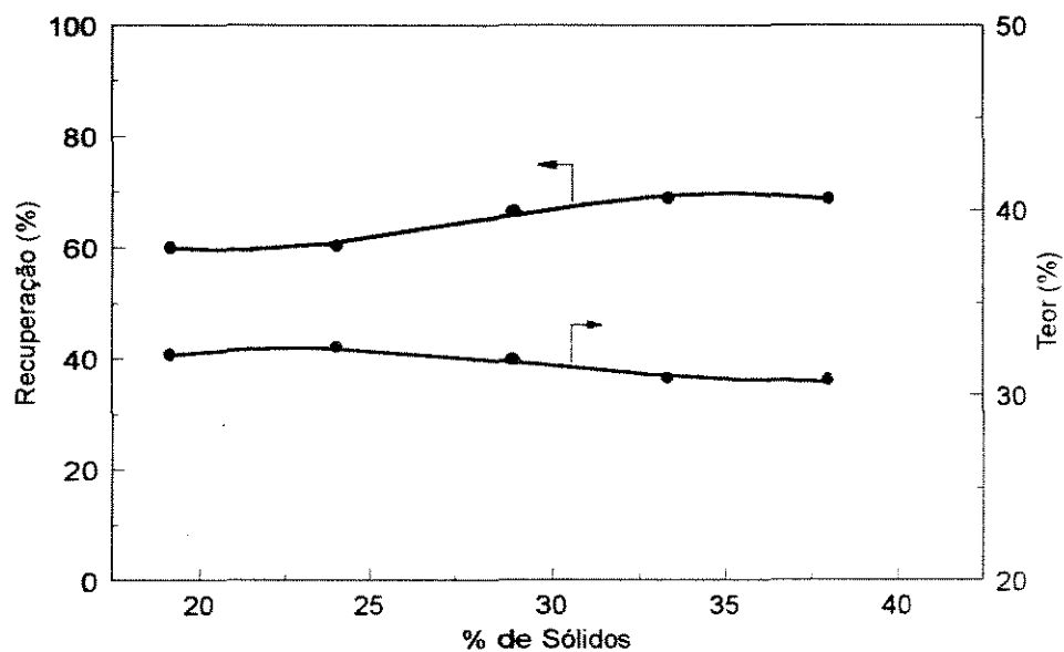
Figura V.19 - Efeito da concentração de sólidos sobre o teor e recuperação de P_2O_5 no concentrado
