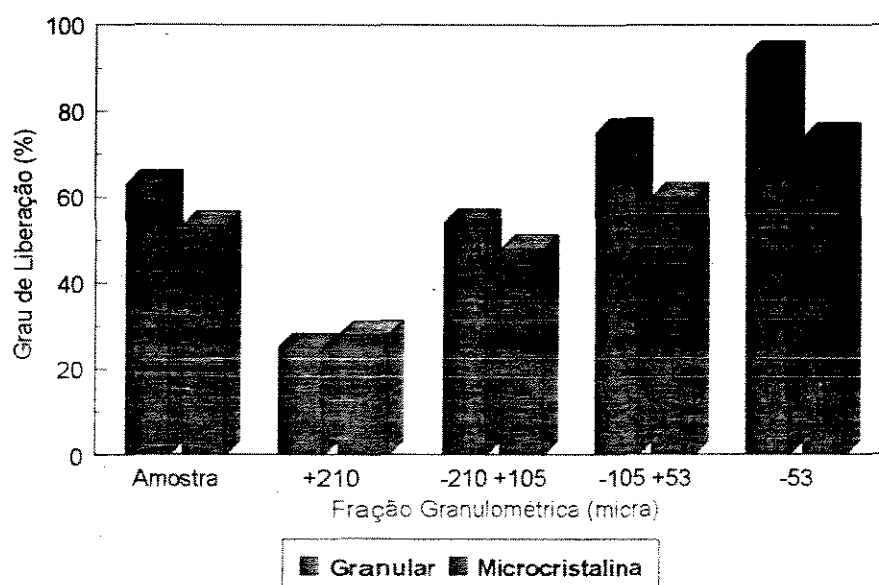
Figura IV.10 - Representação gráfica do grau de liberação da apatita granular e microcristalina da Arafertil
