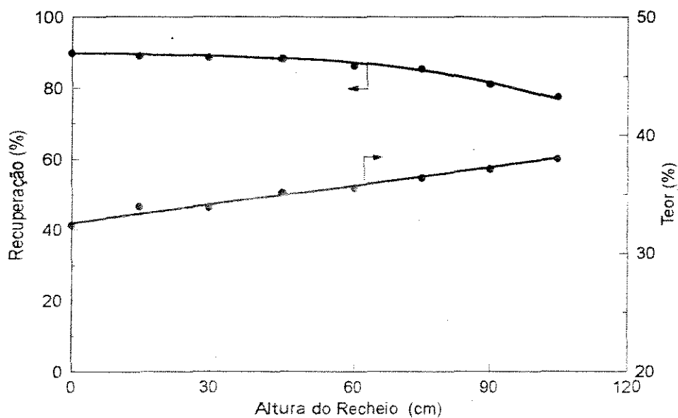
Figura VI.13 – Efeito da altura de recheio sobre o teor e recuperação de P_2O_5 no concentrado
