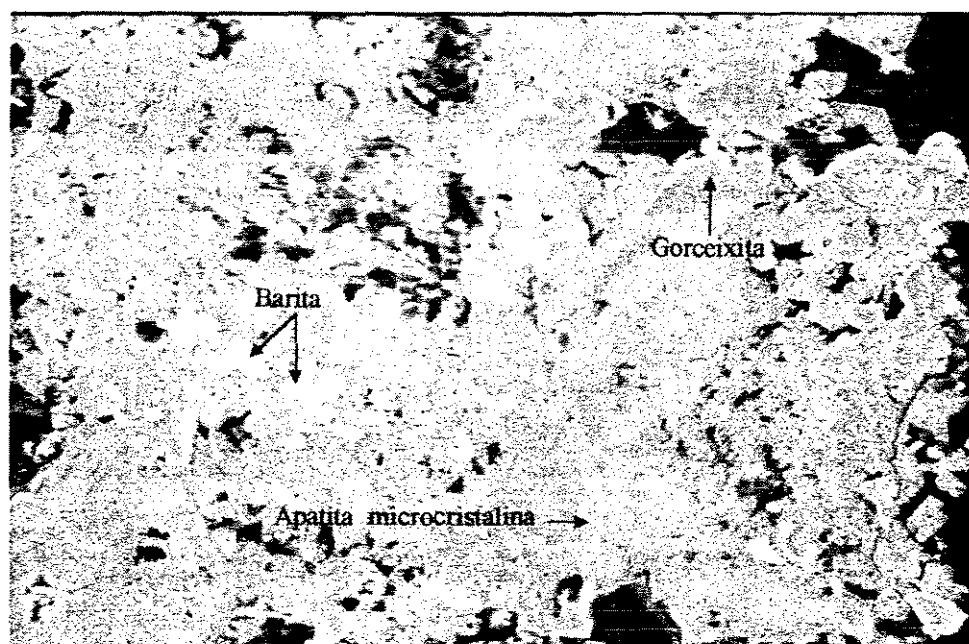
Figura IV.8 – Imagem de elétrons retroespalhados, obtida em microscópio eletrônico de varredura, mostrando apatita granular alterada à gorceixita e apatita microcristalina
