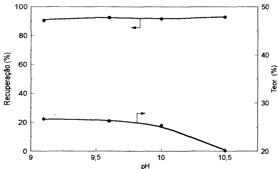
Figura VI.4 - Efeito do pH sobre o teor e recuperação de P_2O_5 no concentrado
