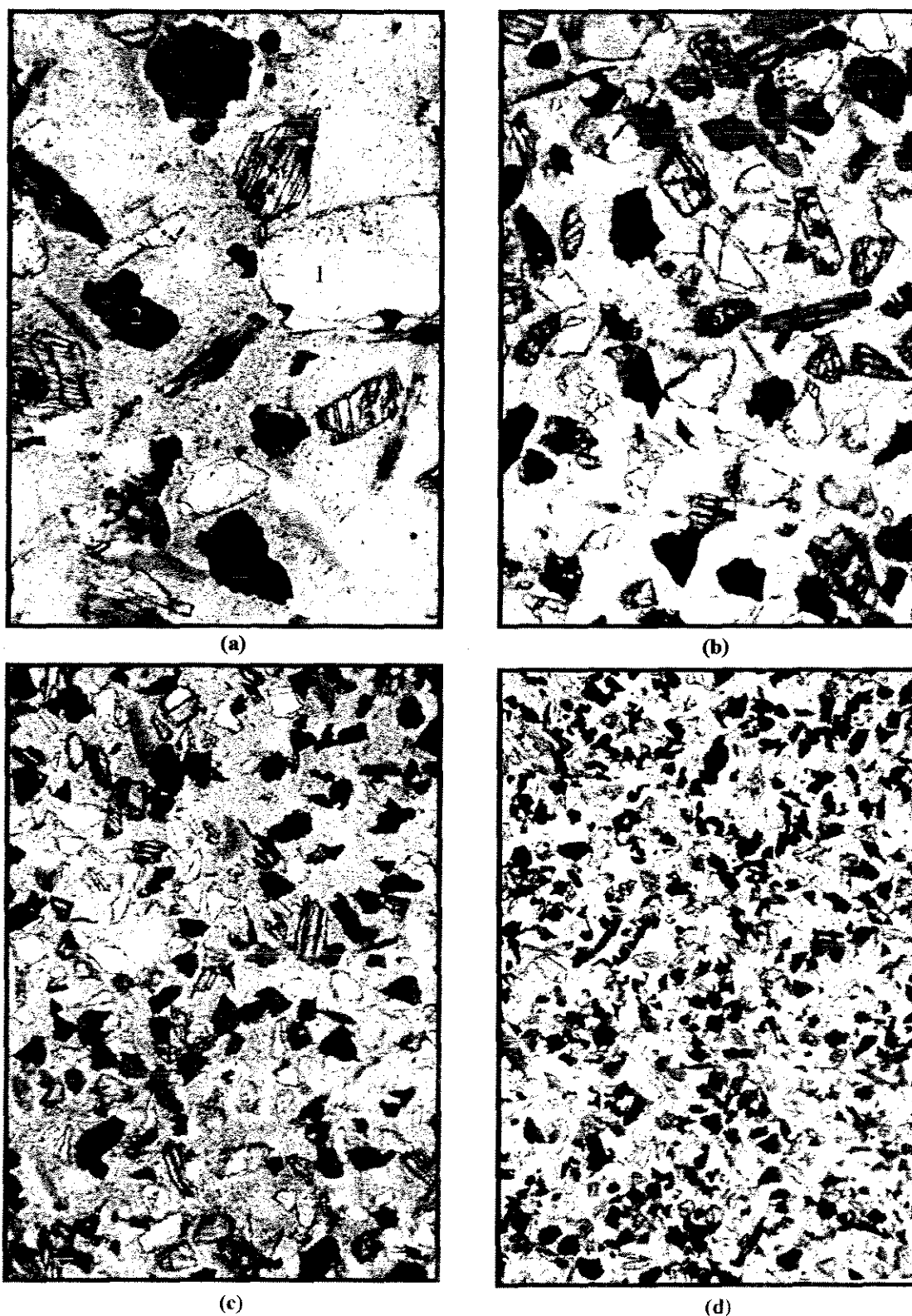
Figura IV.13 – Fotomicrografias do minério apatítico da Fosfertil nas frações granulométricas: (a) + 210; (b) - 210 + 149; (c) - 149 + 74 e (d) - 74 \mu\text{m} . Minerais identificados: apatita (1); opacos (2); vermiculita (3); piroxênio (4) e minerais de titânio (5)
