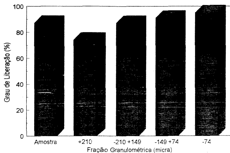
Figura IV.18 - Representação gráfica do grau de liberação da apatita da Fosfertil
