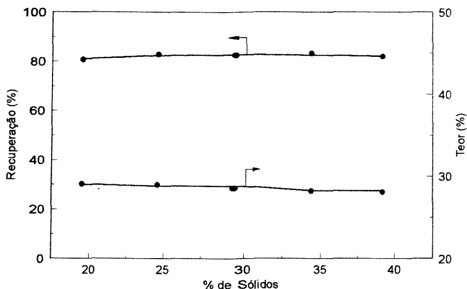
Figura V.7 - Efeito da concentração de sólidos sobre o teor e recuperação de P_2O_5 no concentrado
