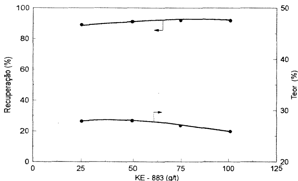
Figura VI.2 - Efeito da dosagem de KE - 883 sobre o teor e recuperação de P_2O_5 no concentrado.
