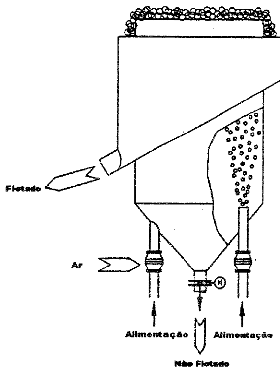
Figura II.8 – Alimentação da polpa na célula Bahr no sentido vertical
