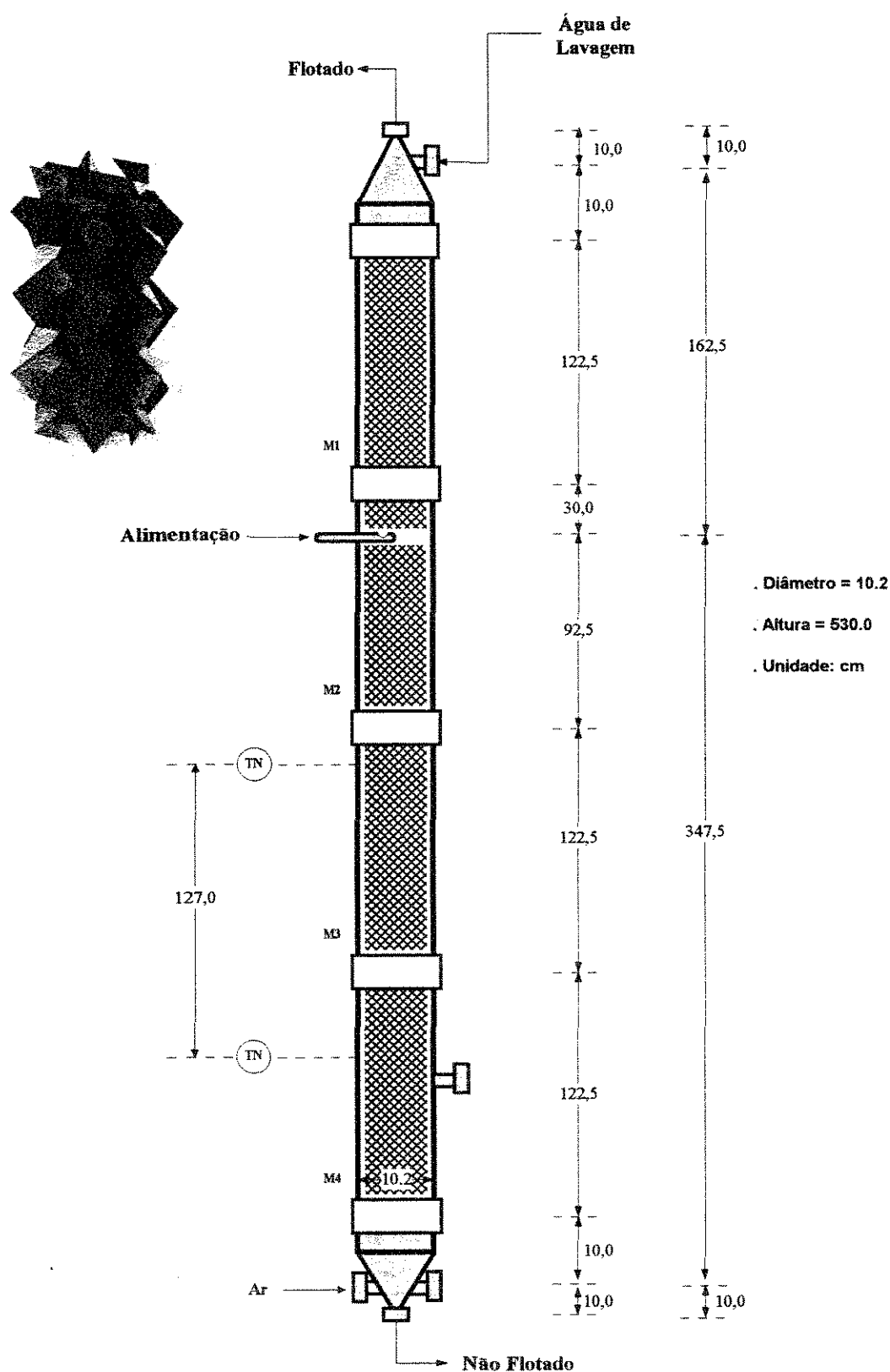
Figura III.7 - Desenho esquemático da coluna de recheio
