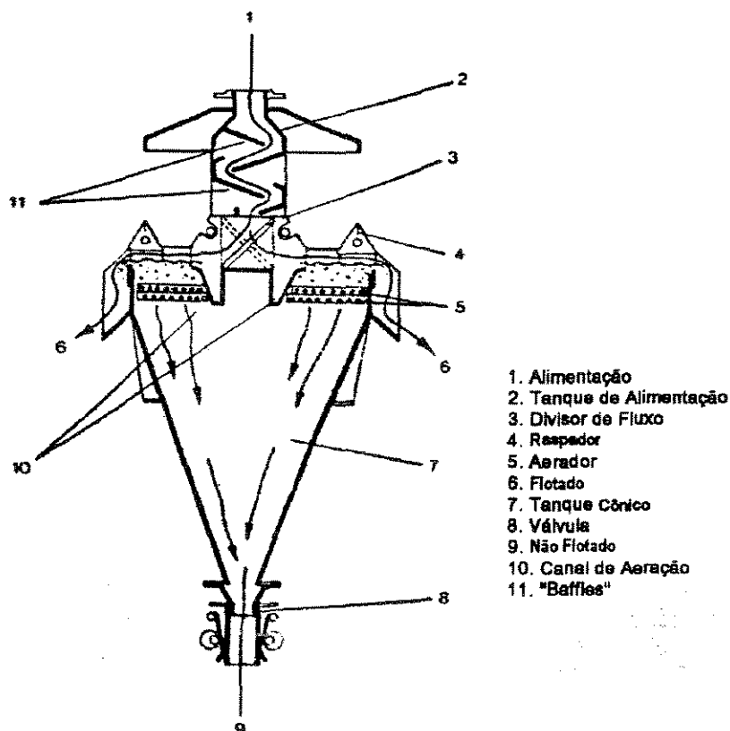
Figura II.10 – Desenho esquemático do separador de espuma
