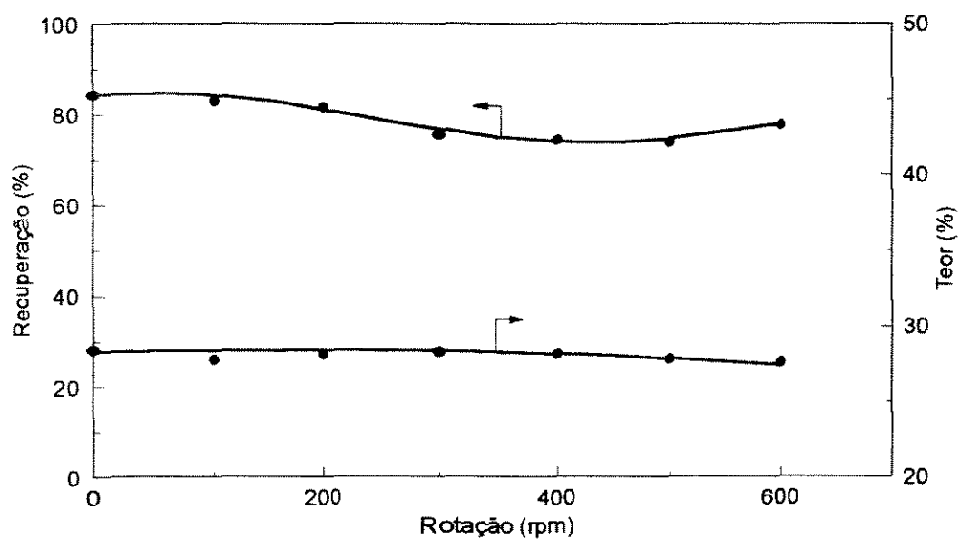
Figura V.10 - Efeito da rotação sobre o teor e recuperação de P_2O_5 no concentrado (número de hélices = 3)
