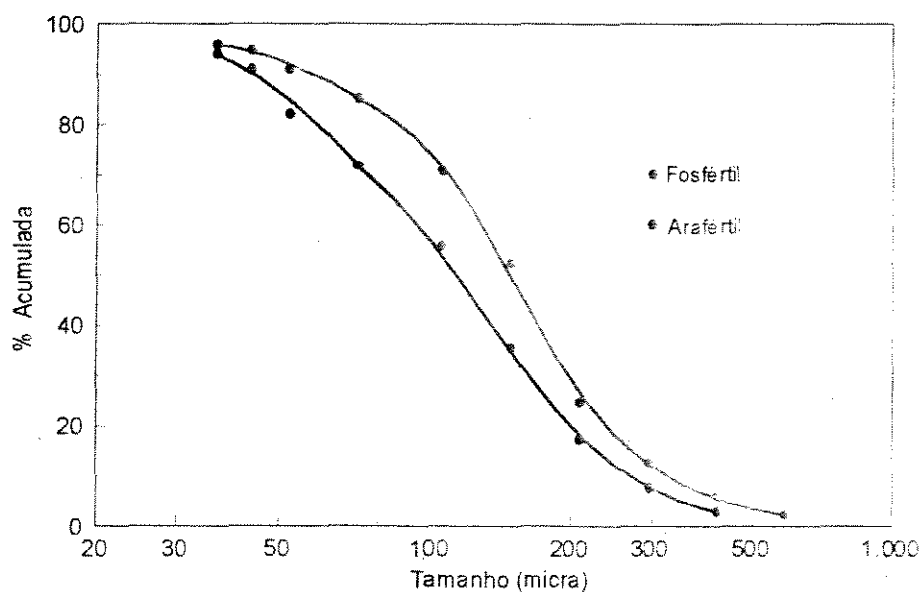
Figura IV.1 - Distribuição granulométrica acumulada das amostras da Arafertil e Fosfertil
