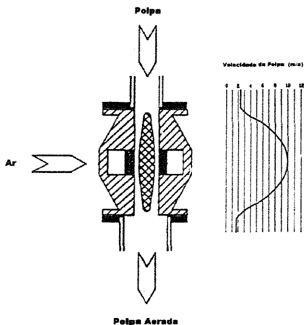
Figura II.7 – Sistema de contato partícula-bolha e a curva de velocidade da polpa
