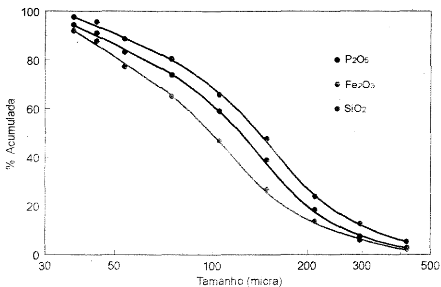
Figura IV.2 – Distribuição de P_2O_5 , Fe_2O_3 e SiO_2 nas frações granulométricas da amostra da Arafertil
