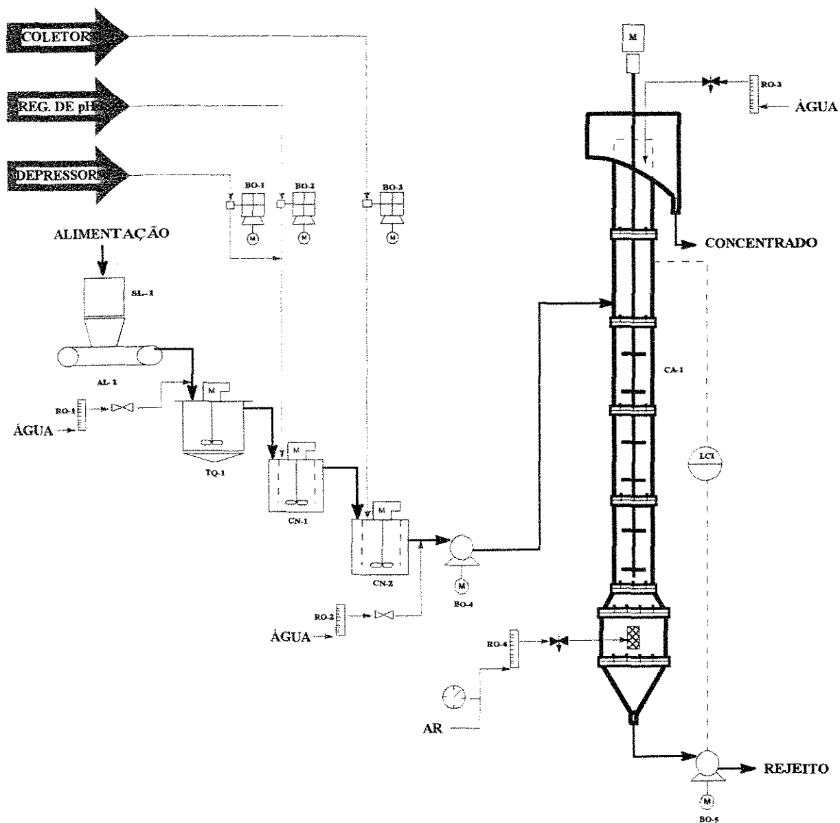
Figura III.10 - Fluxograma do circuito utilizando a coluna agitada
