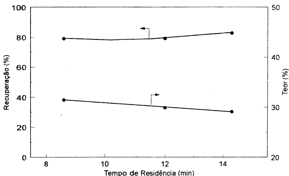
Figura V.5 - Efeito do tempo de residência sobre o teor e recuperação de P_2O_5 no concentrado
