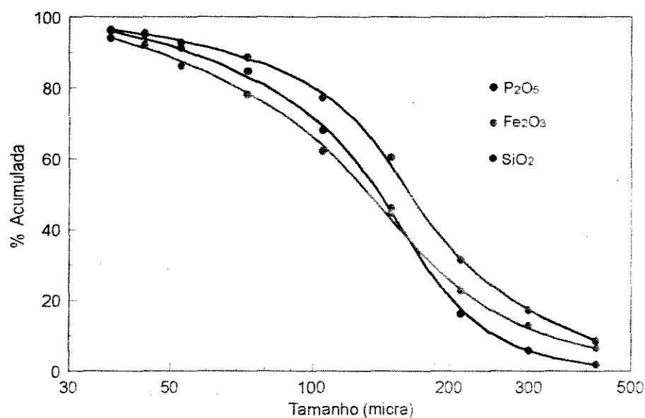
Figura IV.3 – Distribuição de P_2O_5 , Fe_2O_3 e SiO_2 nas frações granulométricas da amostra da Fosfertil
