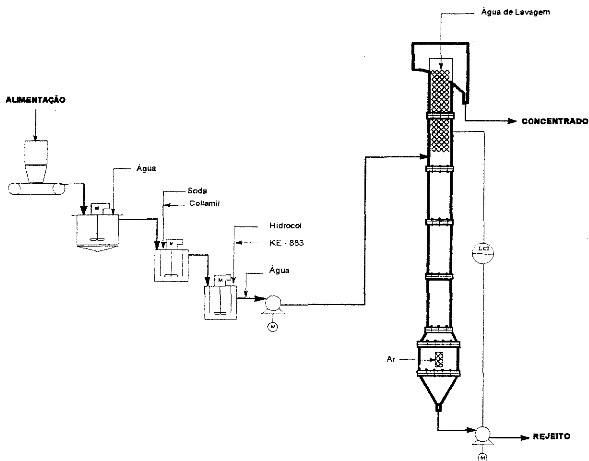
Figura VI.12 – Fluxograma do circuito utilizado nos testes com a coluna modificada
