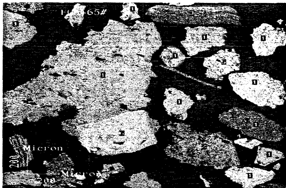
Figura IV.11 – Imagem de elétrons retroespalhados da amostra FGA + 210 µm, obtida via microscópio eletrônico de varredura, mostrando apatita (1), quartzo com inclusões de óxido de ferro (2), clorita (3), barita (4), partícula mista de apatita com óxido de ferro (5) e magnetita (6) parcialmente incluída na apatita.
