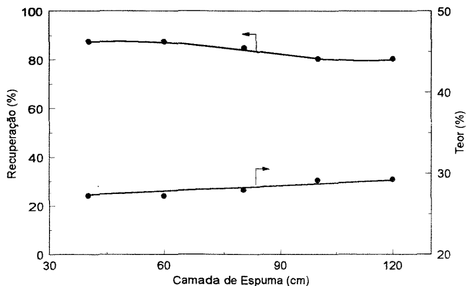
Figura V.6 - Efeito da altura da camada de espuma sobre o teor e recuperação de P_2O_5 no concentrado
