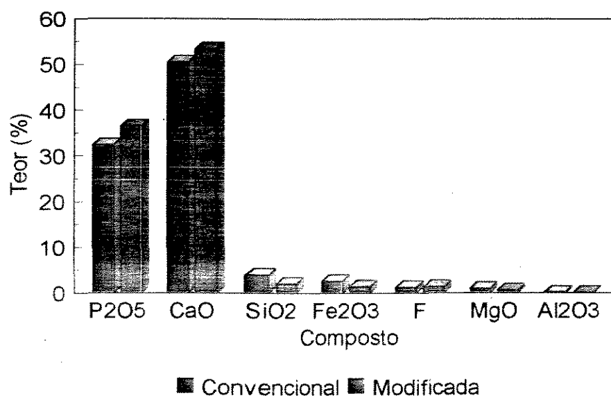
Figura VI.18 – Representação gráfica dos teores obtidos nos concentrados das colunas convencional e modificada
