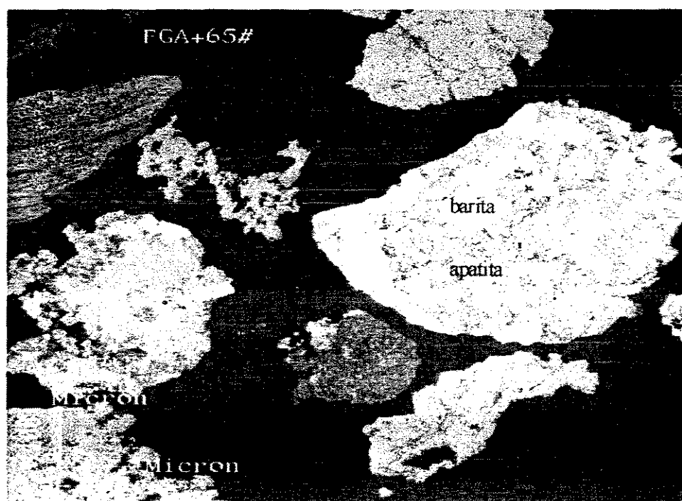
Figura IV.9 – Imagem de elétrons retroespalhados obtida em microscópio eletrônico de varredura, mostrando detalhe da apatita associada com barita
