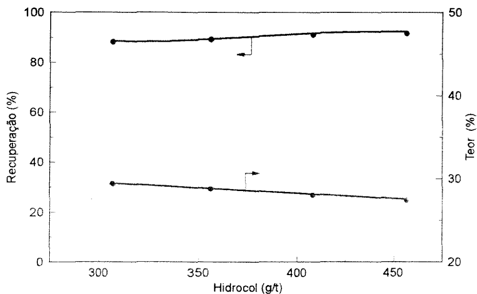
Figura VI.1 - Efeito da dosagem do hidrocol sobre o teor e recuperação de P_2O_5 no concentrado
