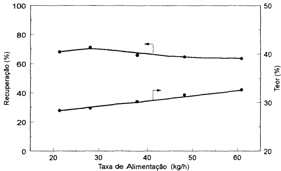
Figura V.20 - Efeito da taxa de alimentação sobre o teor e recuperação de P_2O_5 no concentrado
