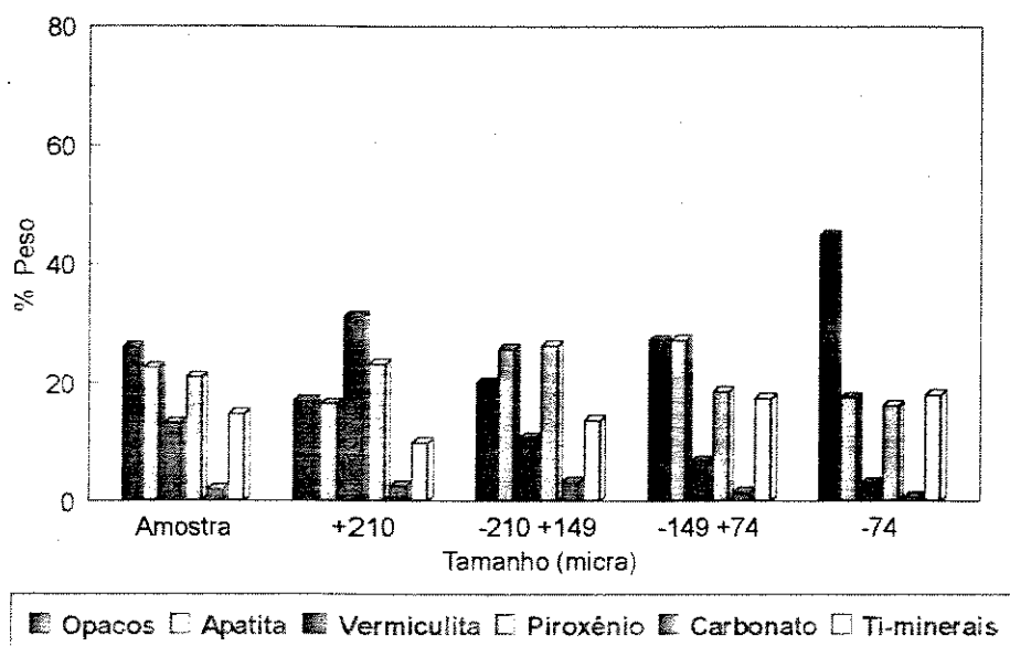
Figura IV.12 – Representação gráfica da composição mineralógica da amostra da Fosfertil e de suas frações granulométricas
