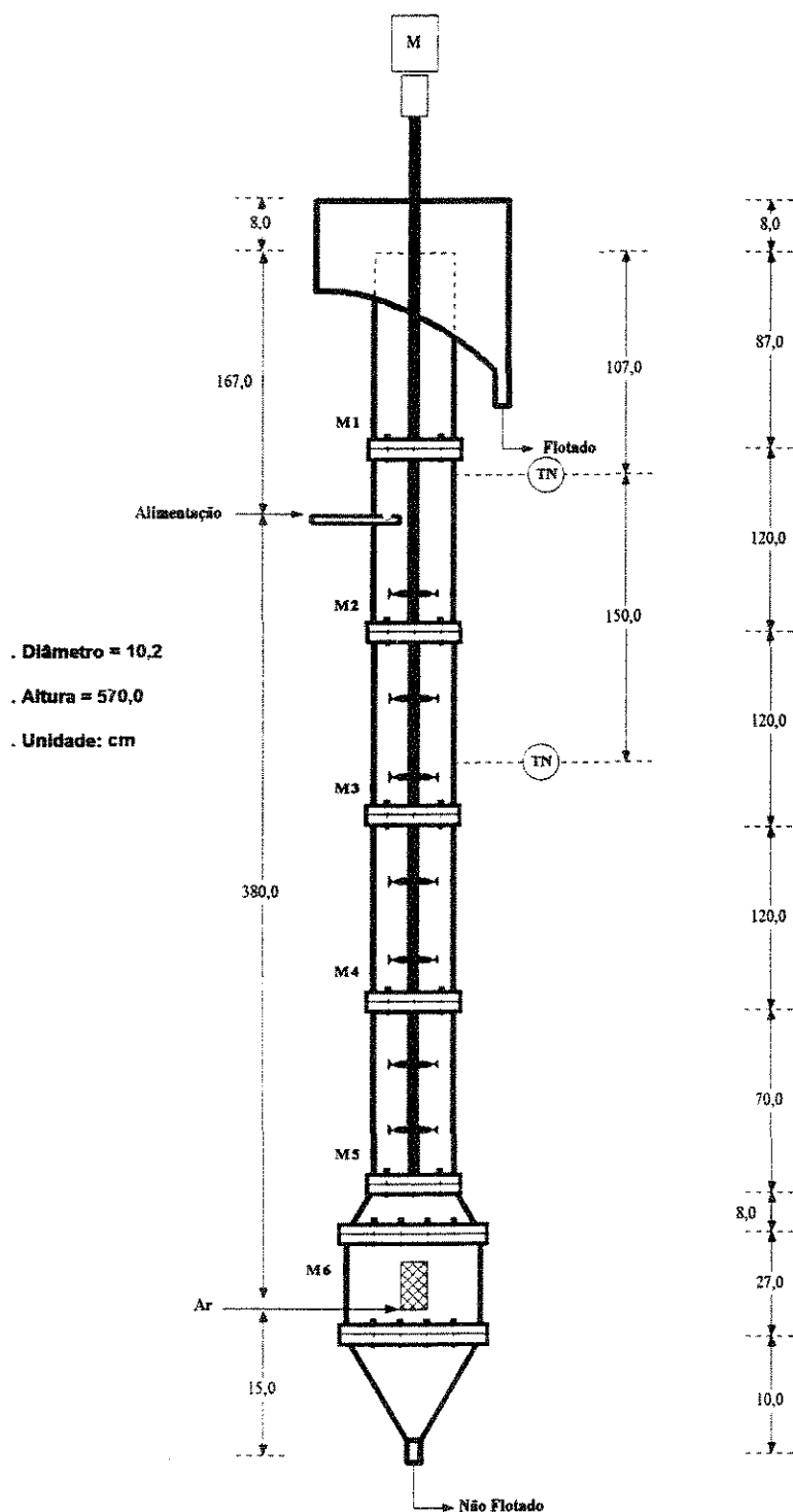
Figura III.5 - Desenho esquemático da coluna agitada
