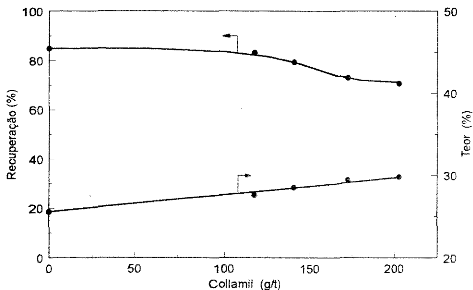
Figura V.1 - Efeito da dosagem de collamil sobre o teor e recuperação de P_2O_5 no concentrado
