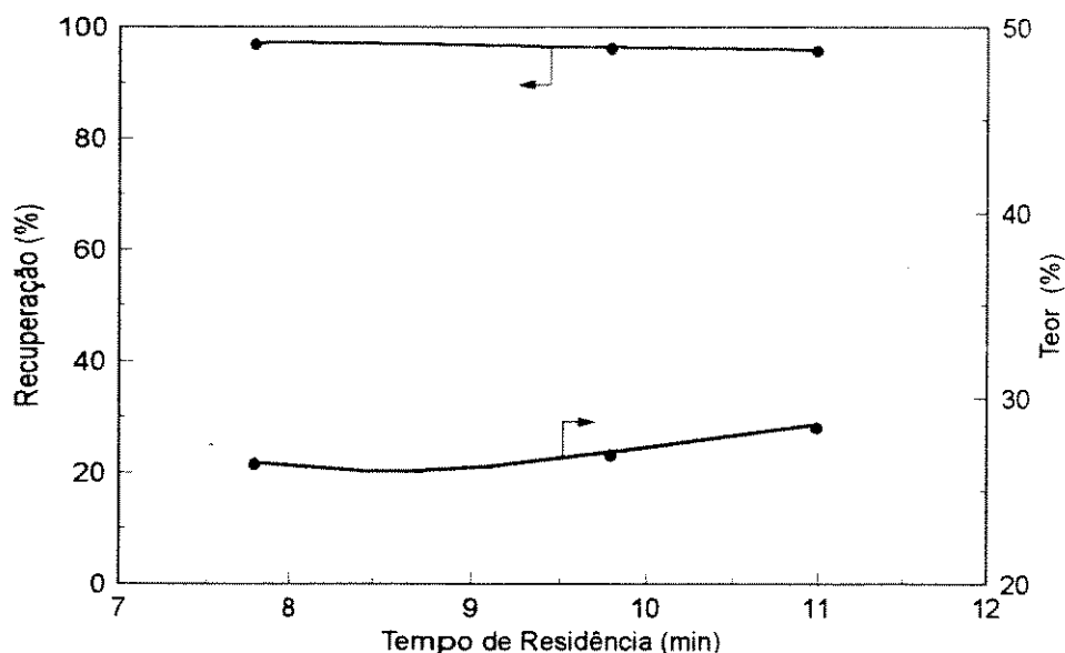
Figura VI.6 - Efeito do tempo de residência sobre o teor e recuperação de P_2O_5 no concentrado
