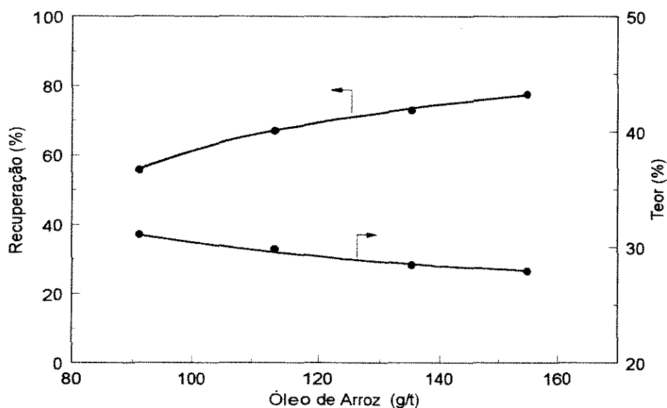
Figura V.2 - Efeito da dosagem de óleo de arroz sobre o teor e recuperação de P_2O_5 no concentrado
