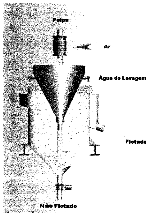
Figura II.6 – Desenho esquemático da célula pneumática do tipo Bahr
