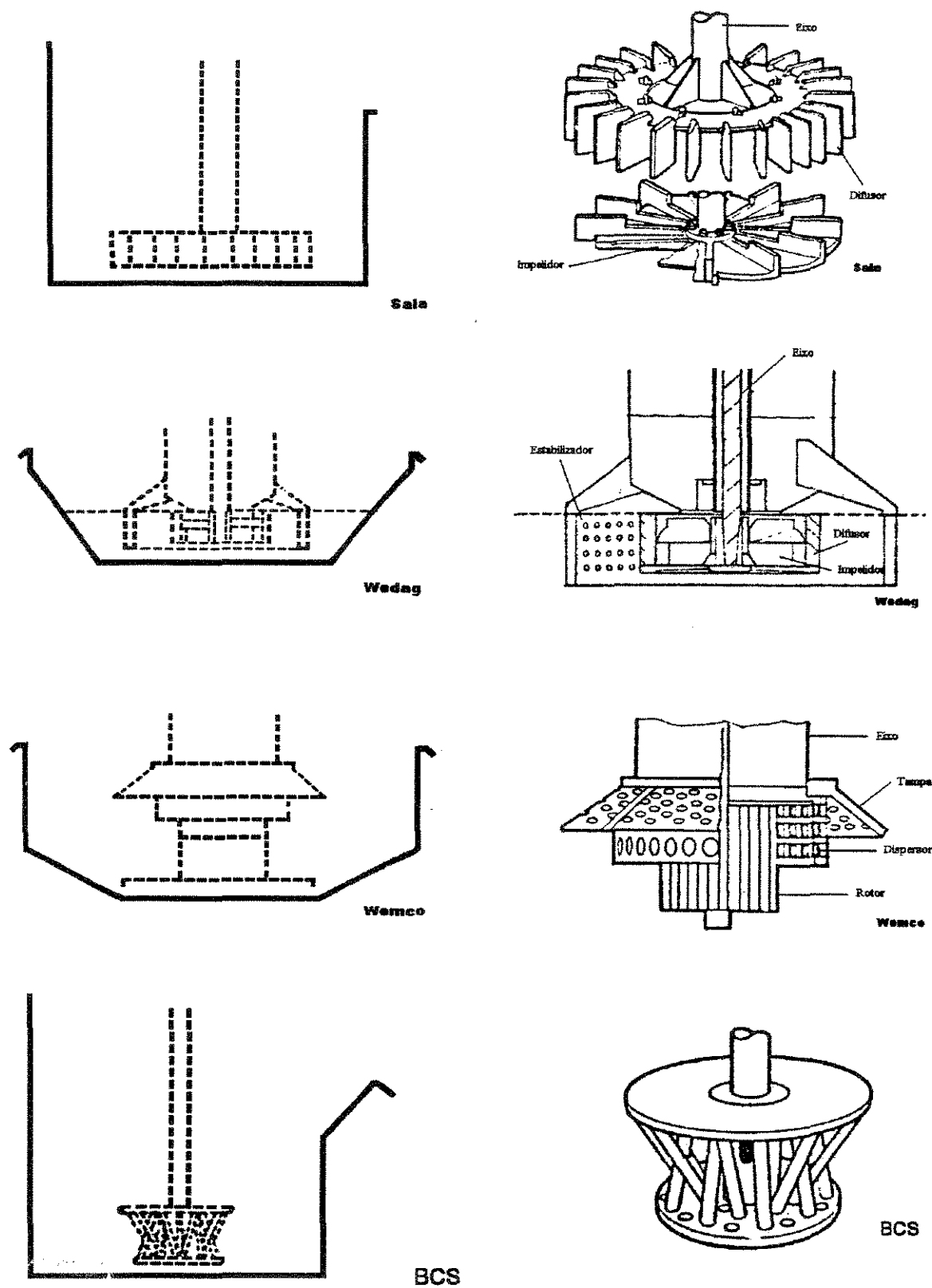
Figura II.3 – Desenho esquemático de tanques e rotores das células mecânicas Sala, Wedag, Wemco e BCS
