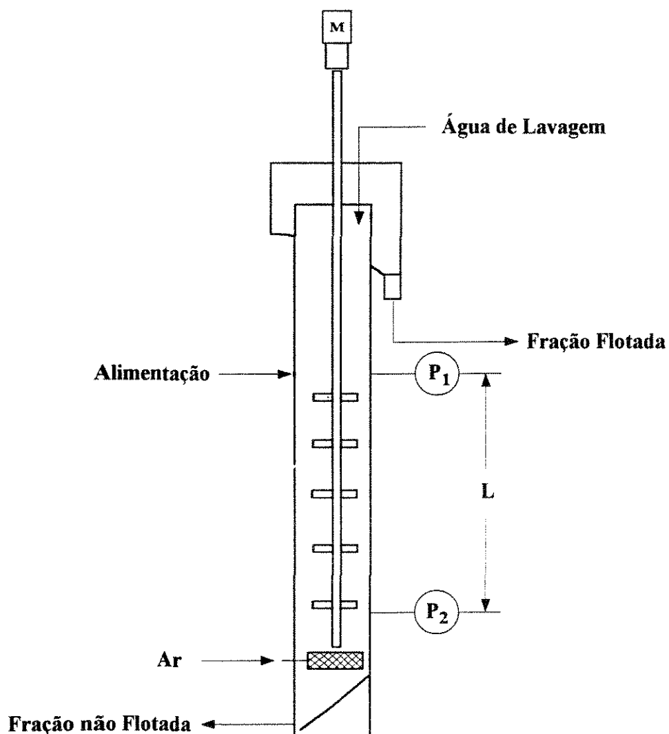
Figura II.13 - Desenho esquemático da coluna agitada
