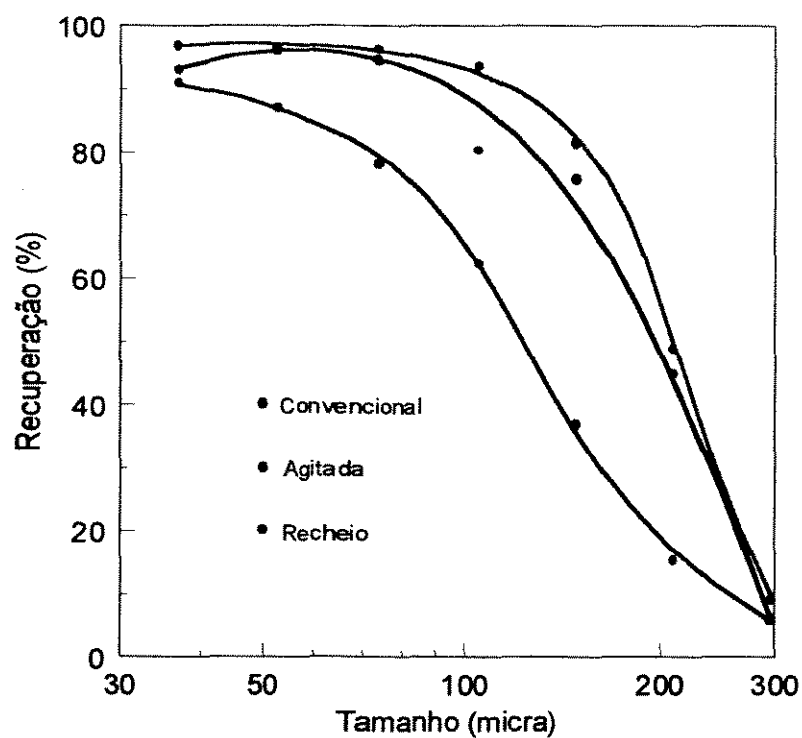
Figura V.22 – Recuperação de P_2O_5 em função do tamanho de partícula nas colunas convencional, agitada e de recheio
