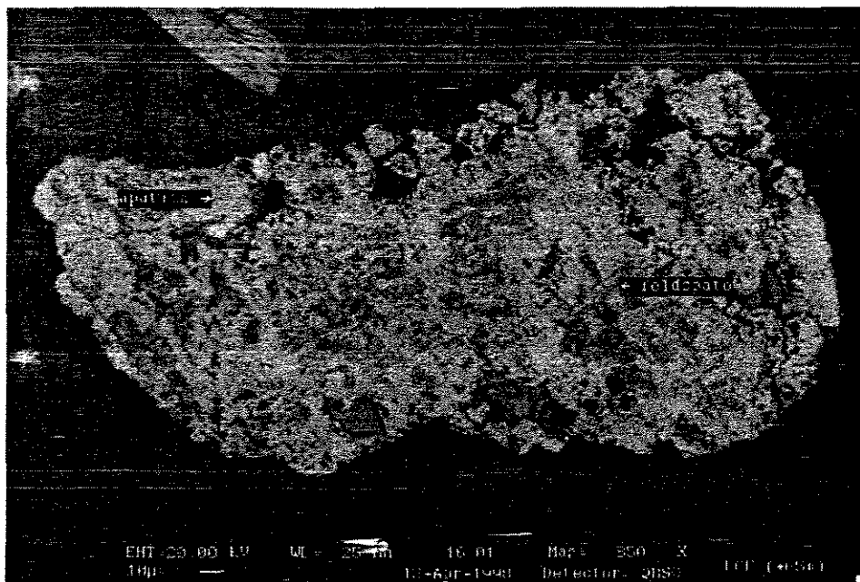
Figura IV.17 – Imagem de elétrons retroespalhados obtida através de microscópio eletrônico de varredura em grão de apatita intercrescido com feldspato
