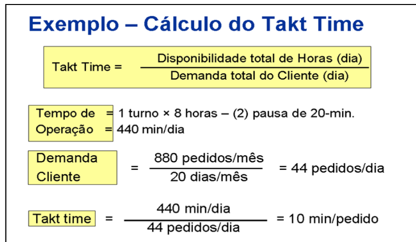
Figura 2.14: Cálculo do Takt time
