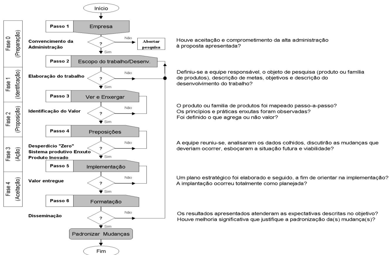
Figura 4.12: Fluxograma simplificado do método de melhoria da manufatura
