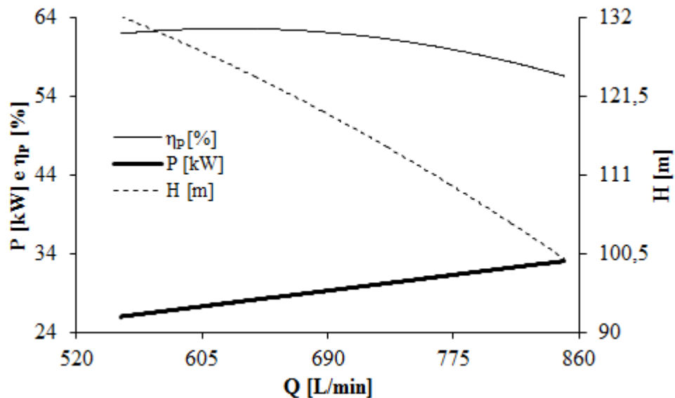
Figura 3.4 – Curvas de desempenho da bomba booster para 3500 [rpm] e 60 [Hz].
