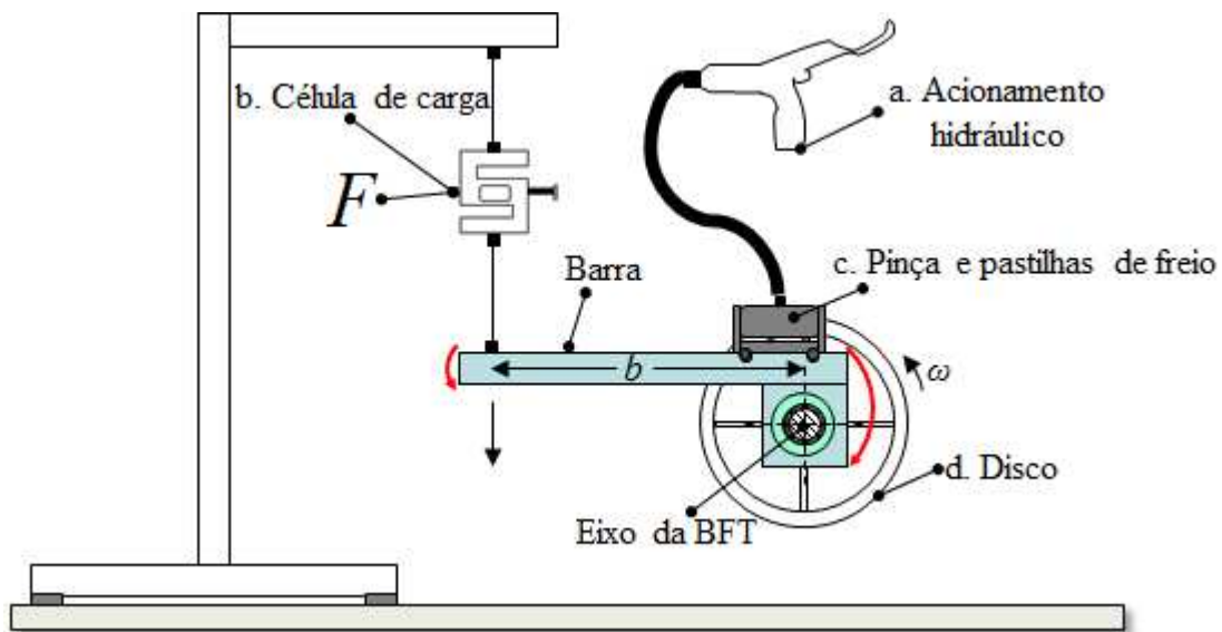
Figura 3.5 – Sistema de freio de Prony.
