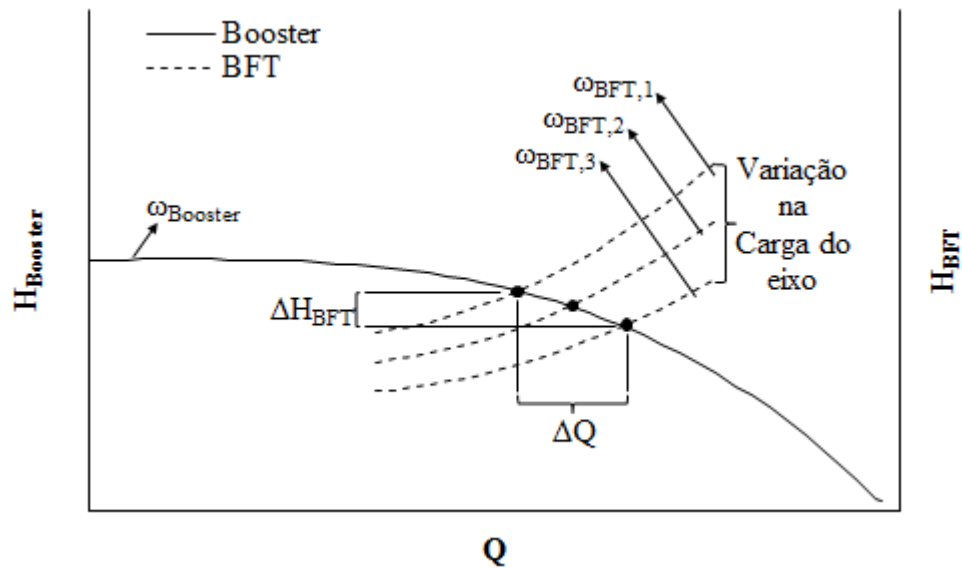
Figura 3.9 – Curva de altura manométrica em função da vazão para uma bomba booster e, para uma BFT com diferentes cargas no eixo.
