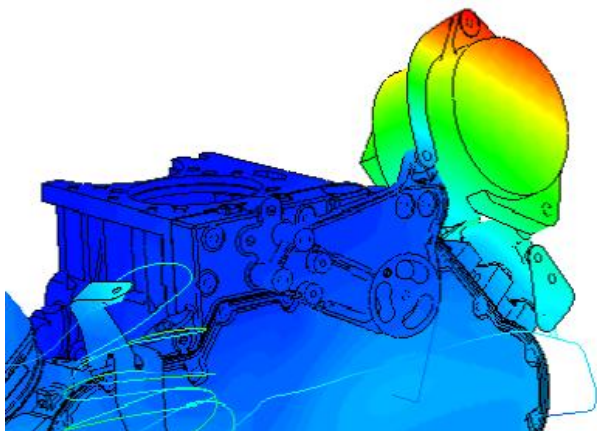
Figura 5.5- Análise modal do alternador -1º modo de vibrar (eixo X) – 144,1Hz
