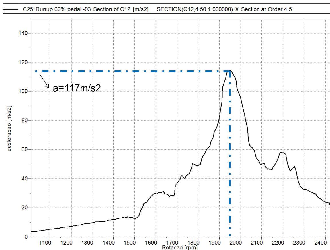
Figura 5.3- Curva característica de aceleração ( \text{m/s}^2 ) em função da rotação do motor (RPM) com 60% de carga na 4,5ª ordem
