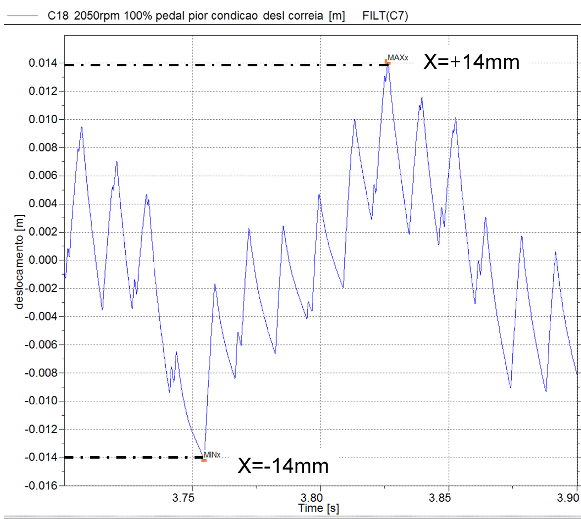
Figura 5.15- Gráfico ampliado do nível de deslocamento linear do vão livre da correia (m) em função do tempo (s) com 100% de carga à rotação de 2050rpm.
