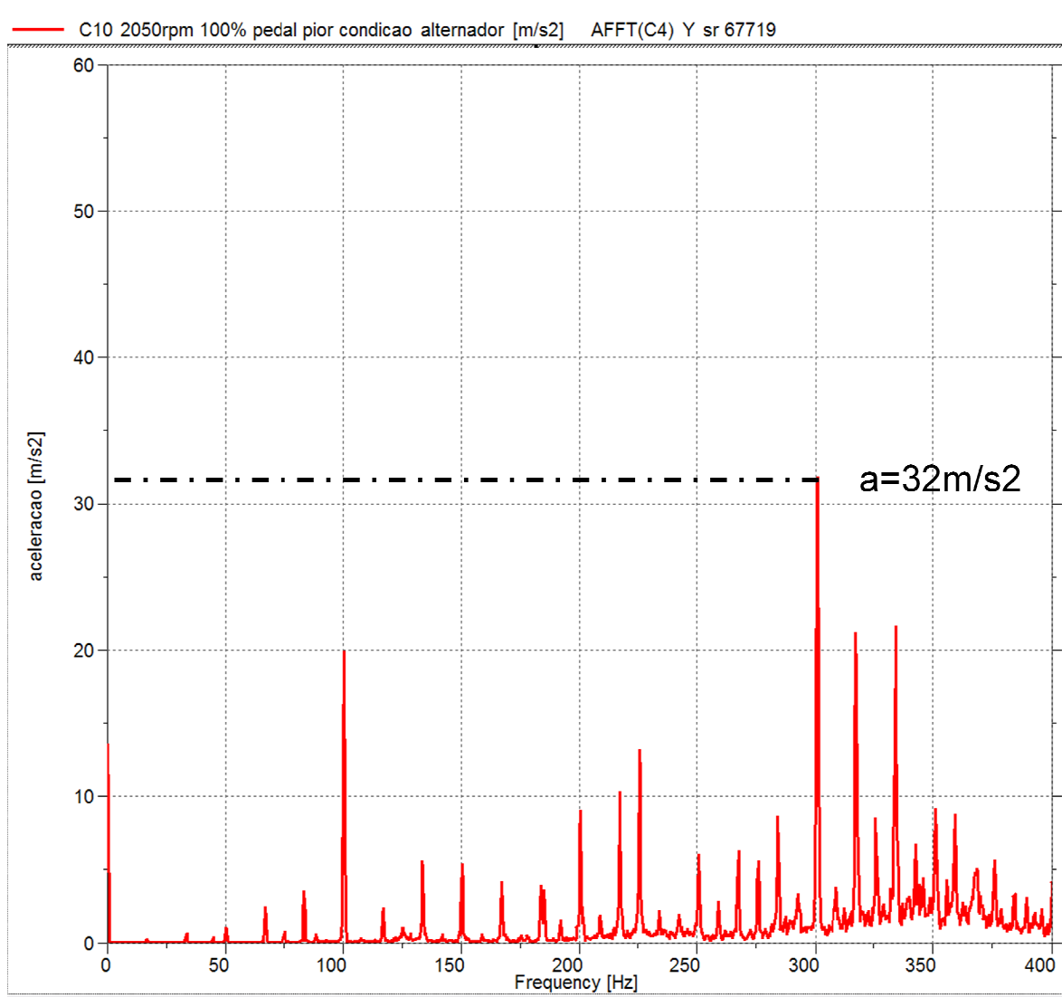
Figura 5.8- Gráfico do nível de aceleração do alternador ( \text{m/s}^2 ) no eixo Y em função da frequência (Hz) com 100% de carga à rotação de 2050rpm.
