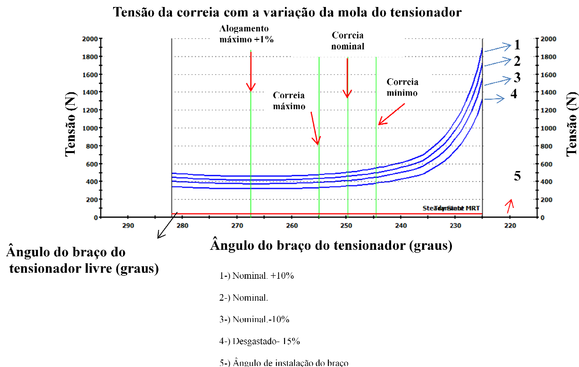
Figura 4.2- Curva característica do tensionador testado em dinamômetro
