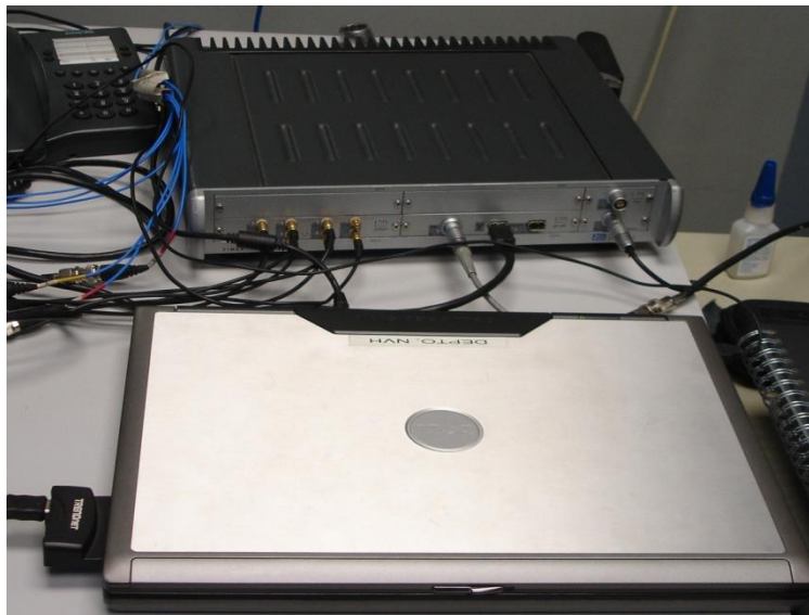
Figura 4.3- Equipamento LMS Pimento 8 canais e software LMS Pimento 6.1
