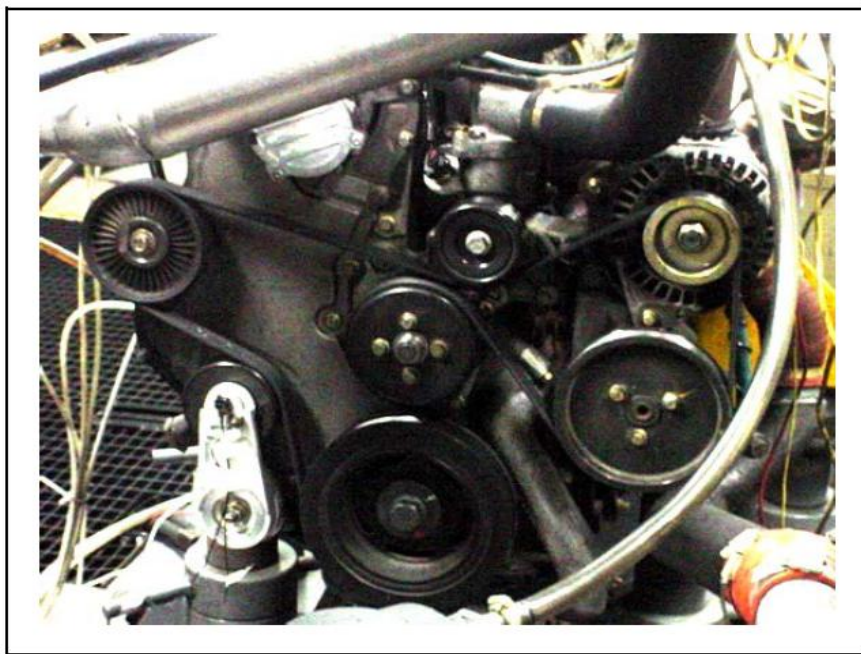
Figura 6.1- Exemplo de um sistema de acionamento frontal por correia
