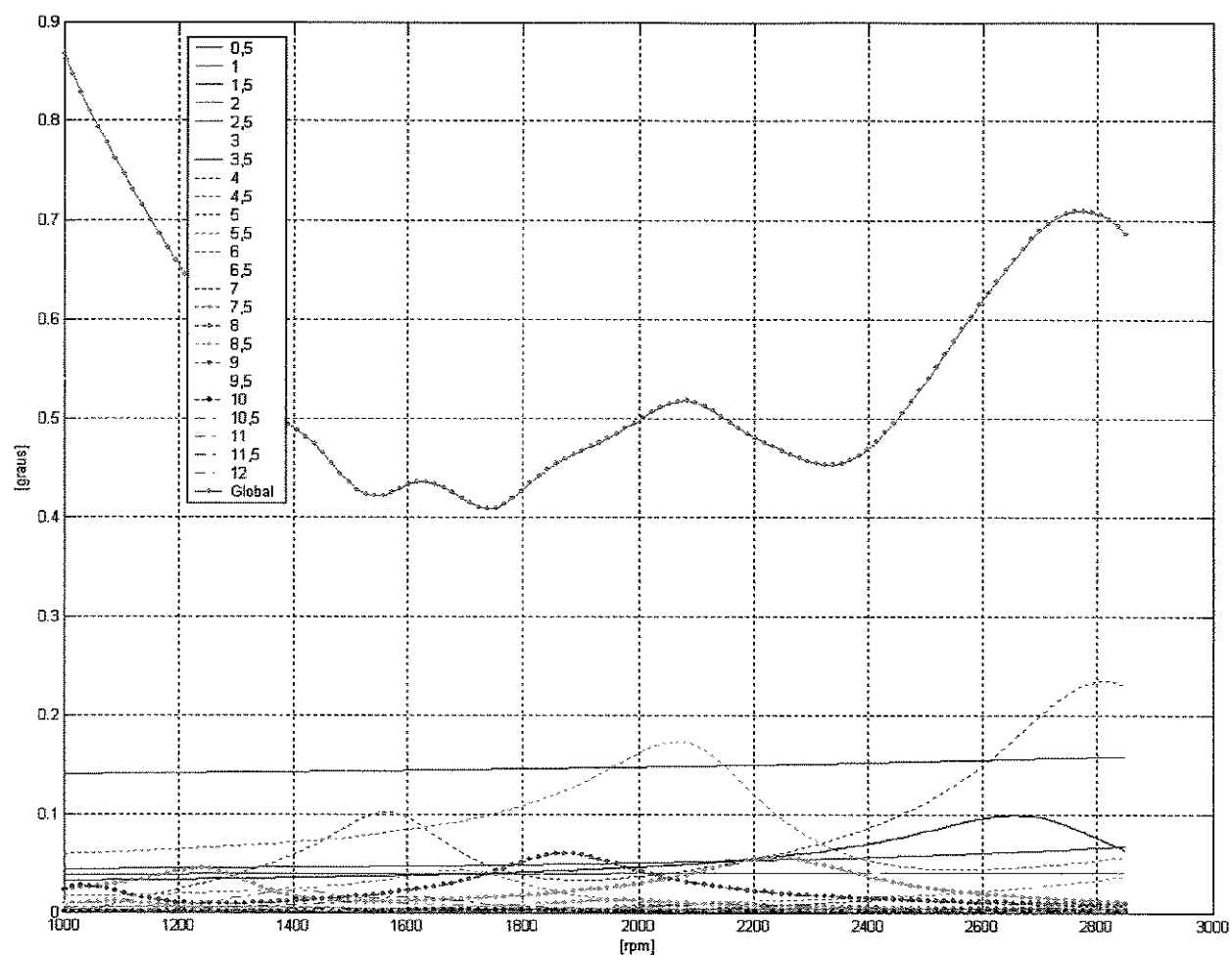
Figura A.3: Amplitudes de vibrações torcionais
