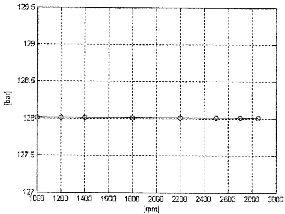
Figura A.2: Picos de pressão de combustão em função da rotação do motor
