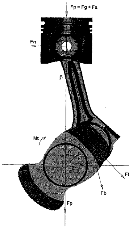
Figura 3: Esforços atuantes na árvore de manivelas.
