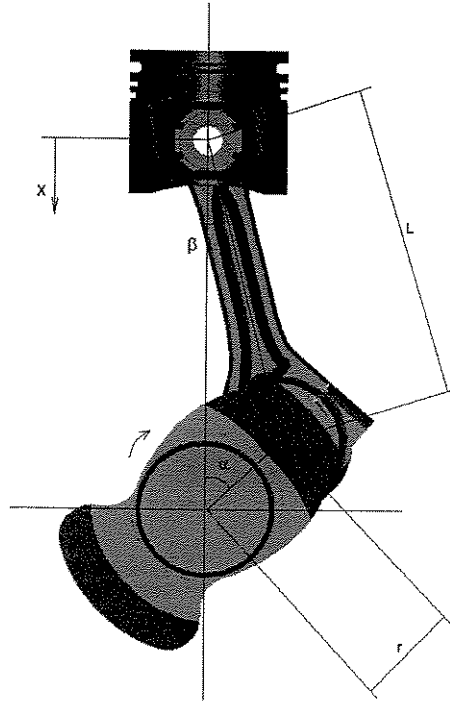
Figura 3.1: Sistema biela-manivela
