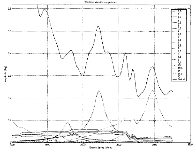
Figura 10: Torciograma.
