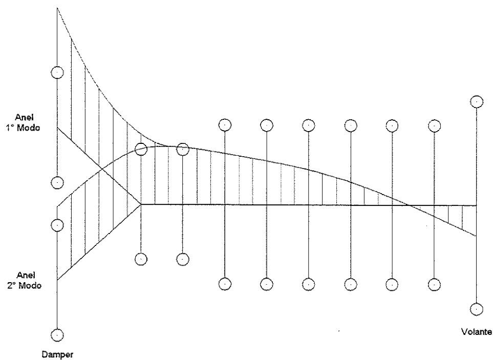
Figura 4.1: Representação gráfica do 1º modo de vibrar (112,23 Hz)
