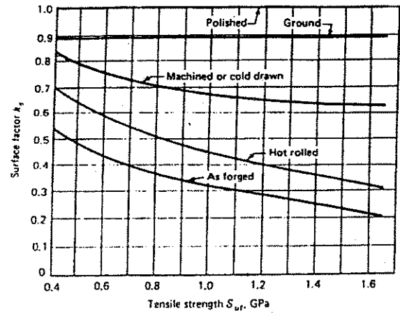
Figura 17: Fator de acabamento superficial [10].
