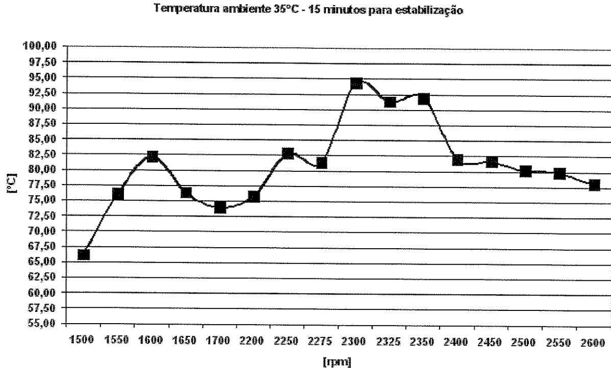
Figura 4.17: Medições de temperatura no anti-vibrador
