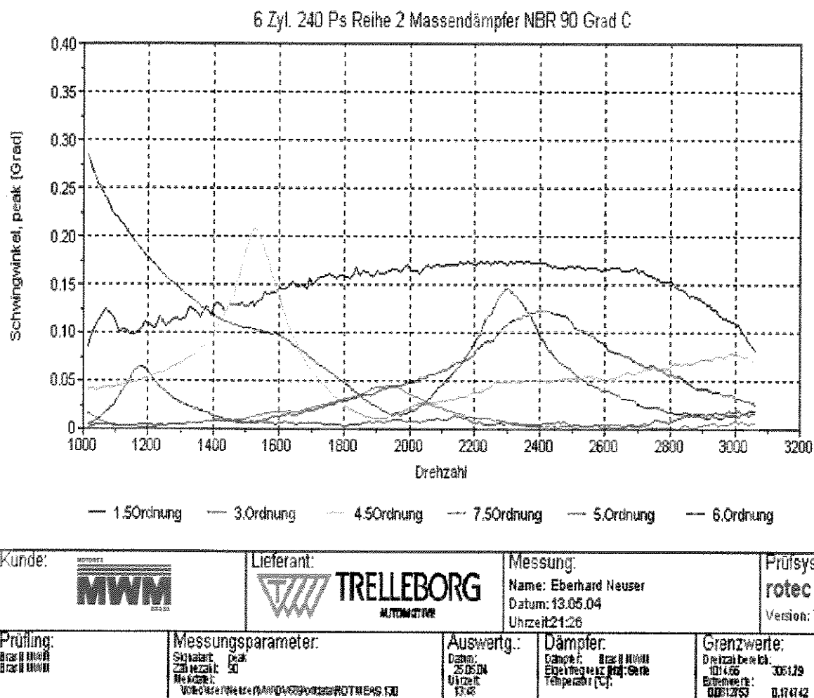
Figura 4.16: Amplitudes de vibrações torcionais das ordens mais significativas
