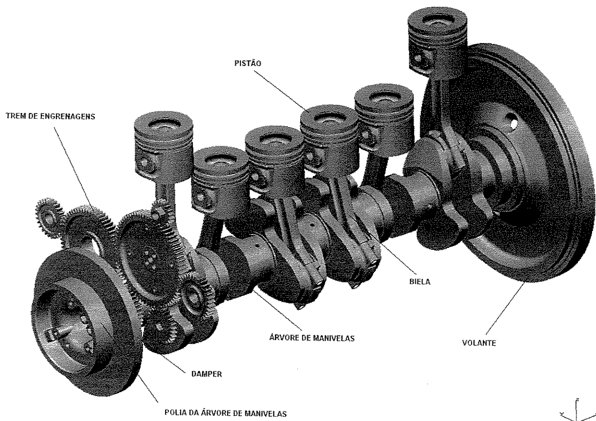
Figura 1.4: Árvore de manivelas e demais componentes responsáveis pela geração de torque do motor
