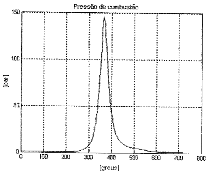
Figura 3.3: Curva experimental p = f(\alpha) para a condição de 2500 rpm a plena carga.
