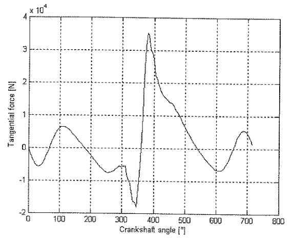
Figura 4: Força tangencial para a condição de 2500 rpm.
