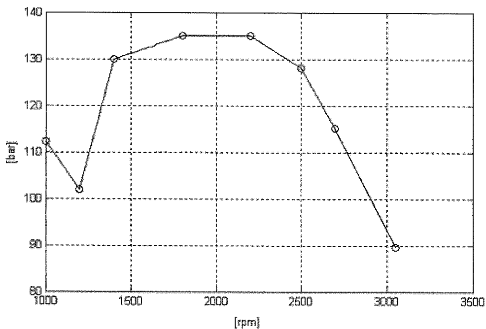
Figura 4.14: Picos de pressão de combustão em função da rotação do motor
