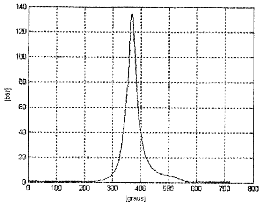
Figura 4.13: Curva experimental de pressão de combustão a 1800rpm em plena carga
