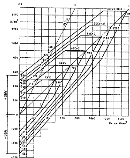
Figura 16: Diagrama de Goodman modificado.
