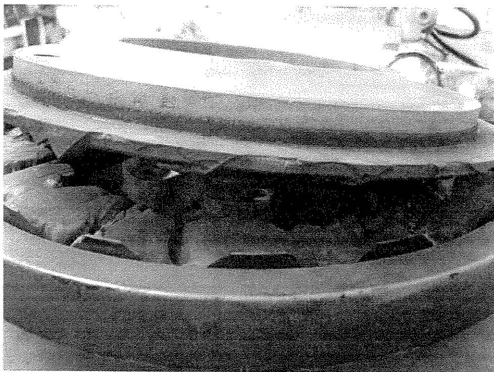
Figura 4.12: Falha do amortecedor por cisalhamento da borracha do primeiro anel
