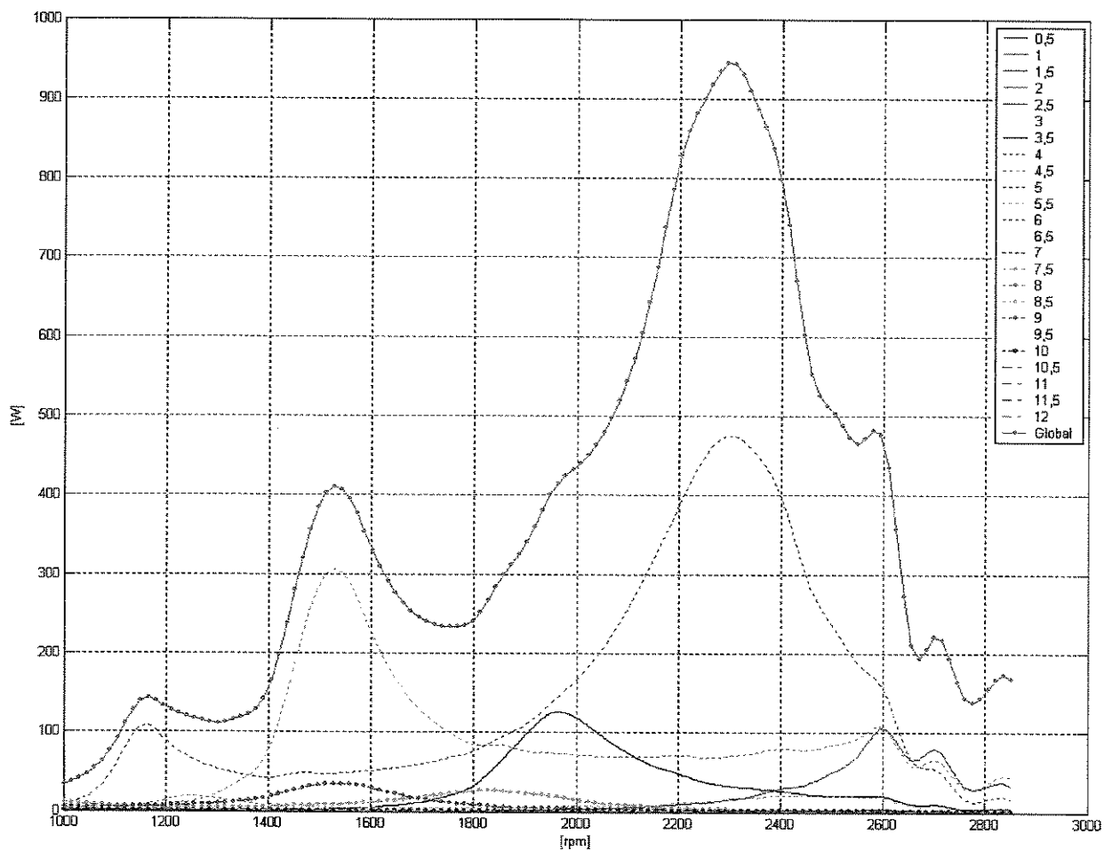
Figura 4.10: Potência dissipada pela borracha do anel do primeiro modo de vibrar
