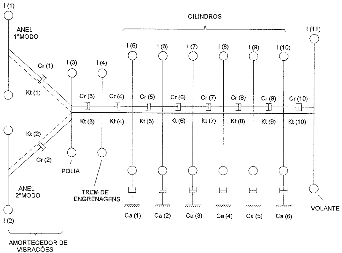
Figura 3.7: Modelo equivalente
