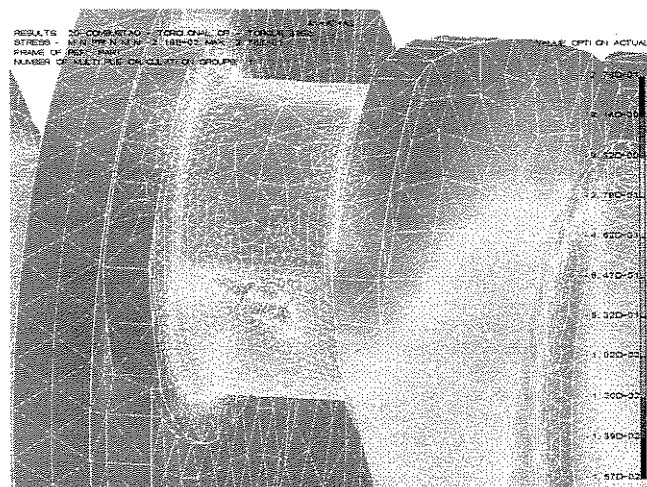
Figura 14: Tensão mínima principal.
