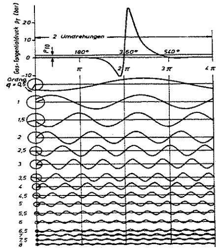
Figura 9: Exemplo de expansão em série de Fourier de uma curva de pressão tangencial.
