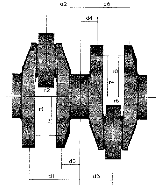
Figura 11: Dimensões para verificação do balanceamento.
