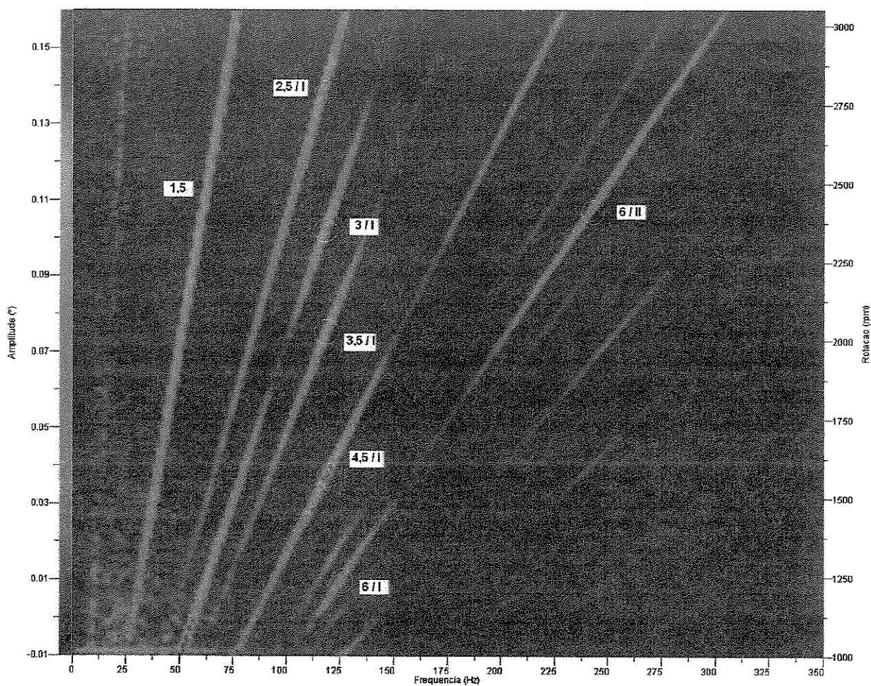
Figura 4.19: Diagrama de Campbell para análise de vibrações torcionais
