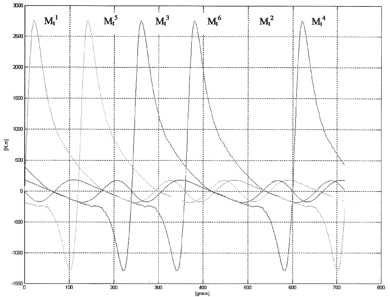
Figura 3.13: Curvas de torque teóricas para uma condição de 2600 rpm a plena carga
