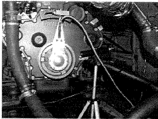
(c) – Encoder e Laser para medições das amplitudes
