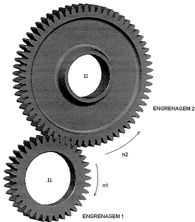
Figura 3.10: Esquema para redução da inércia de eixos com rotações diferentes ( n_1 e n_2 )
