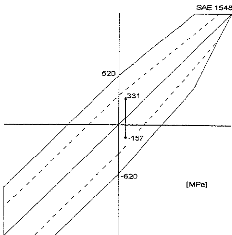
Figura 18: Diagrama de Goodman para o componente.
