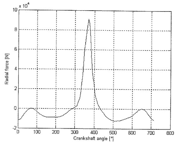
Figura 5: Força radial para a condição de 2500 rpm.
