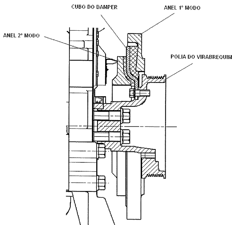
Figura 3.11: Amortecedor de vibrações torcionais de massa dupla
