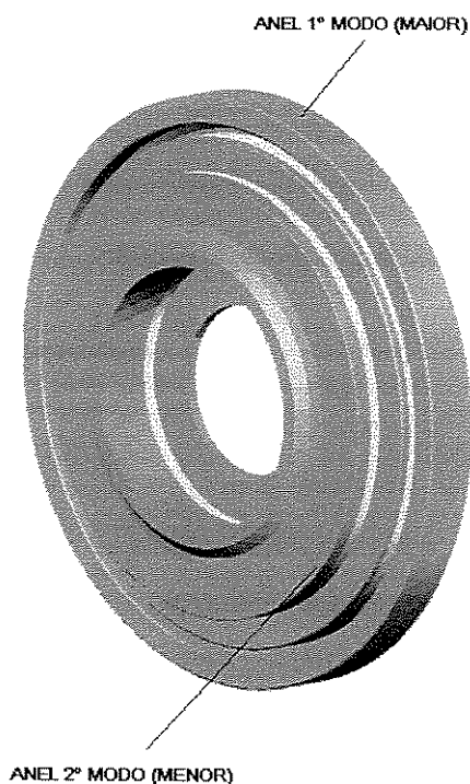
Figura 3.12: Modelo para a obtenção das rigidezes dinâmicas do amortecedor de vibrações
