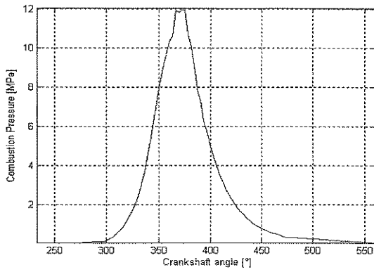
Figura 2: Curva p = f(\alpha) para a condição de 2500 rpm.
