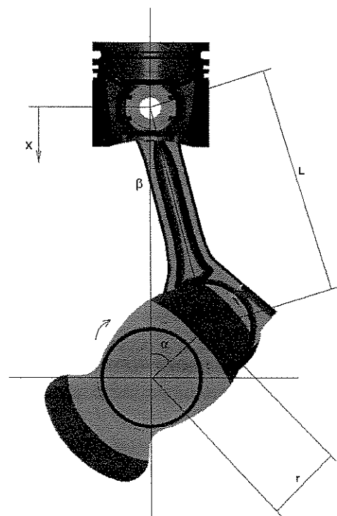
Figura 1: Sistema biela / manivela.
