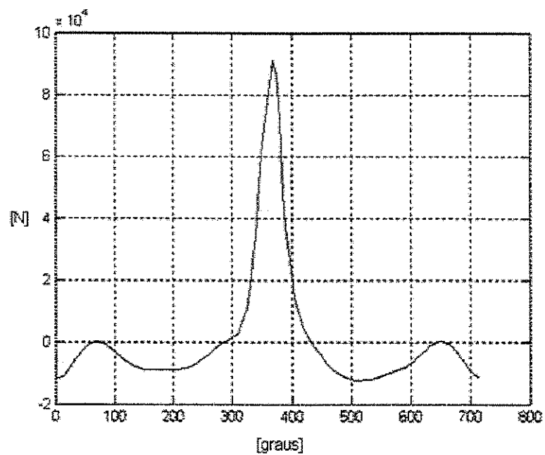
Figura 3.6: Força radial teórica resultante para a condição de 2500 rpm a plena carga
