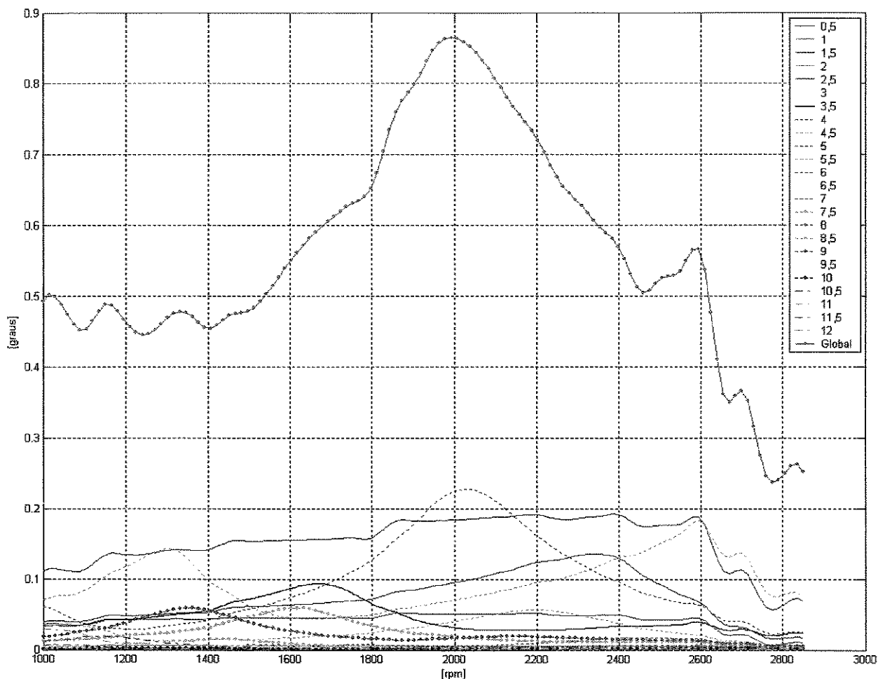
Figura 4.8: Amplitudes de vibrações torcionais com K_t(1) = 64254 \text{ N.m/rad} e K_t(2) = 88887 \text{ N.m/rad}
