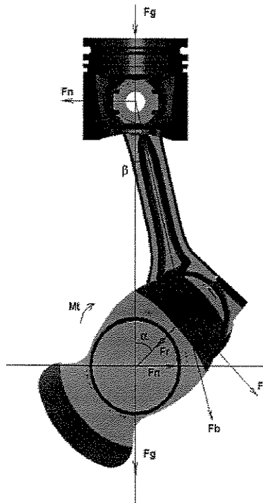
Figura 3.4: Esforços atuantes na árvore de manivelas
