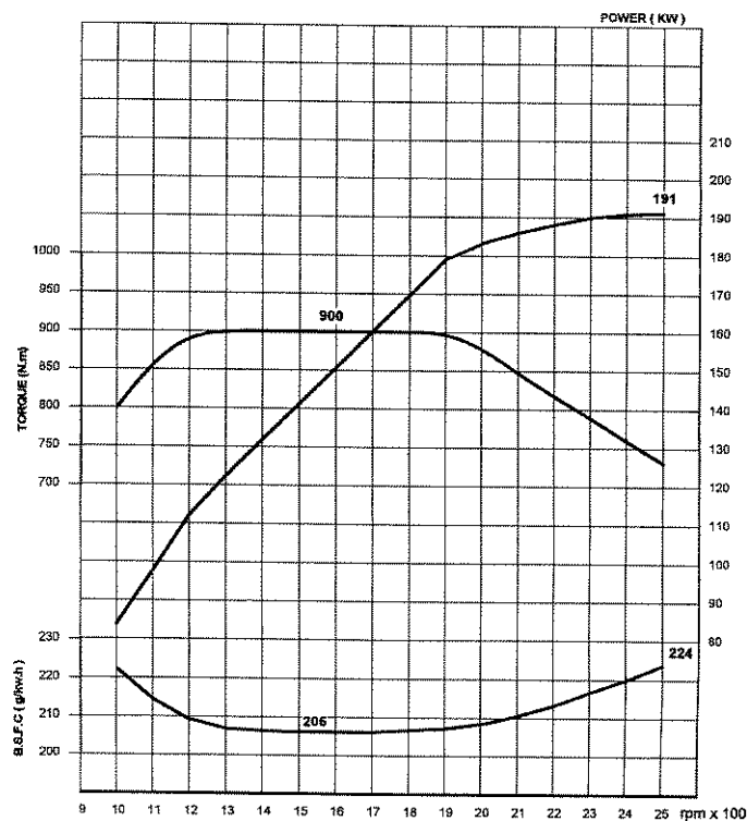
Figura 1.2: Curva de oferta do motor Acteon ®
