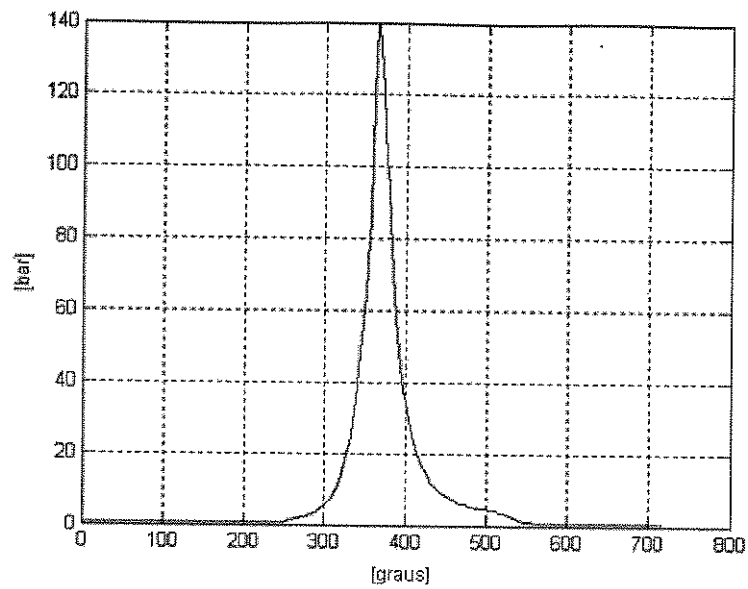
Figura 4.3: Curva experimental de pressão de combustão a 1000rpm e plena carga
