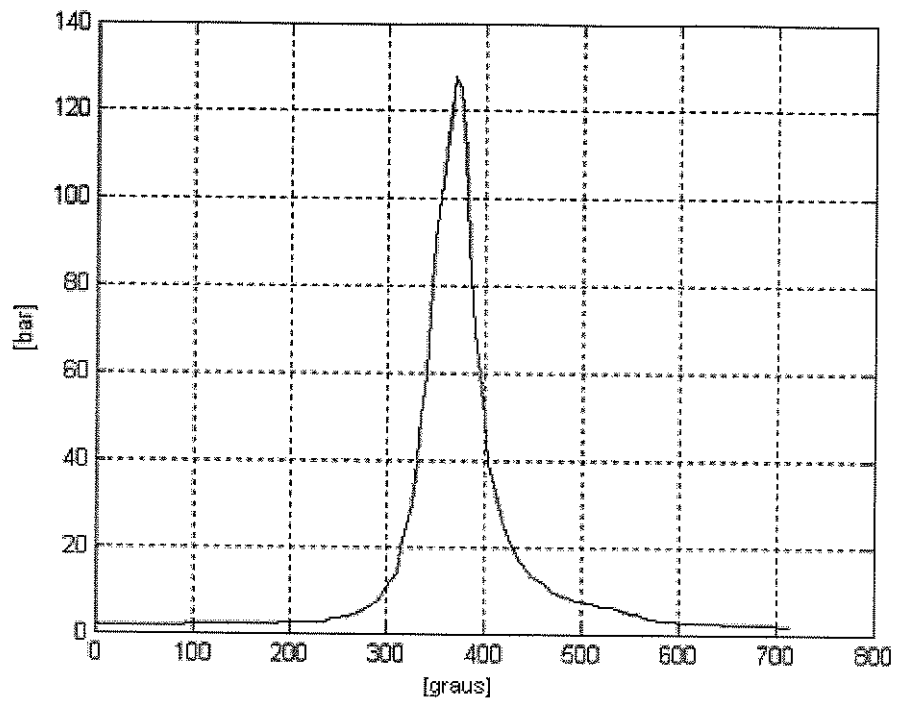
Figura A.1: Curva teórica de pressão de combustão
