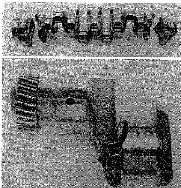
Figura 1.3: Falha estrutural em uma árvore de manivelas devido às vibrações torcionais excessivas
