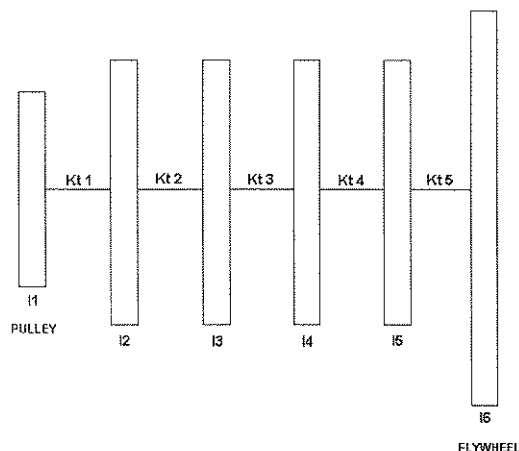
Figura 6: Modelo equivalente.
