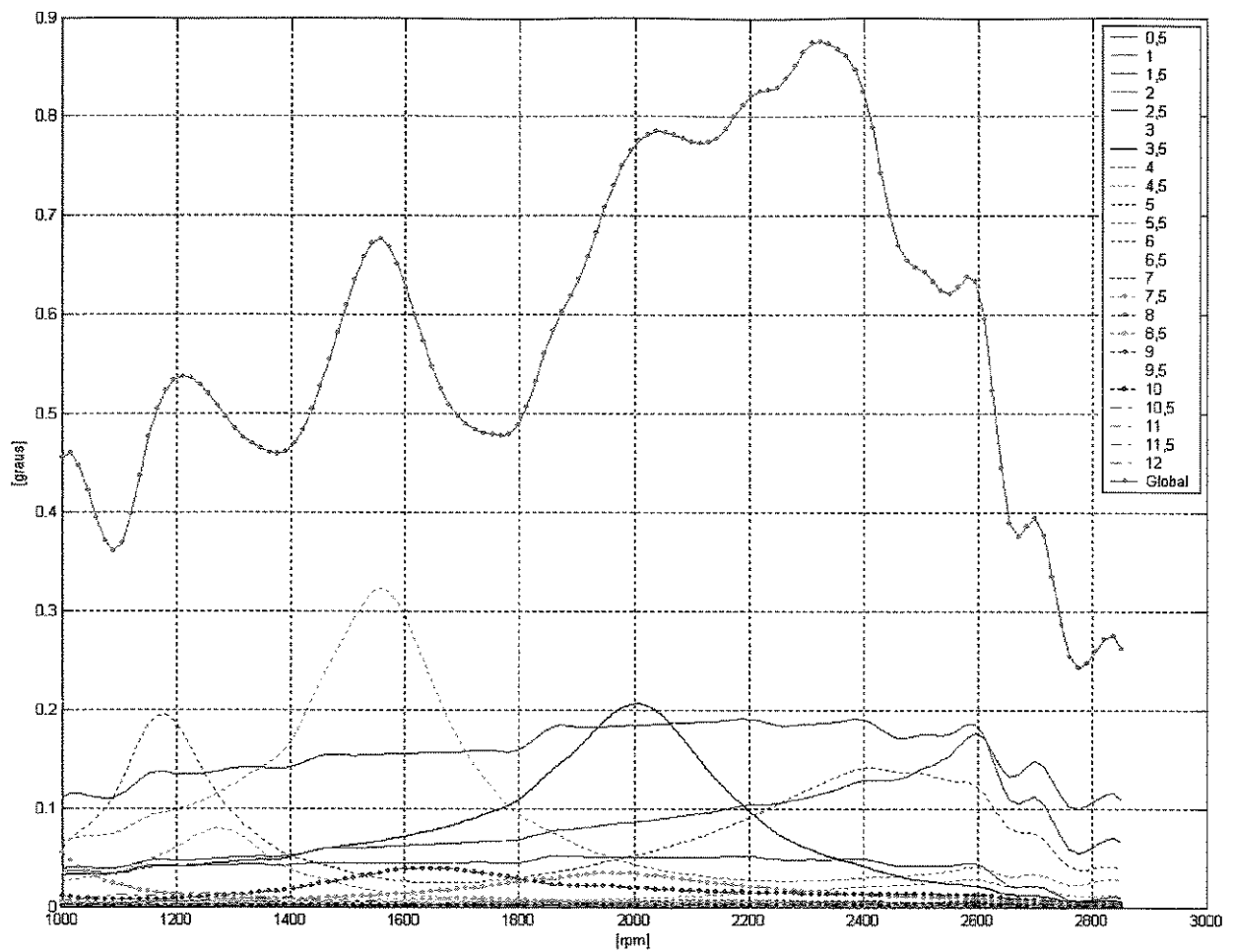
Figura 4.9: Amplitudes de vibrações torcionais com K_t(1) = 127999 \text{ N.m/rad} e K_t(2) = 177252 \text{ N.m/rad}
