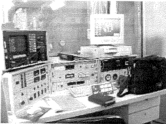
(a) – Painel de controle do dinamômetro
