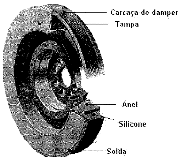
Figura 5.1: Detalhe de um amortecedor de vibrações torcionais do tipo viscoso
