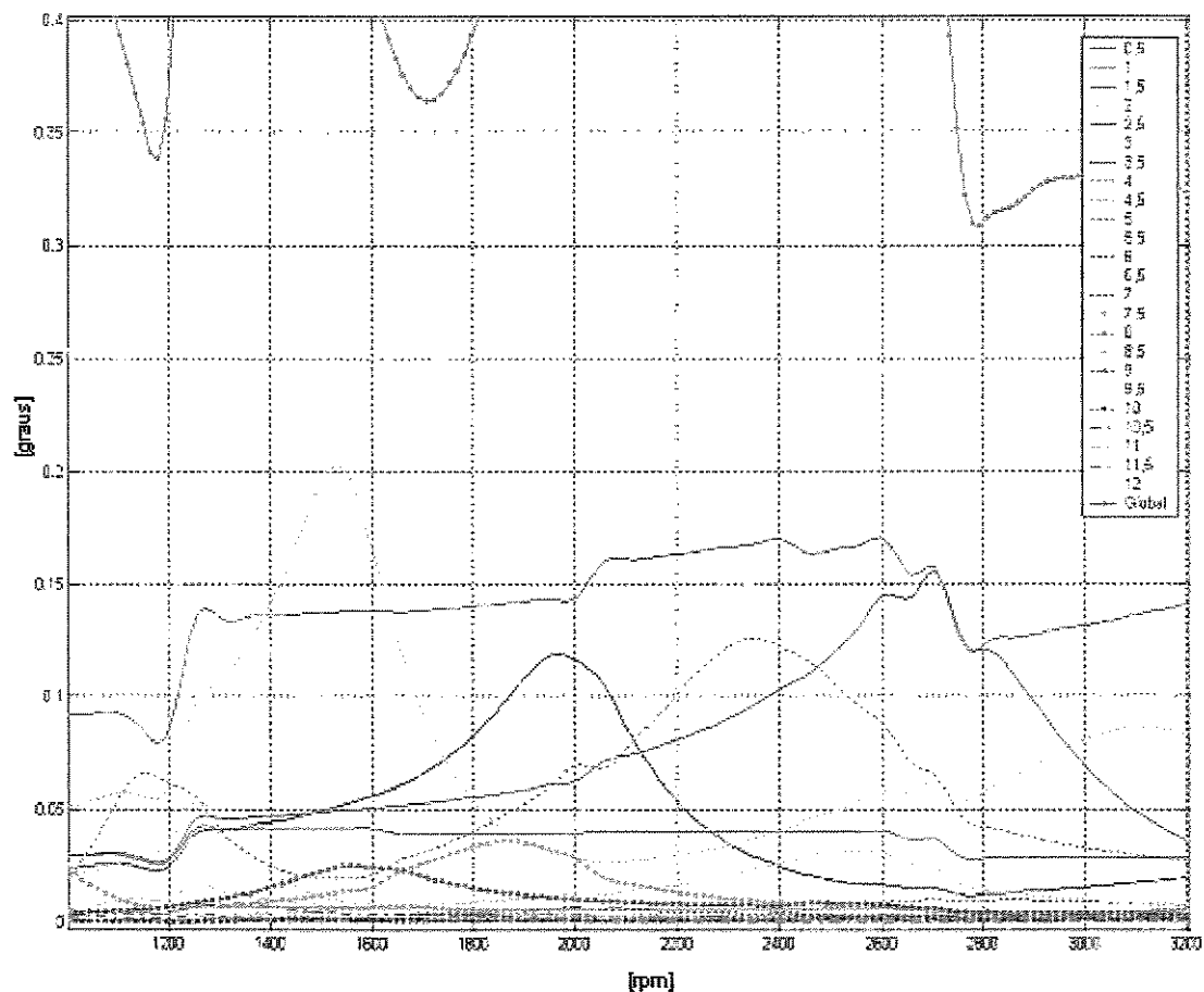
Figura 4.15: Amplitudes de vibrações torcionais
