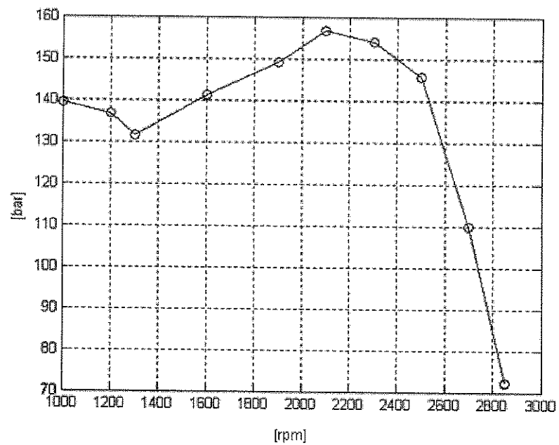
Figura 4.4: Picos de pressão de combustão em função da rotação do motor
