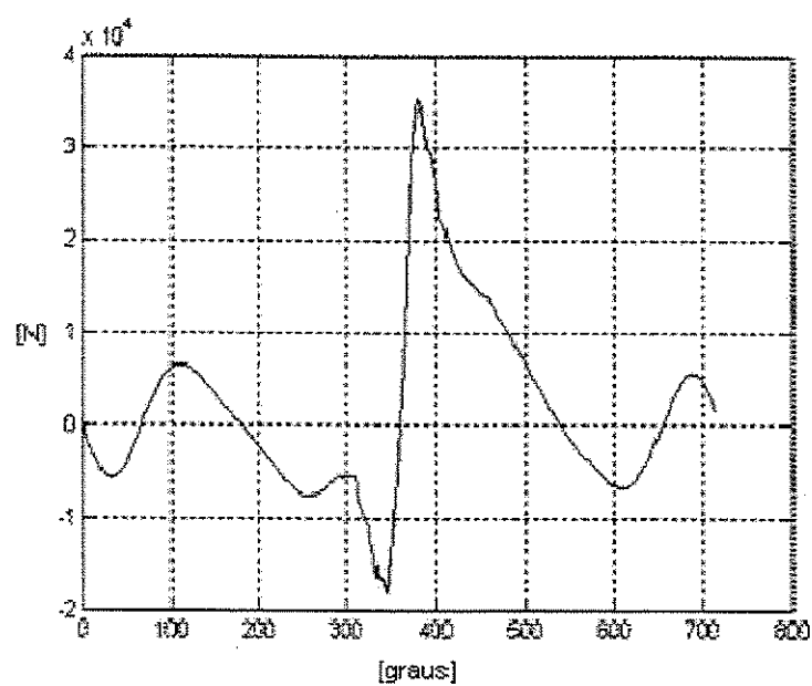
Figura 3.5: Força tangencial teórica resultante para a condição de 2500 rpm a plena carga
