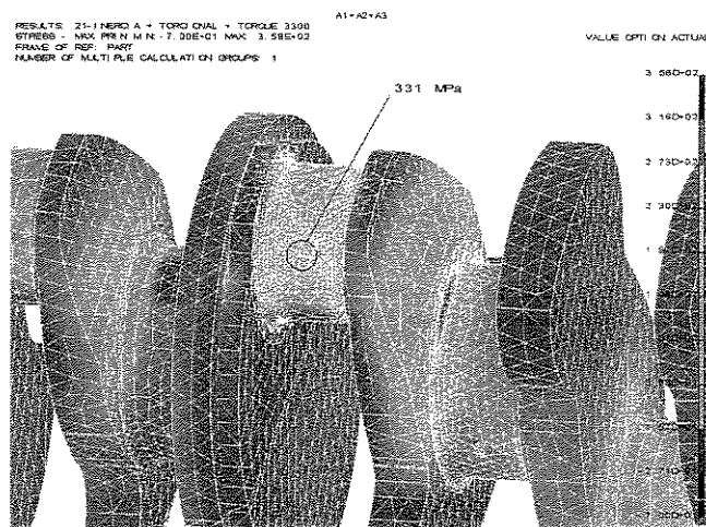
Figura 13: Tensão máxima principal.
