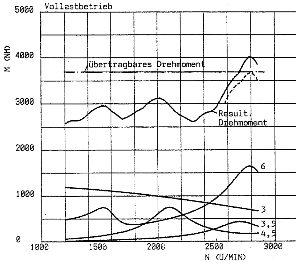
Figura A.6: Torque atuante entre o volante e o 6° cilindro das ordens mais significativas
