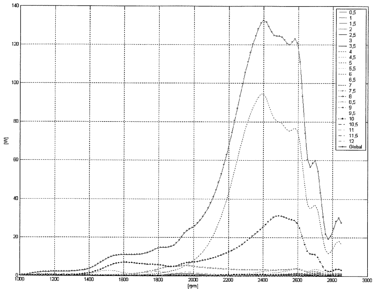
Figura 4.11: Potência dissipada pela borracha do anel do segundo modo de vibrar
