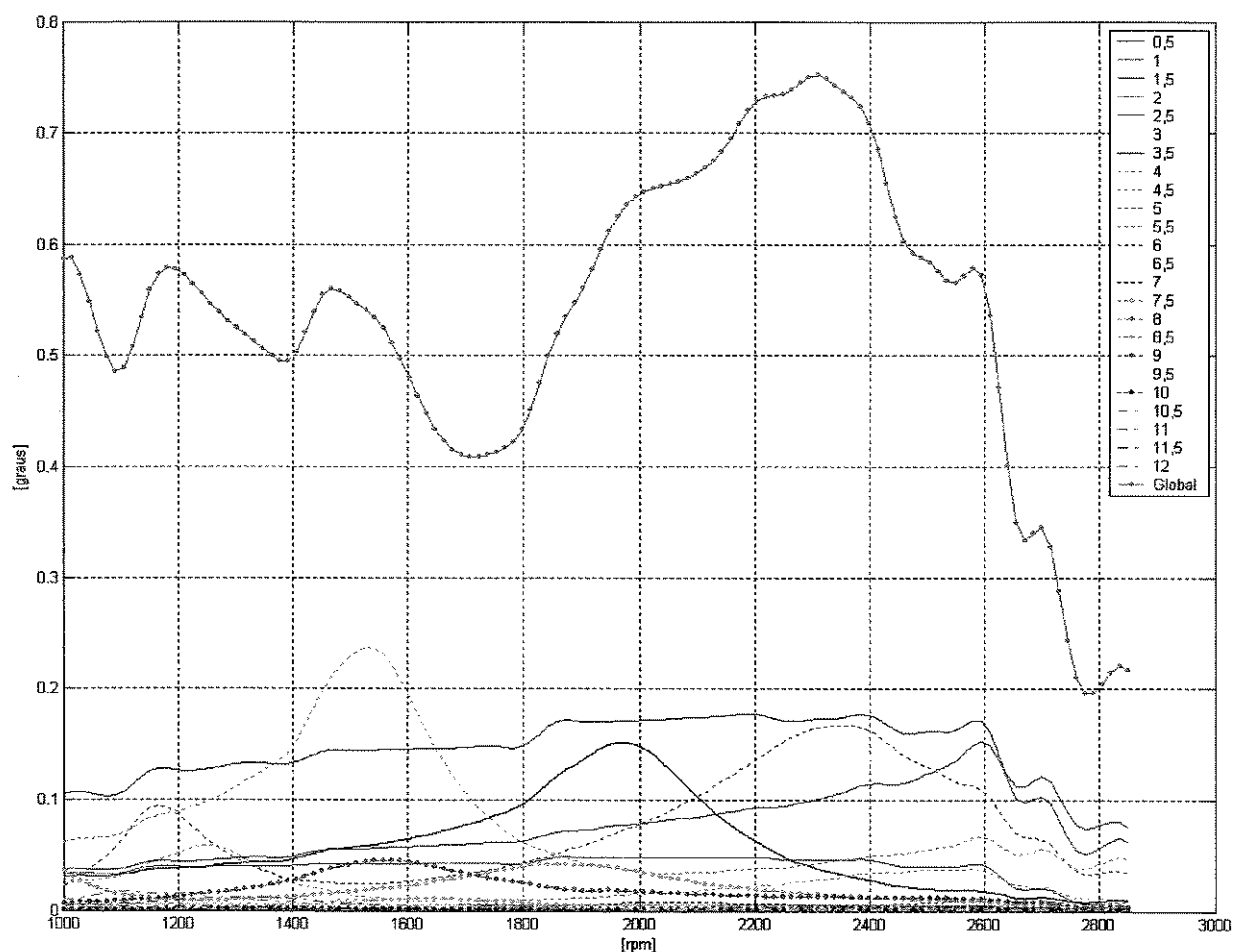
Figura 4.7: Amplitudes de vibrações torcionais considerando-se redução na inércia do volante
