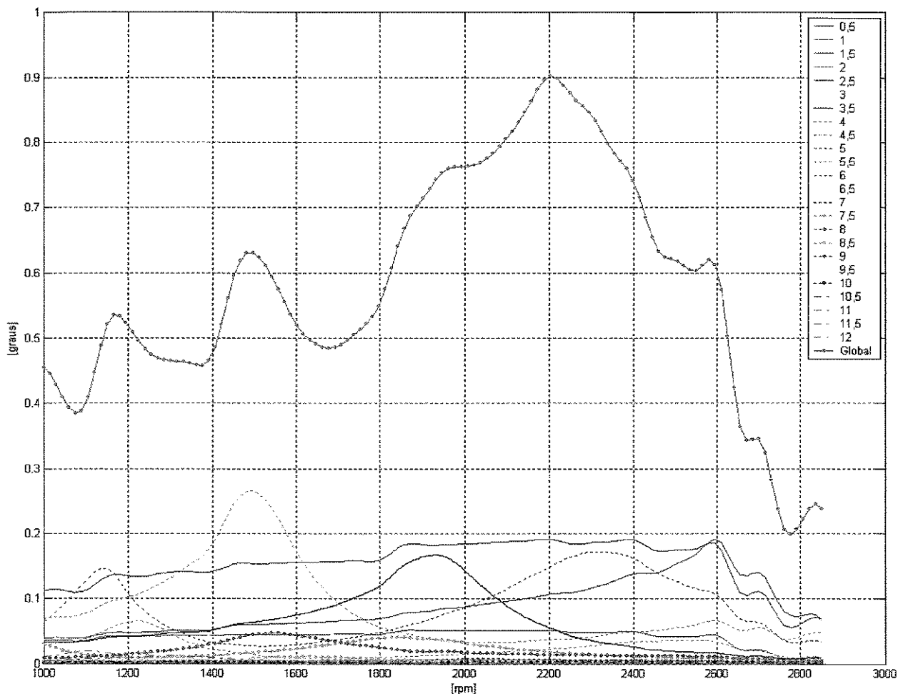
Figura 4.5: Amplitudes de vibrações torcionais
