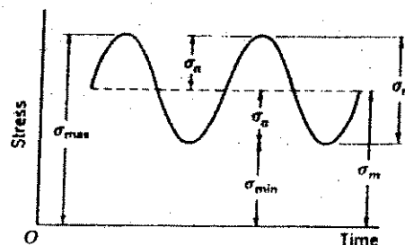
Figura 15: Tensões cíclicas.
