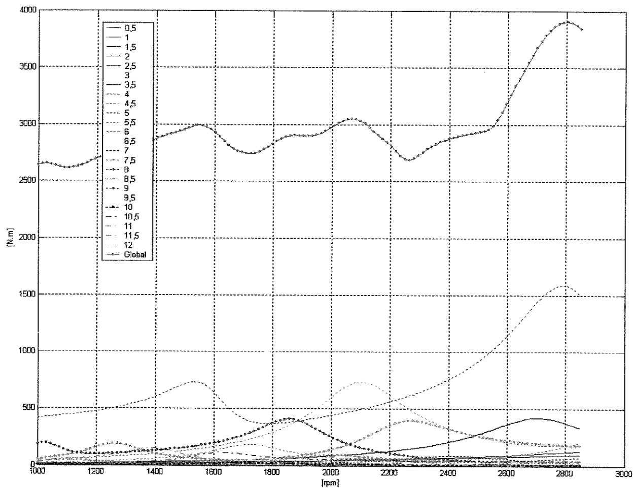
Figura A.4: Torque atuante entre o volante e o 6° cilindro
