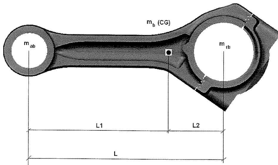
Figura 3.2: Divisão das massas da biela
