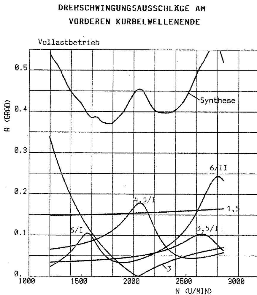
Figura A.5: Amplitudes de vibrações torcionais das ordens mais significativas
