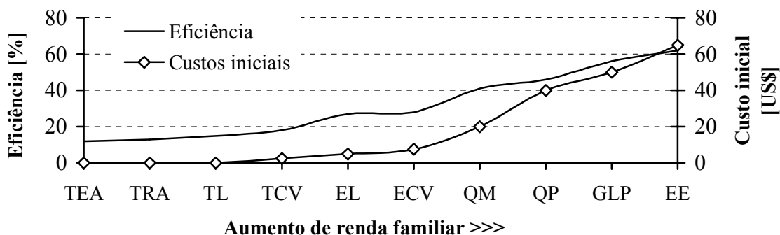
Figura 12: Comparação de eficiência e custos de fogões
