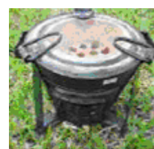
Fogão eficiente de forma cônica com duas câmaras de isolante cerâmico
