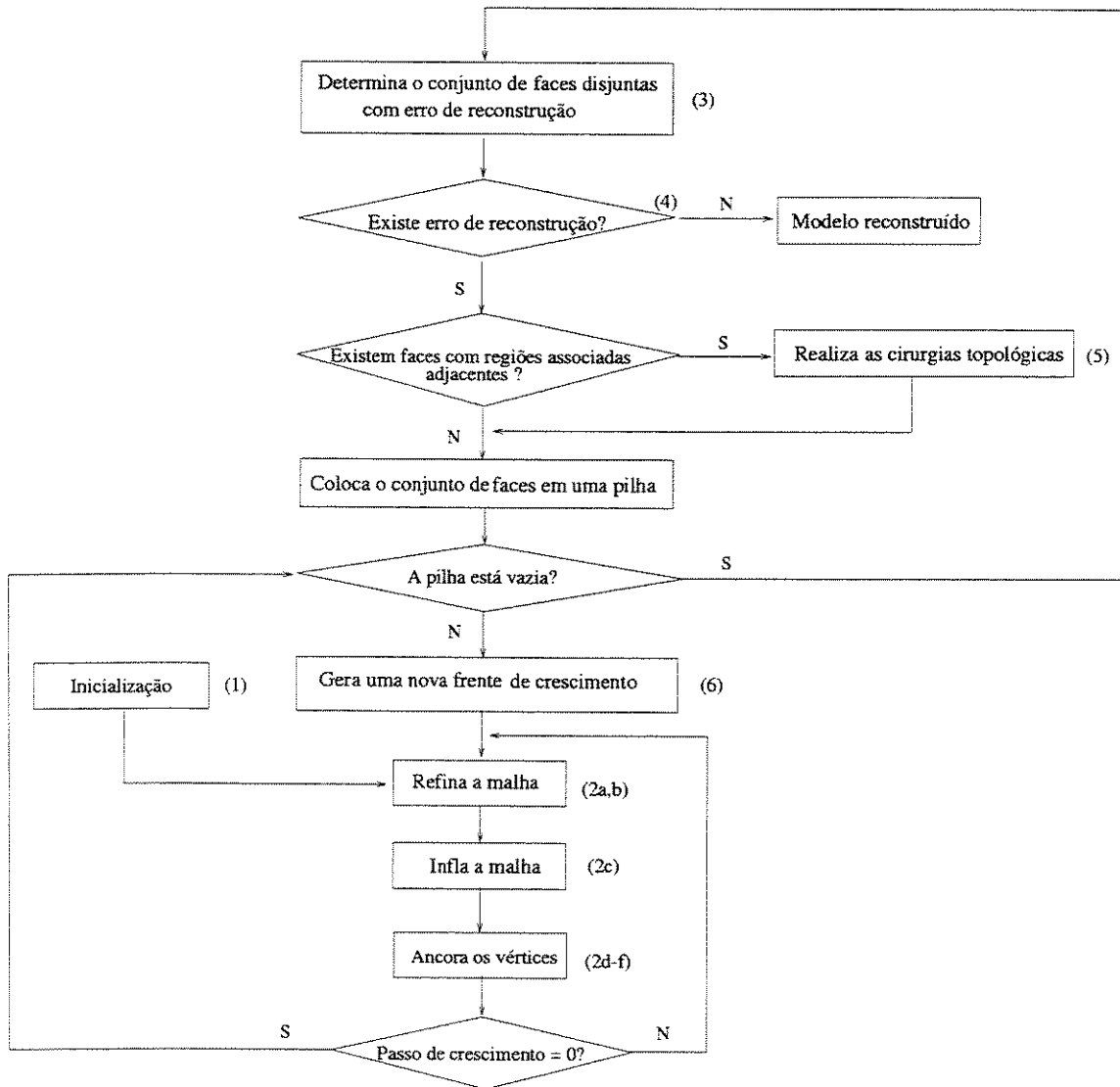
Figura 4.10: Fluxograma.
