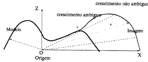
Figura 4.9: Direção ambígua de crescimento.
