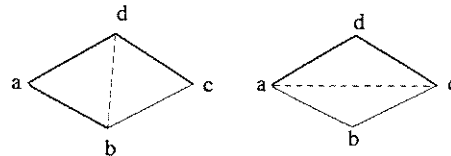
Figura 4.3: Configurações possíveis para bissecar uma face.
