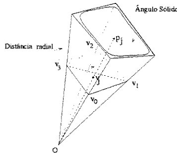
Figura 4.2: Ângulo sólido de procura do correspondente.
