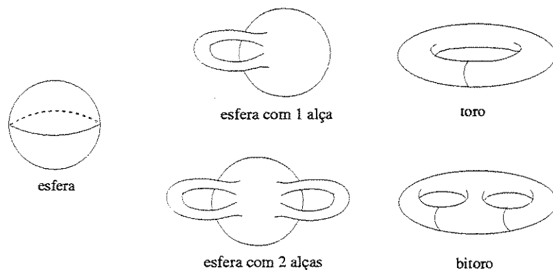
Figura 2.4: Superfícies orientáveis em \mathbb{R}^3 .
