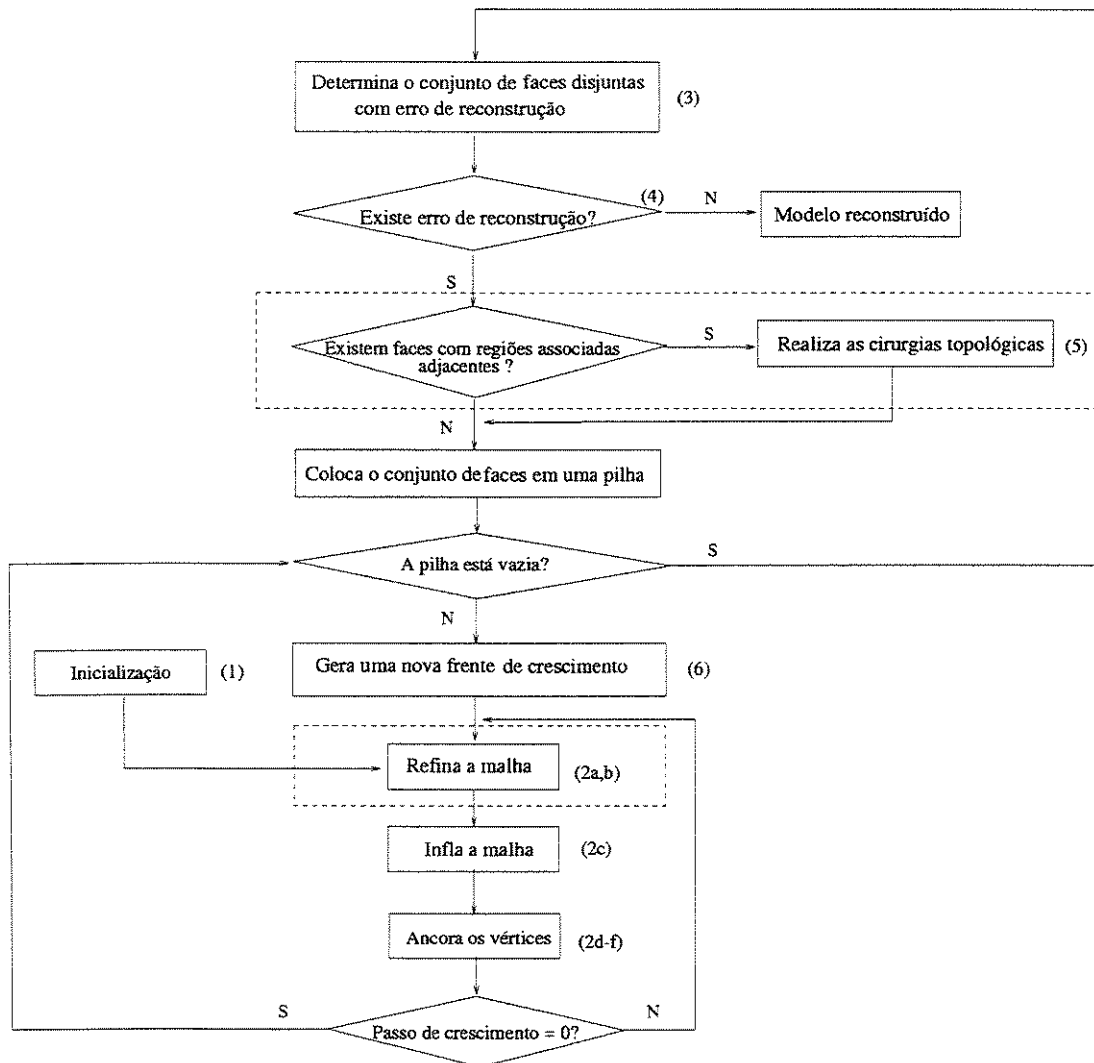
Figura 5.17: Fluxograma.
