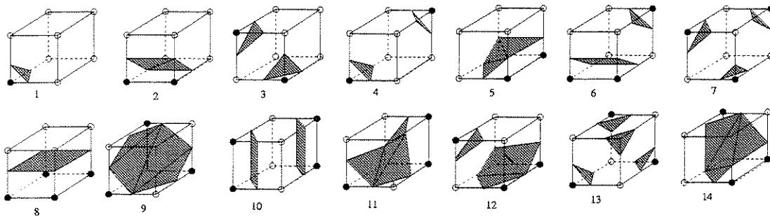
Figura 3.4: Tabela dos cubos com topologias distintas.
