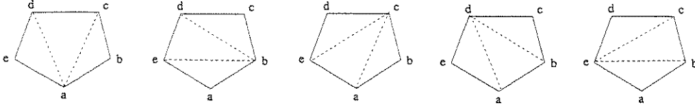
Figura 4.4: Configurações possíveis para trissecar uma face.
