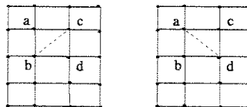
Figura 3.1: Possíveis conexões entre quatro pontos adjacentes.
