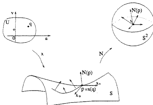
Figura 2.1: Aplicação de Gauss de S .
