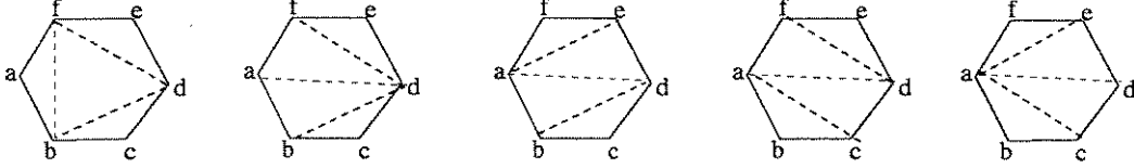
Figura 4.5: Tipos de configurações para tetrasecar uma face.
