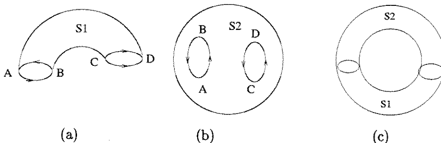
Figura 2.5: A costura de uma alça (a) e uma superfície esférica (b) resulta no toro (c).
