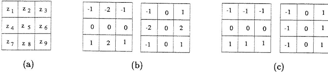
Figura 2.11: (a) Uma região da imagem, (b) máscaras de Sobel, (c) máscaras de Prewitt.
