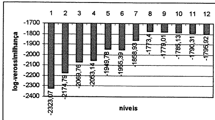
Figura 17: Variação de P(O|\lambda) com o número de níveis para uma locução de oito palavras. Verifica-se um comportamento não monotônico de crescimento e decaimento nos valores da log-verossimilhança com o número de níveis.
