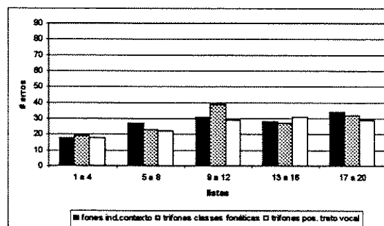
Figura 21: número de erros para cada subconjunto de frases nos testes com dependência de locutor.
