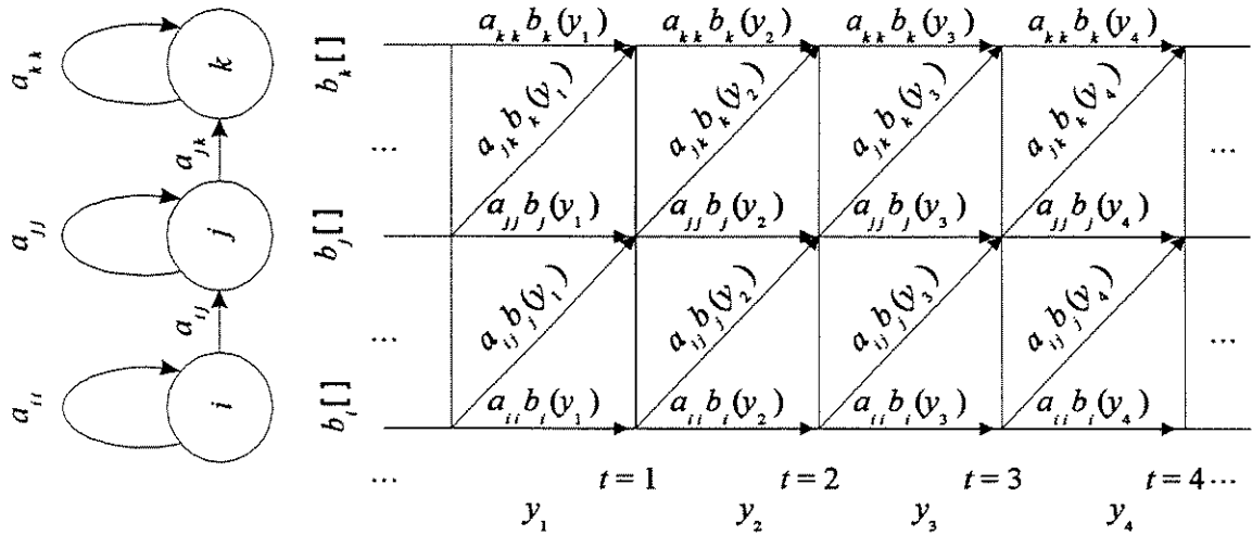
Figura 4: Exemplo de funcionamento do algoritmo de Viterbi.
