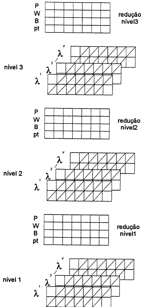
Figura 5: Exemplo de funcionamento do algoritmo Level Building .
