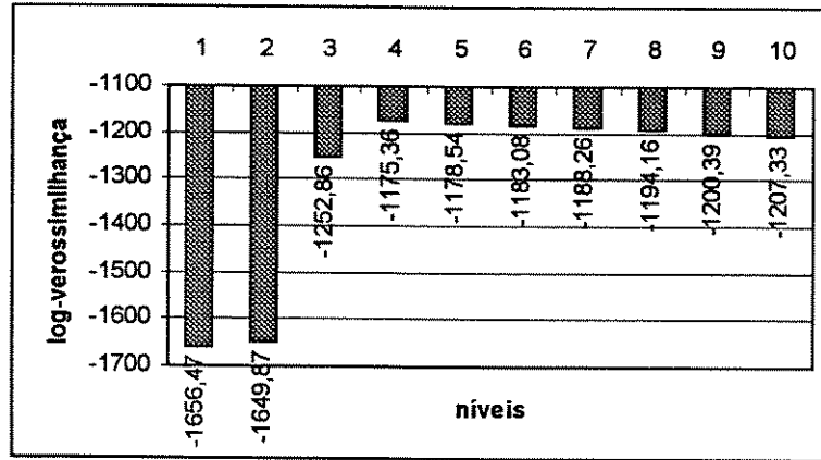
Figura 16: Variação de P(O|\lambda) com o número de níveis para uma locução de quatro palavras. Verifica-se um comportamento monotônico de crescimento e decaimento nos valores da log-verossimilhança com o número de níveis.
