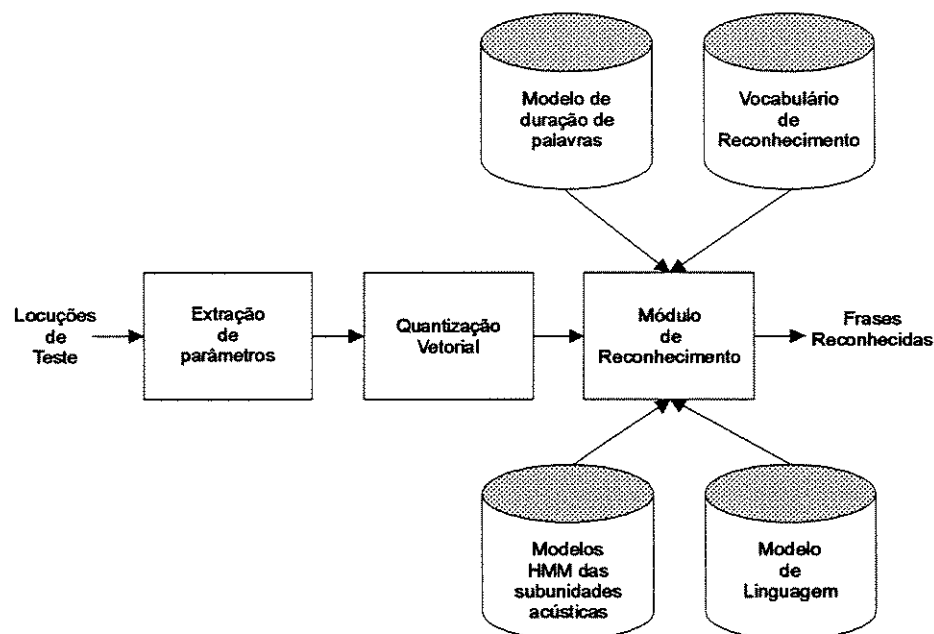
Figura 14: Diagrama de blocos do módulo de reconhecimento.
