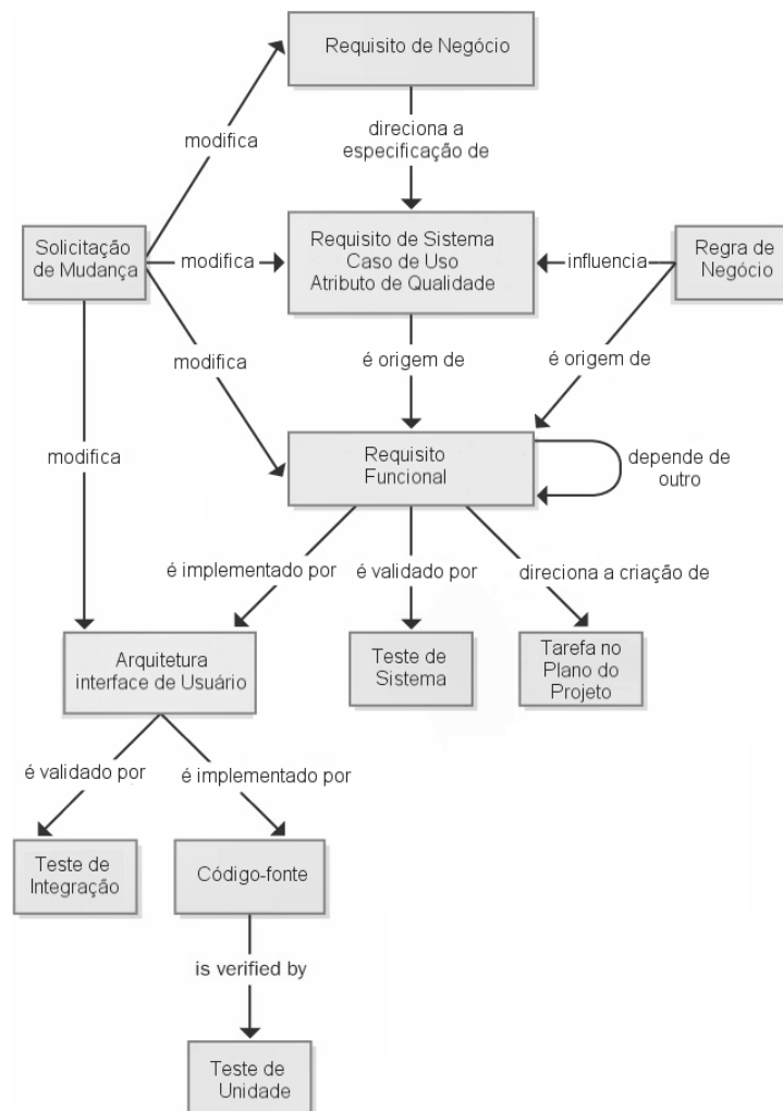
Figura 4.7: Exemplo de rastreabilidade em um projeto (Wiegers, 2003).
