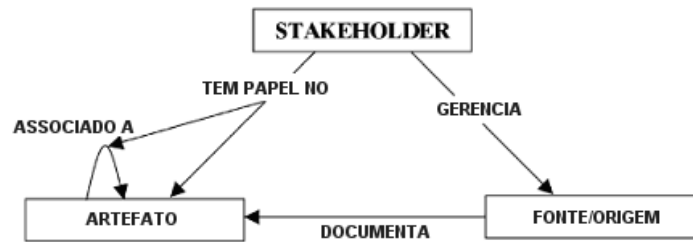
Figura 4.1: Meta-modelo de rastreabilidade (Ramesh e Jarke, 2001).
