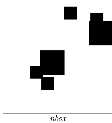
Figura 4.21: Imagem 256 \times 256 utilizada para teste de eficiência para os algoritmos da TDE, onde a cor preta é 0 e a cor branca é k \neq 0 .
