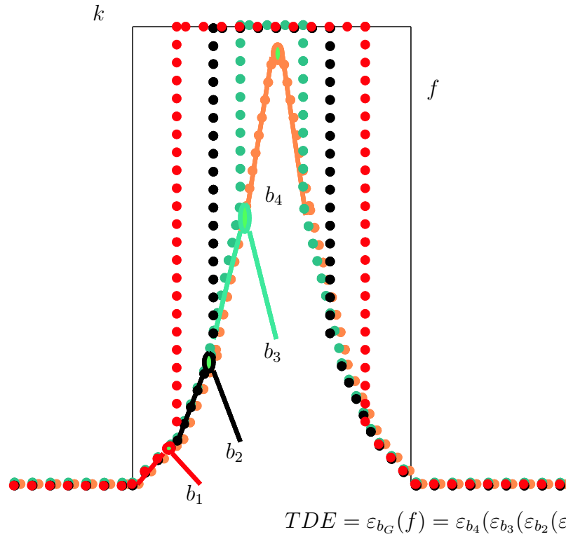
Figura 4.15: Ilustração da TDE 1D obtida de erosões por decomposição de função estruturante.
