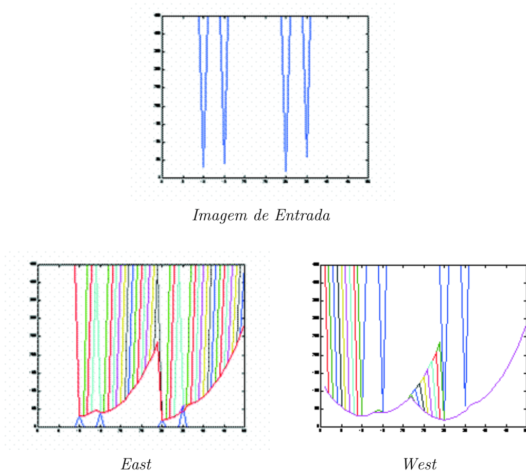
Figura 4.17: Ilustração do segundo passo do algoritmo multidimensional.
