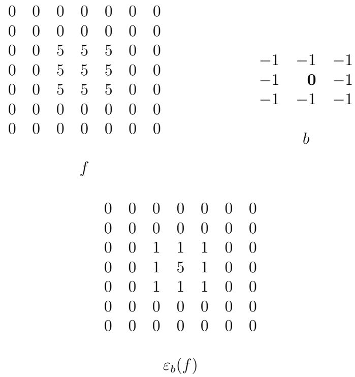
Figura 3.2: Ilustração da erosão paralela \varepsilon_b(f) da imagem de entrada f pela função estruturante b , com origem no centro.
