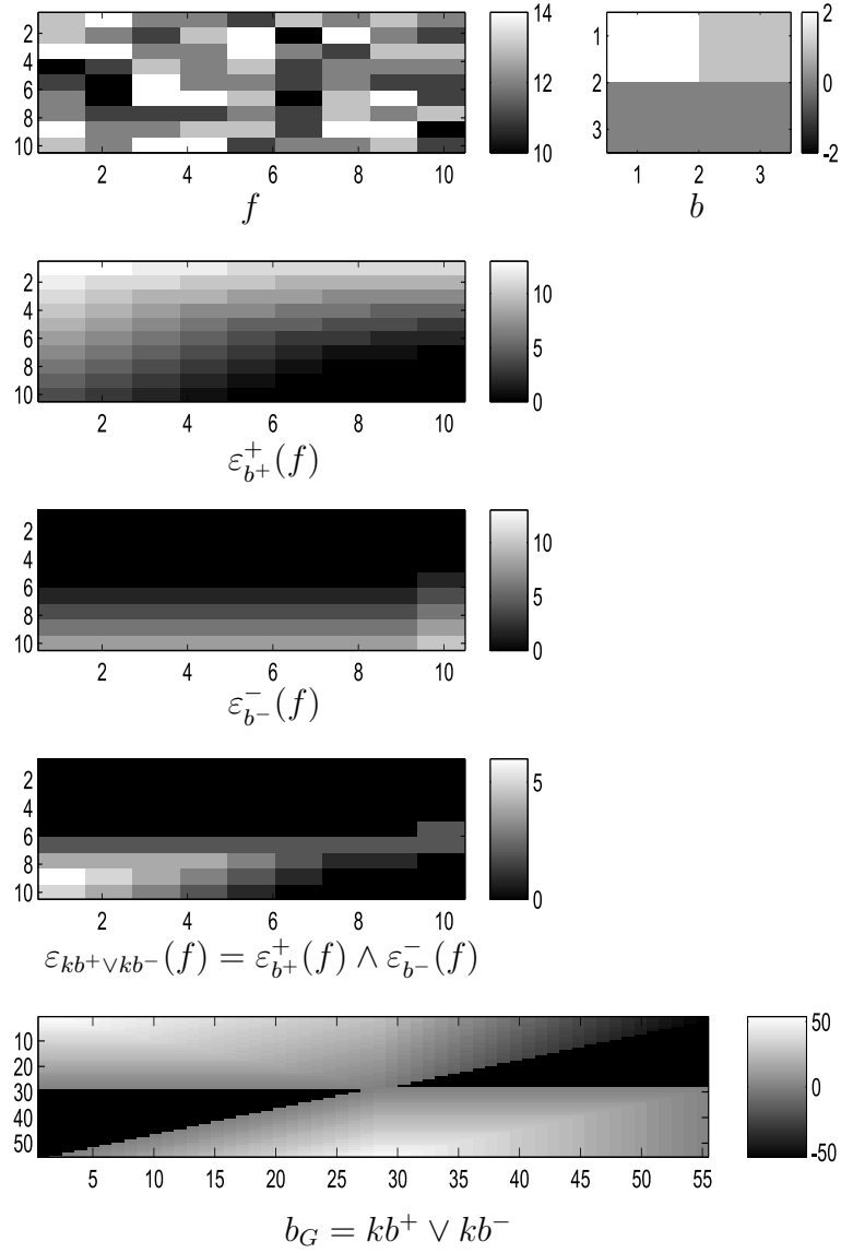
Figura 3.8: Ilustração da equivalência entre algoritmos paralelos e sequenciais para funções estruturantes bidimensionais.
