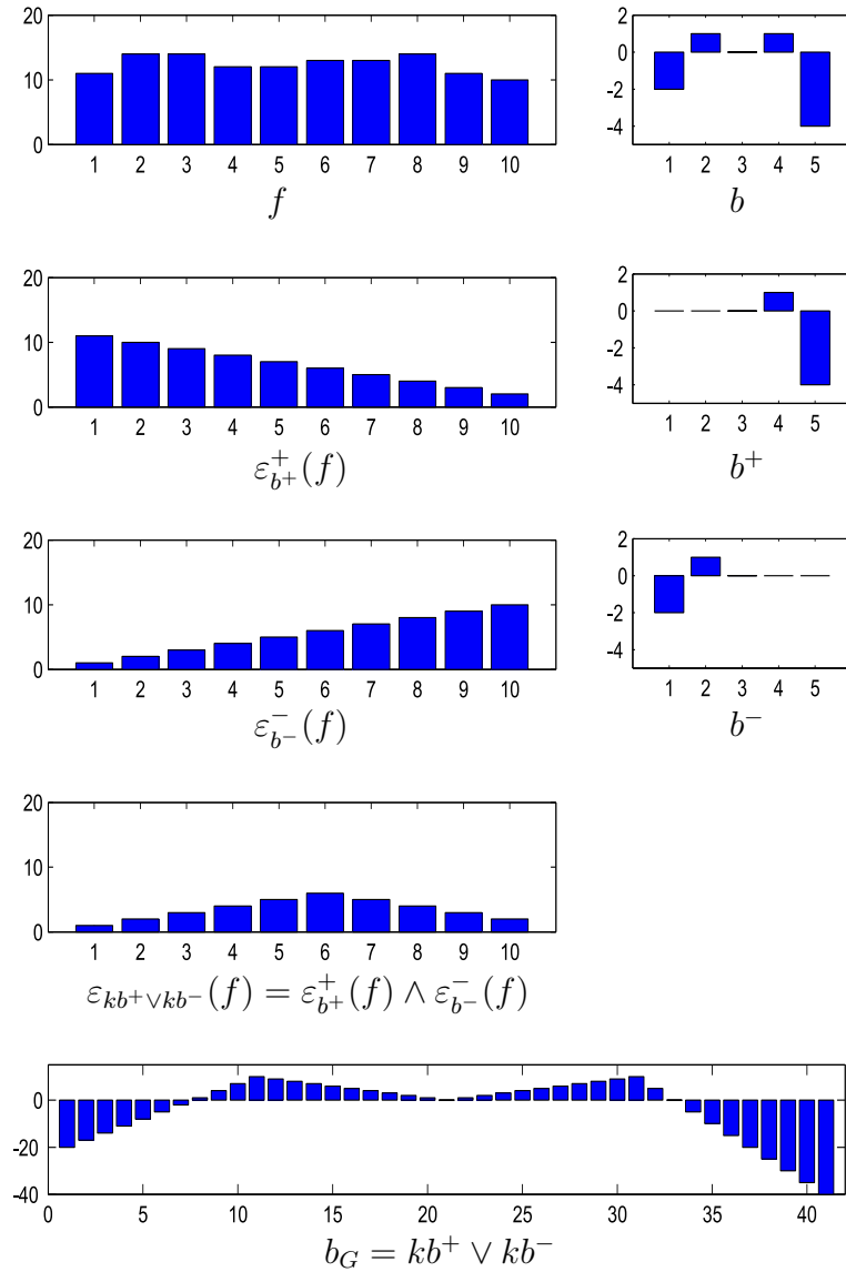
Figura 3.6: Ilustração da equivalência entre algoritmos paralelos e sequenciais para funções estruturantes unidimensionais.
