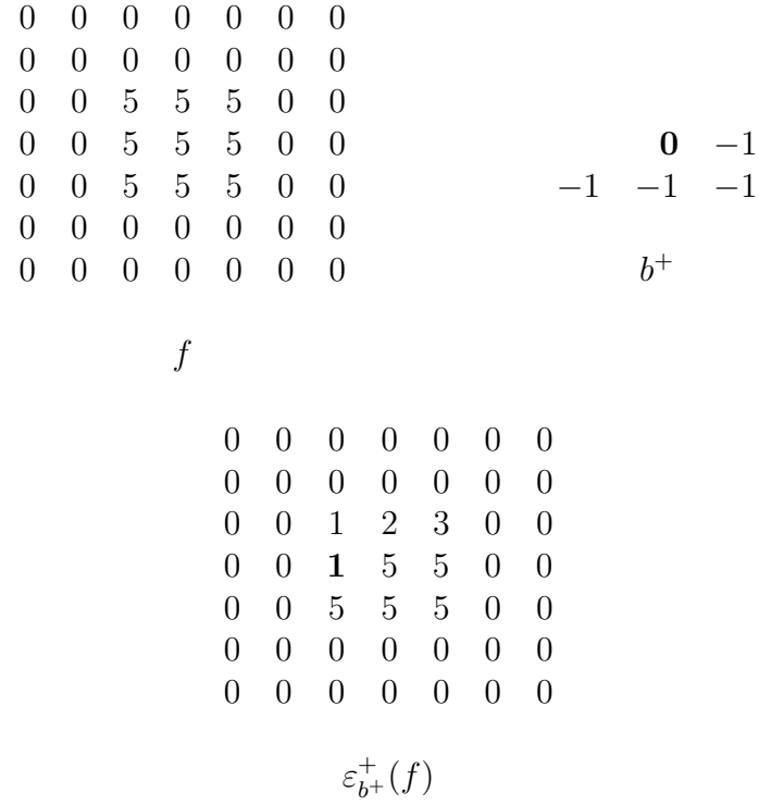
Figura 3.5: Ilustração de uma iteração intermediária da erosão seqüencial raster , \varepsilon_{b^+}^+(f)(x) , da imagem de entrada f pela função estruturante b^+ , com origem em negrito. O pixel x , que está em negrito com valor 1 , é o que está sendo processado.
