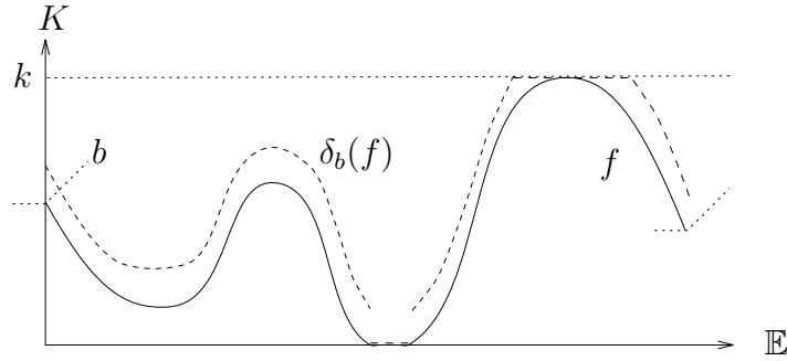
Figura 2.3: Dilatação de uma imagem em níveis de cinza f por uma função estruturante b .
