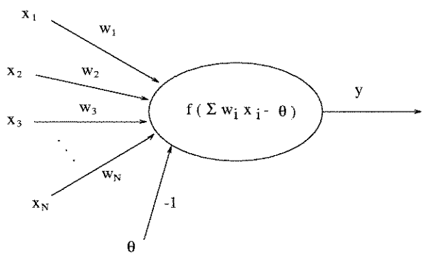
Figura 4.1: Ilustração de um neurônio ou nó.
