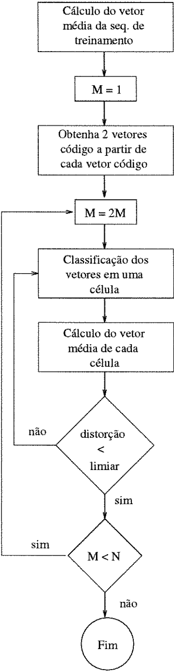
Figura 6.6: Procedimento do algoritmo LBG
