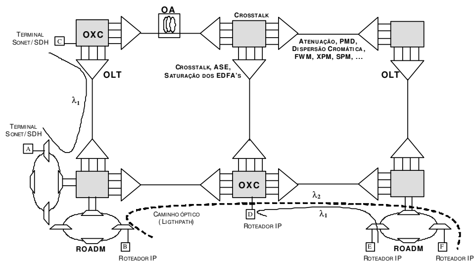
Figura 2.2: Arquitetura de Rede Óptica.
