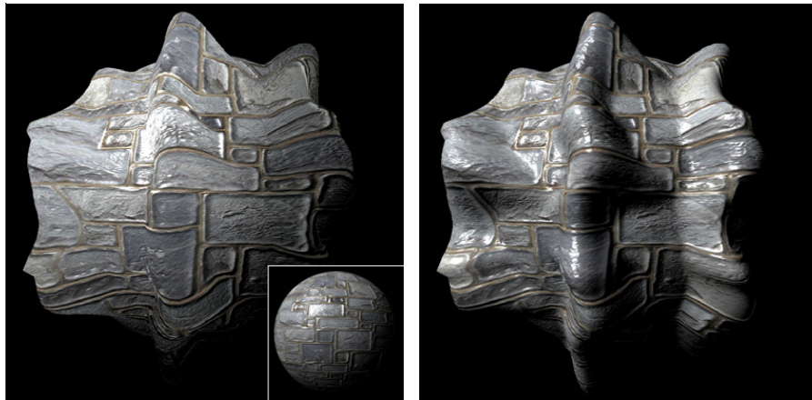
Fig. 4.1: Esfera deformada na GPU por ruído de Perlin, com normal mapping e sombreamento Phong. Esquerda: iluminação usando propriedades de geometria diferencial da esfera original (detalhe). Direita: iluminação usando propriedades de geometria diferencial calculadas na GPU após a deformação.
