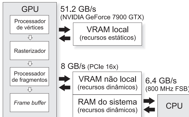
Fig. 1.1: Largura de banda da transferência de recursos armazenados na memória de vídeo e na memória do sistema.
