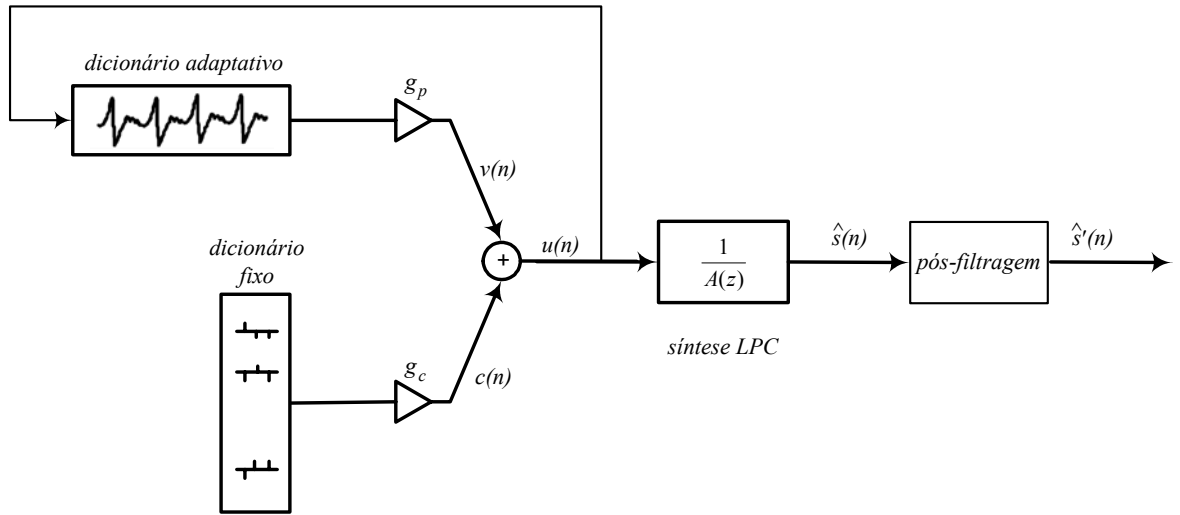
Figura 3-5: Diagrama de Blocos Simplificado do Modelo de Síntese CELP.
