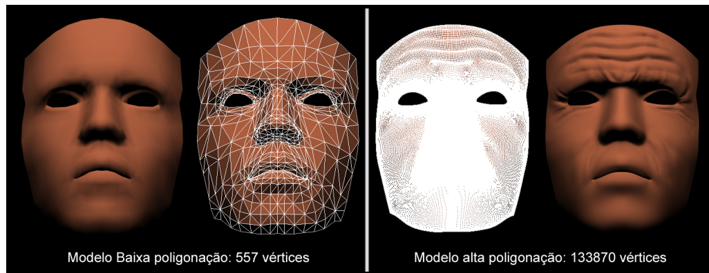
Fig. 4.16: Modelos geométricos utilizados para a geração dos mapas de normais. Modelos de baixa densidade de polígonos texturizado e aramado (esquerda) e modelos de alta densidade de polígonos com rugas aramado e texturizado (direita).
