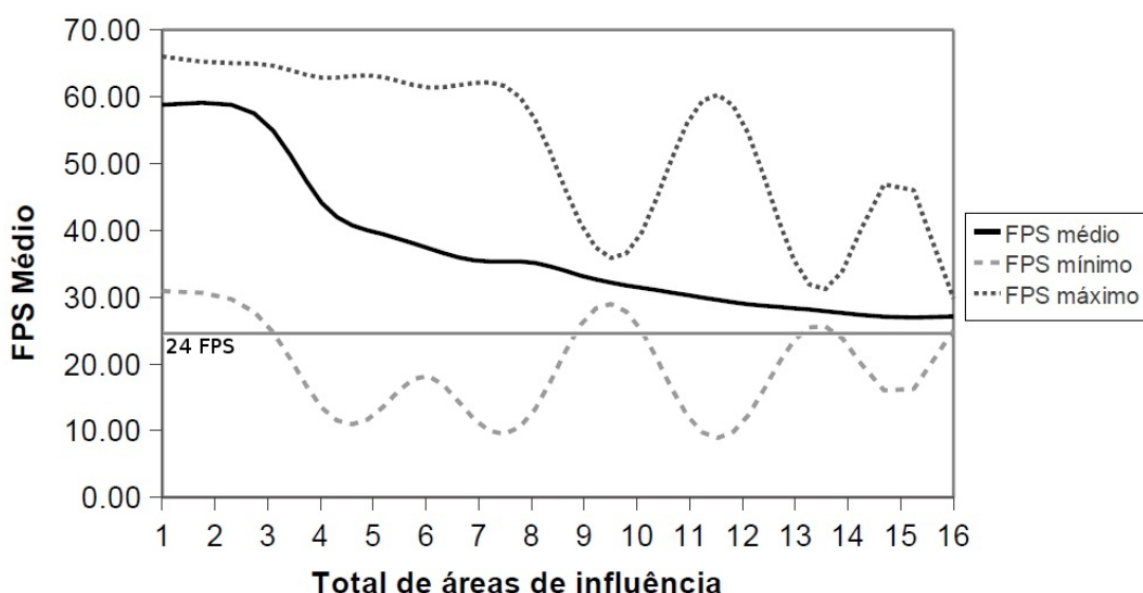
Fig. 5.3: Comparativo entre FPS médio pelo número de áreas de influência utilizadas, para a técnica da Seção 4.2, considerando as configurações propostas na Seção 5.1.
