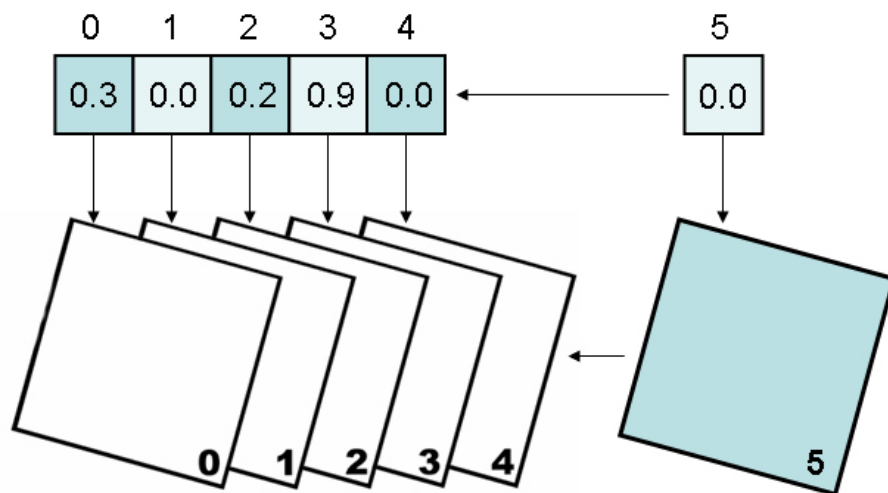
Fig. 4.4: Inclusão de uma área de influência e redimensionamento do Vetor de Ativação.
