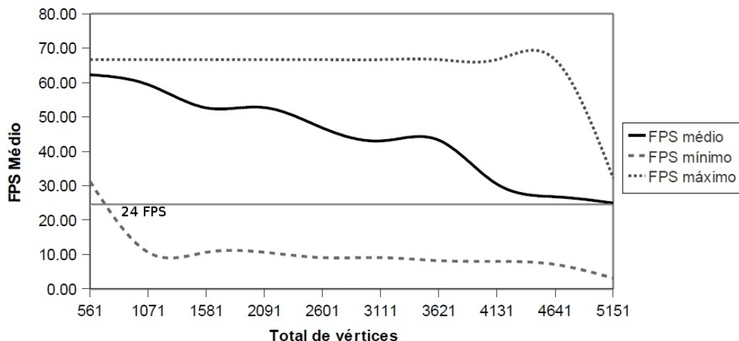
Fig. 5.4: Comparativo entre FPS médio pelo número de vértices nos modelos geométricos utilizados, para a técnica da Seção 4.3, trabalhando com as configurações propostas na Seção 5.1.
