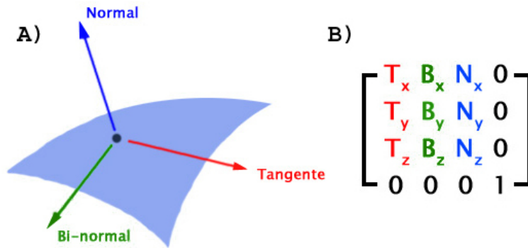
Fig. 3.10: Vetores normal, tangente e binormal no espaço tangente, criado a partir do raio de origem (Vetor normal do modelo de baixa densidade de polígonos), e matriz de rotação criada a partir desses vetores.
