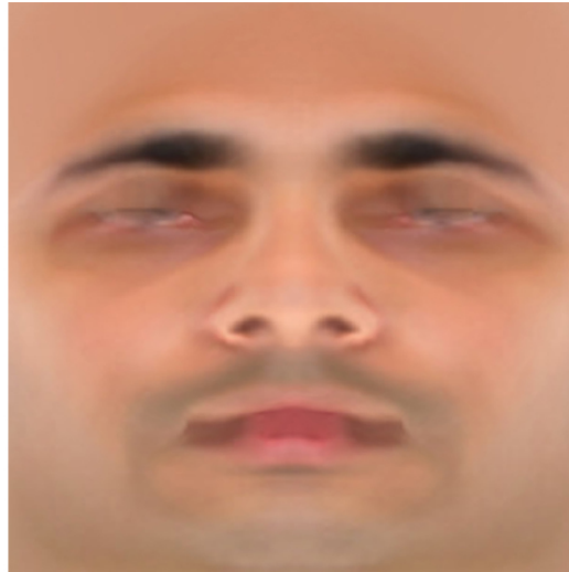
Fig. 4.15: Textura difusa.
