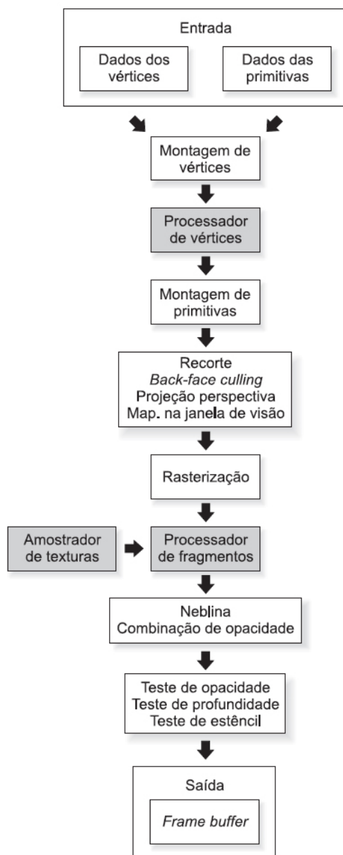
Fig. 3.1: Diagrama típico de um fluxo programável de síntese da imagem (Adaptado de Batagelo (2007)).
