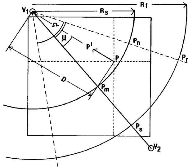
Fig. 2.4: Modelagem da região de influência do músculo virtual de Waters (Adaptado de Waters (1987)).
