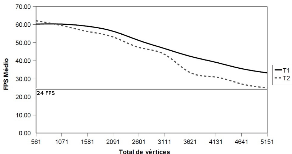
Fig. 5.5: Gráfico comparativo de performance entre as técnicas das Seções 4.2 (T1) e 4.3 (T2).
