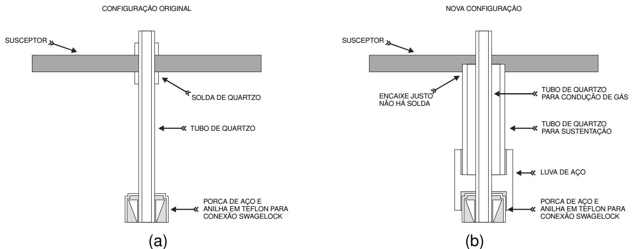
Figura 3.4: Detalhe mostrando a alteração efetuada na forma de sustentação do susceptor de grafite devido às constantes quebras no ponto de solda de quartzo.
