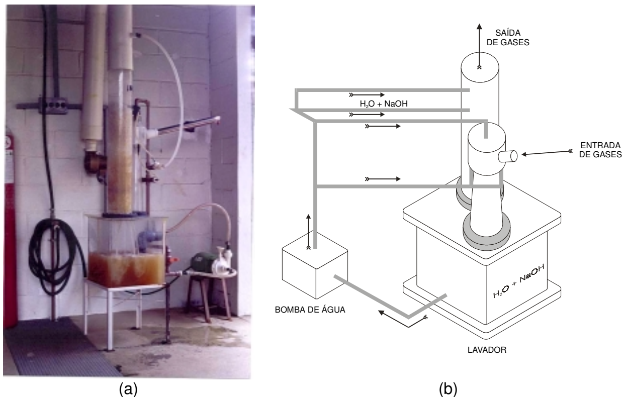
Figura 3.9: Lavador de gases do Reator Vertical. (a) lavador em funcionamento. (b) esquemático
