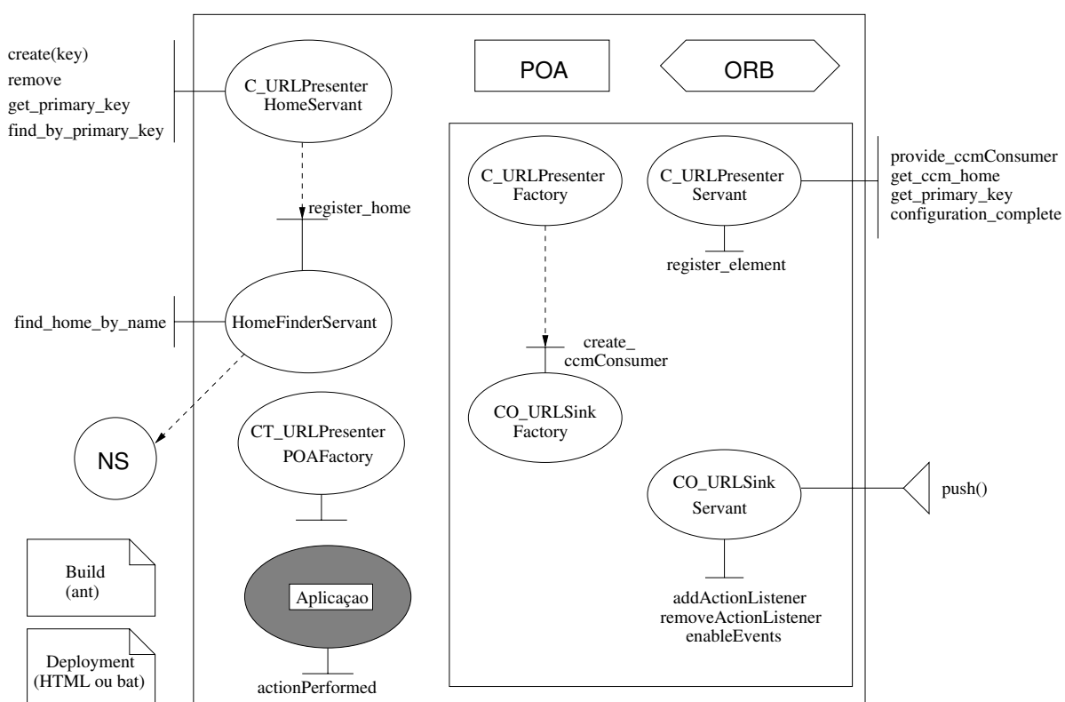
Figura 3.16: Container contendo um componente.
