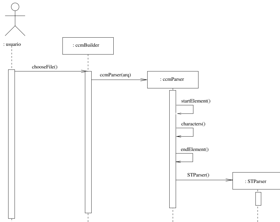
Figura 4.5: Diagrama de sequência do ccmBuilder.
