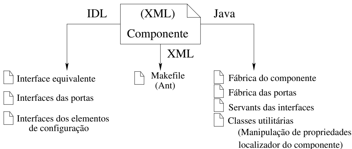
Figura 3.3: Arquivos gerados pelo ccmBuilder para um componente.
