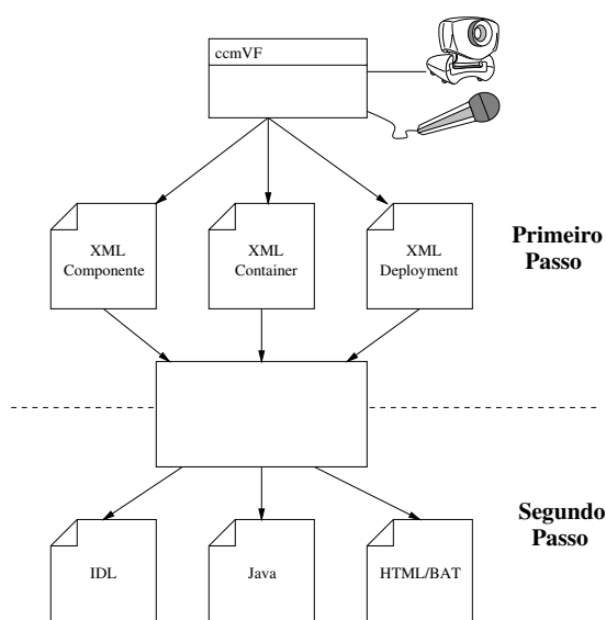
Figura 5.4: Passos para a construção do ccmVF.
